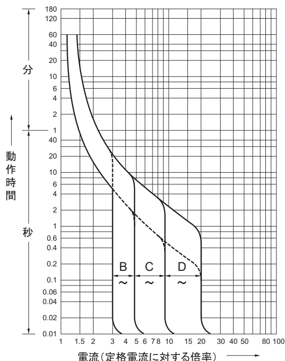
図 2-11 設備側分電盤のブレーカー特性
