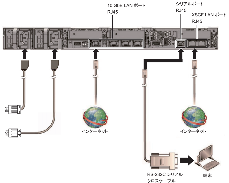
図 2-15 ネットワーク構成例
