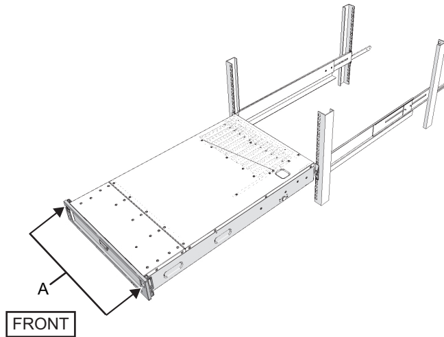
図 3-25 ラックへの搭載
