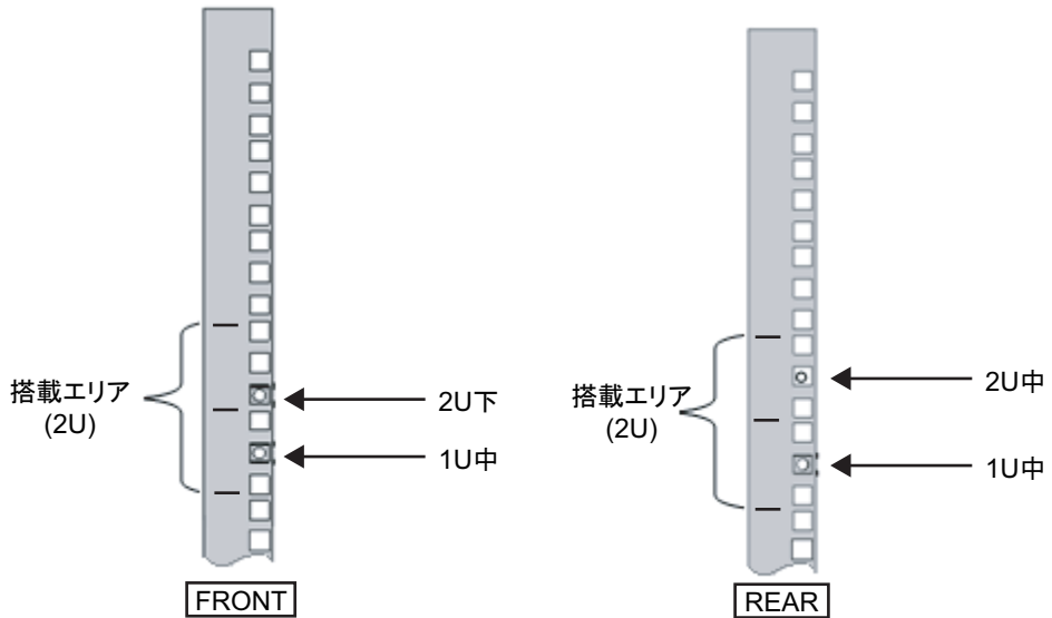
図 3-12 ラック支柱のケージナット取り付け位置
