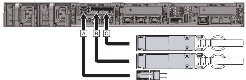
図 4-8 リンクケーブルとマネジメントケーブルの接続（SPARC M12-1側）
