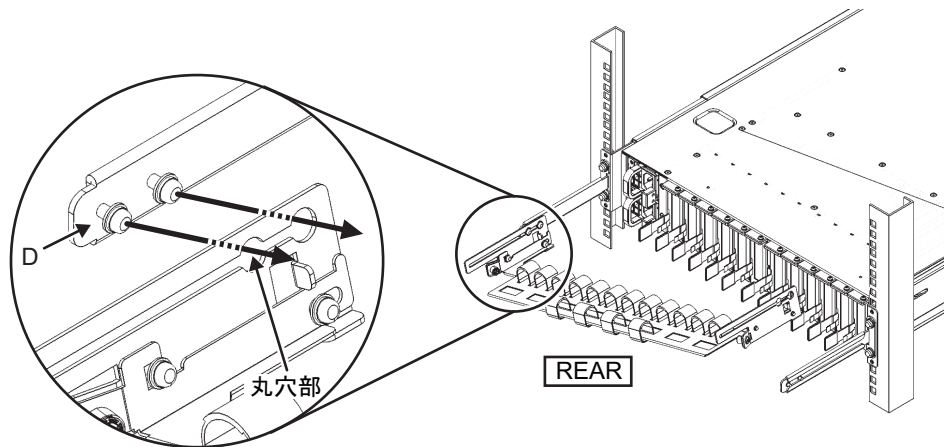
図 3-27 ケーブルサポートの取り付け（1）
