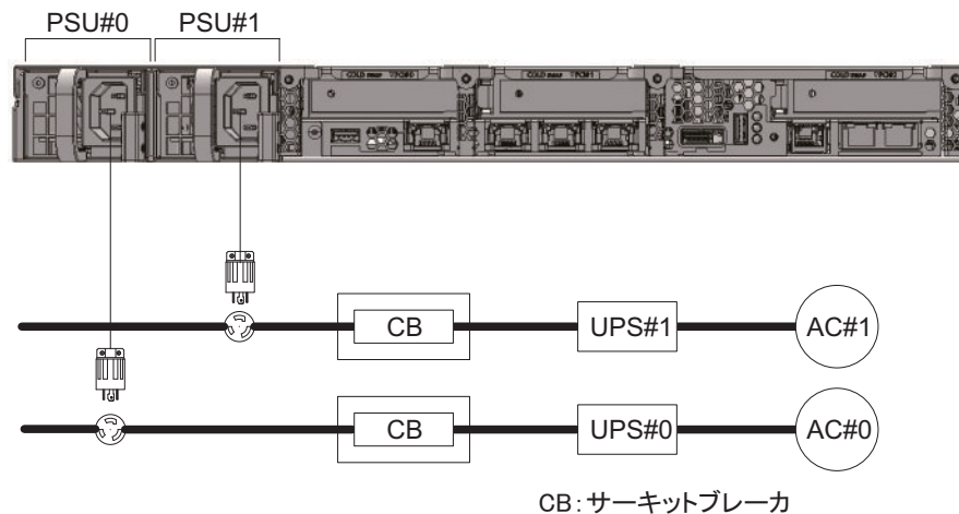
図 2-10 UPS接続時の電源系統図
