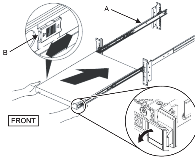
図 3-6 筐体をラックへ搭載
