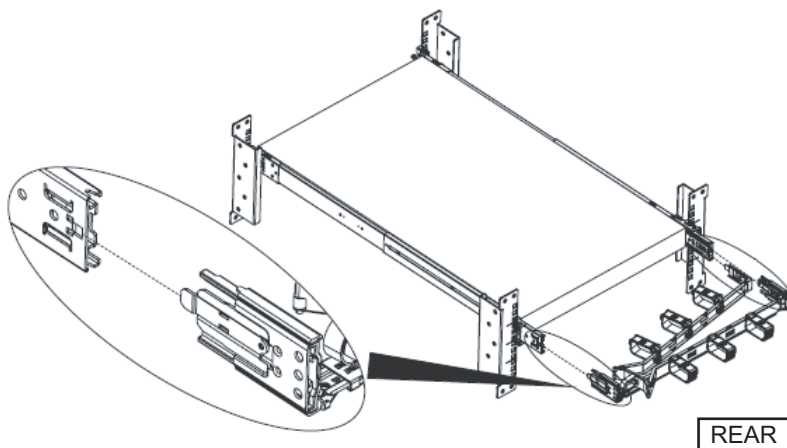
図 3-9 CMA 左側の取り付け
