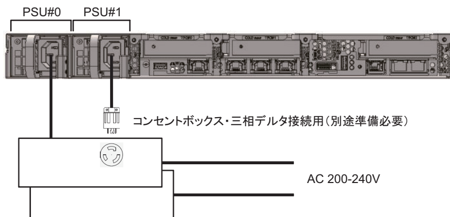
図 2-9 三相受電時の電源系統図（デルタ接続）
