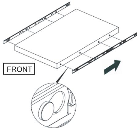
図 3-5 インナーレールの取り付け
