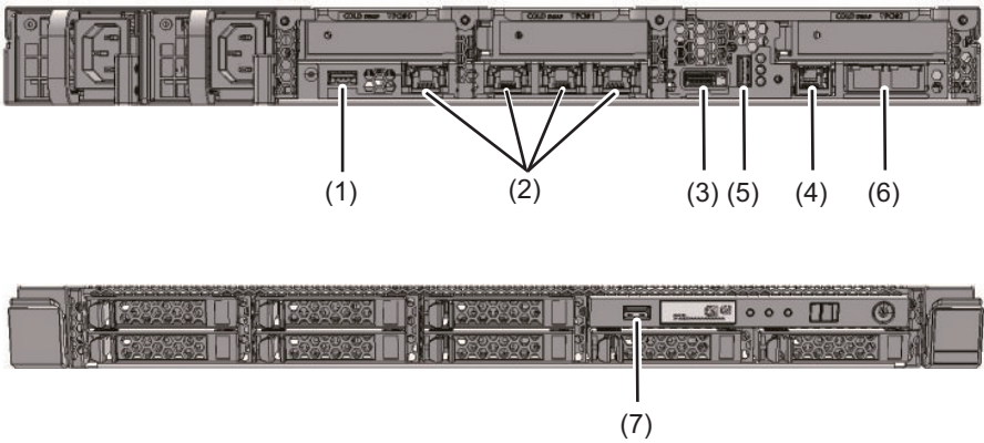
図 2-12 ネットワーク接続用ポートの位置
