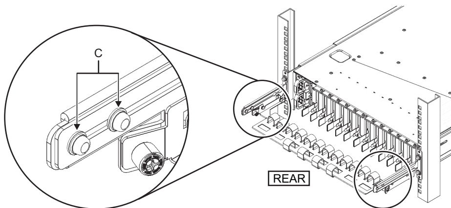
図 3-28 ケーブルサポートの取り付け (2)
