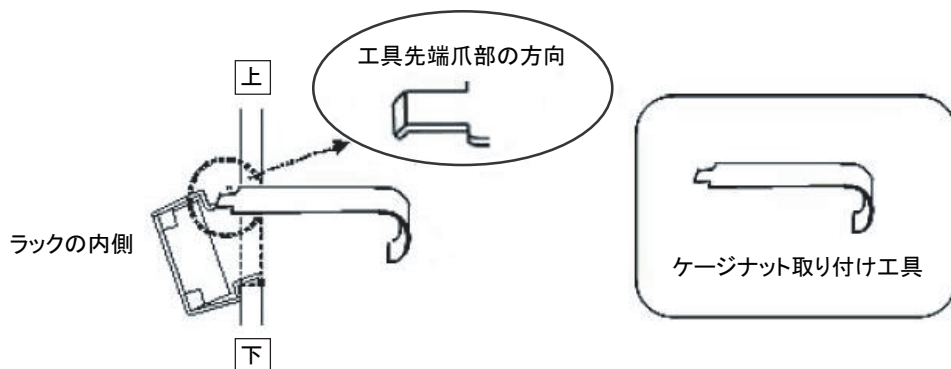
図 3-14 ケージナット取り付け工具の使用
