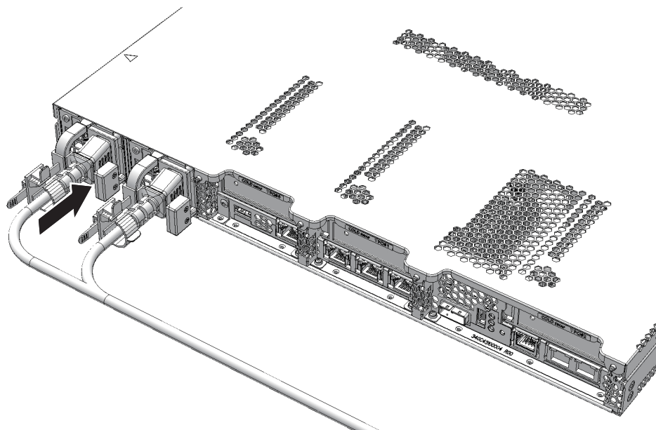
図 4-4 電源コードの取り付け
