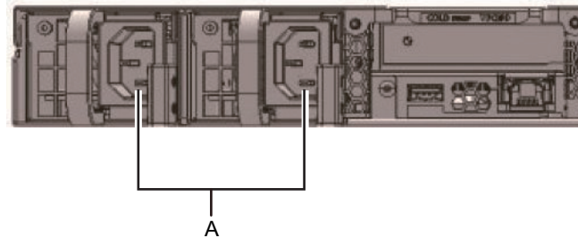
図 4-3 電源ユニットの位置
