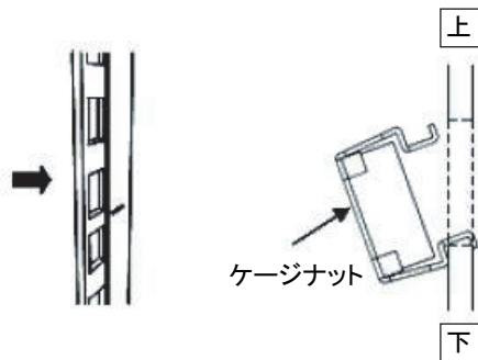
図 3-13 ケージナットのつめの向き
