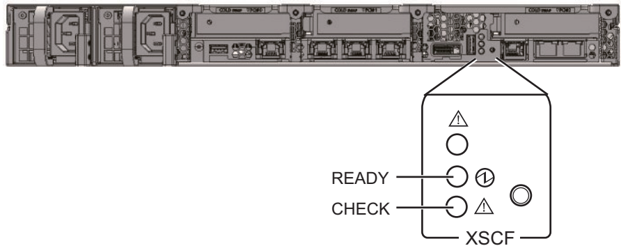
図 5-2 SPARC M12-1背面側
