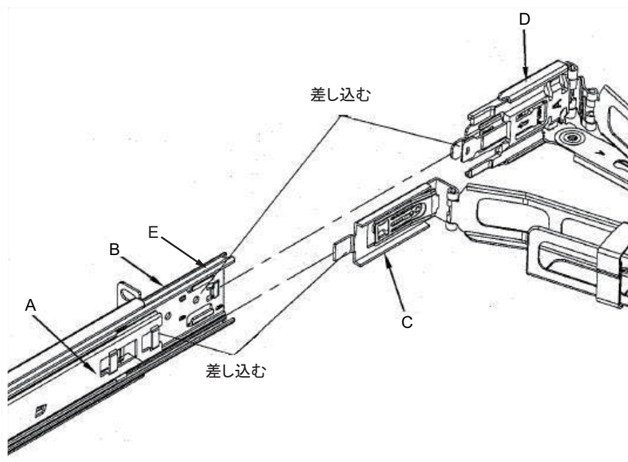
図 3-8 CMA 右側の取り付け
