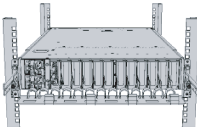
図 3-30 ケーブルサポートの取り付け完成図
