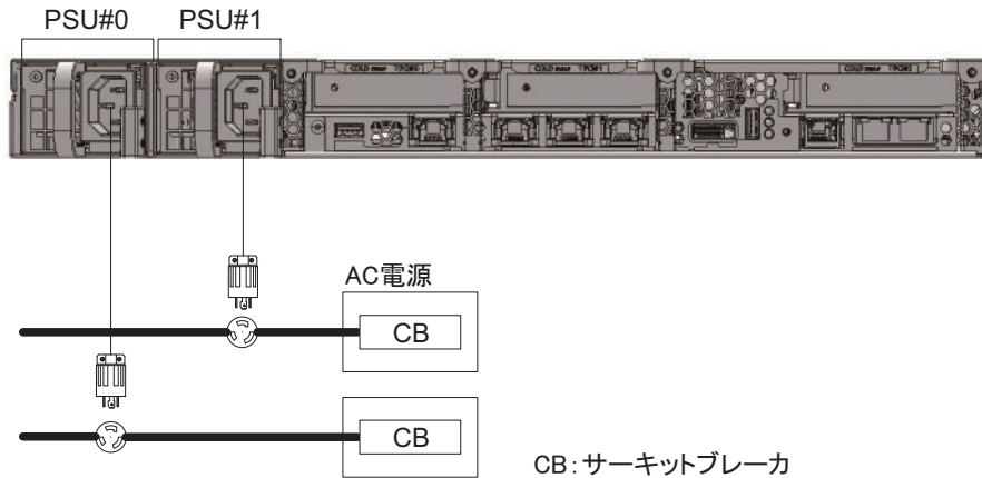
図 2-7 二系統受電時の電源系統図
