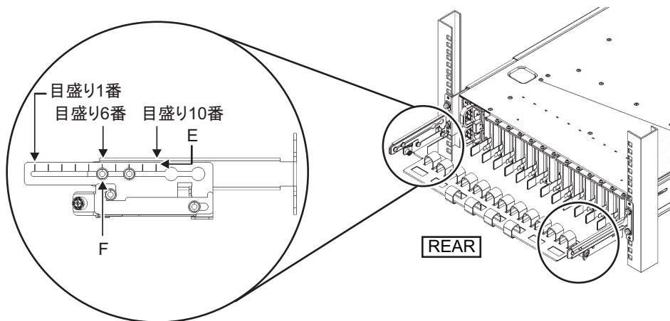
図 3-29 ケーブルサポートの取り付け (3)
