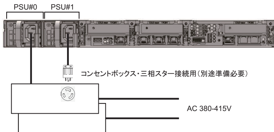
図 2-8 三相受電時の電源系統図（スター接続）
