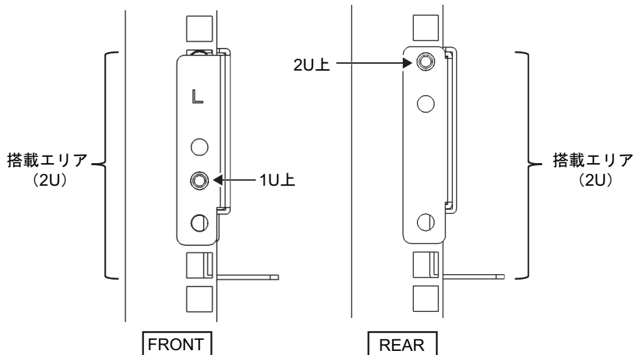
図 3-18 レールの取り付け：突起部の位置
