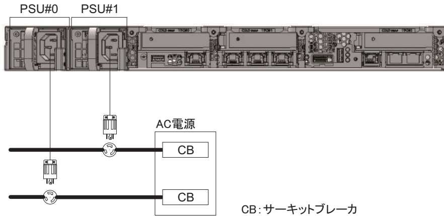
図 2-6 電源冗長接続時の電源系統図
