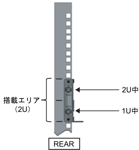
図 3-23 ケーブルサポート固定金具とレールの固定
