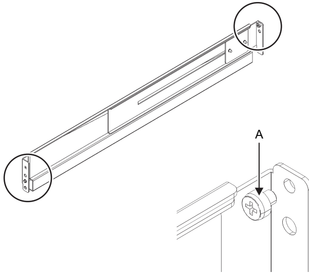
図 3-16 レールのピンの取り外し
