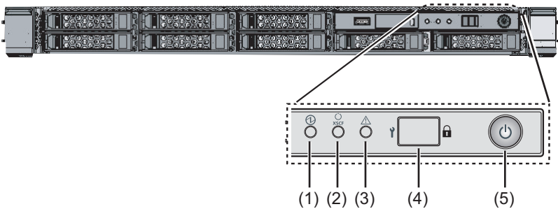
図 2-16 SPARC M12-1のオペレーションパネル
