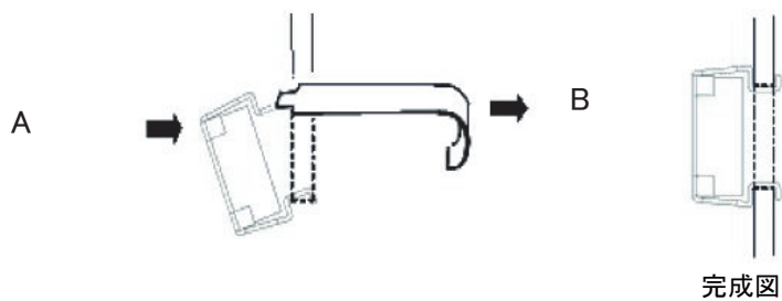
図 3-15 ケージナットの取り付け
