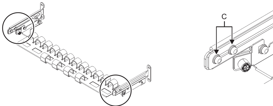
図 3-20 ケーブルサポート固定金具の取り外し（1）
