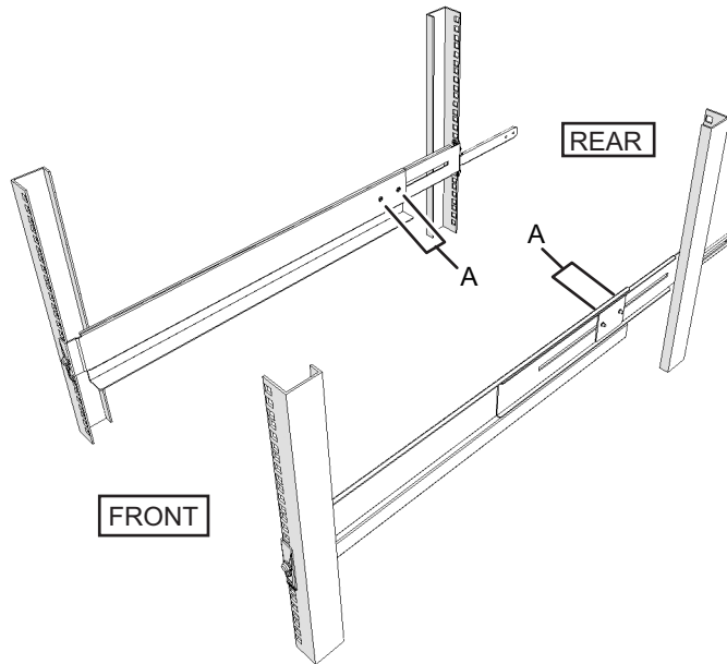
図 3-24 レール側面のねじ固定
