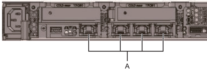
図 4-2 10 GbEポートの位置
