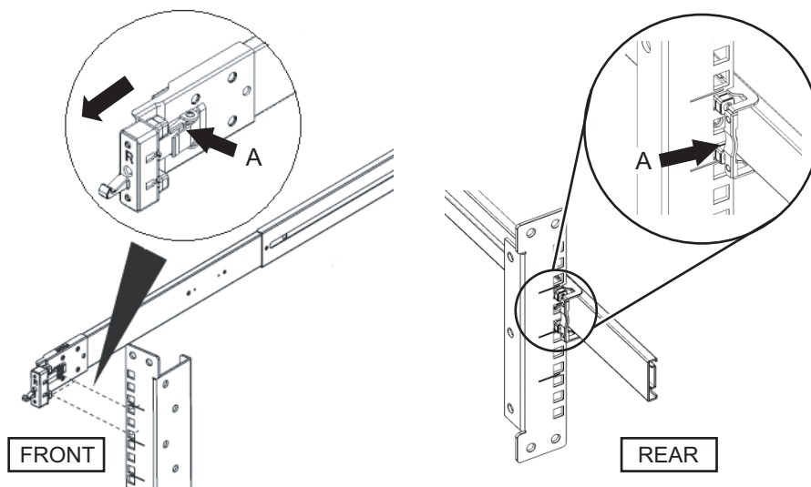
図 3-4 スライドレールの取り外し
