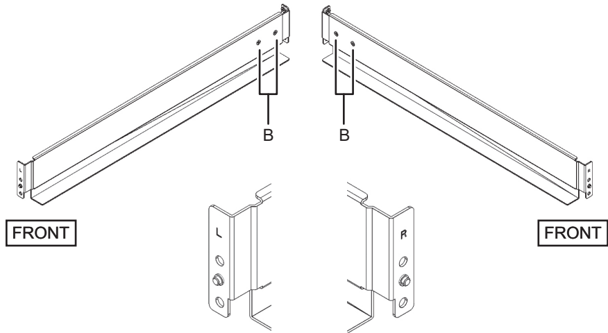
図 3-17 レールの側面のねじ
