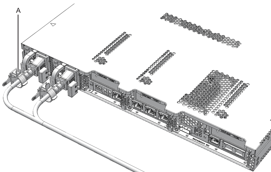
図 4-5 ケーブルクランプのロック
