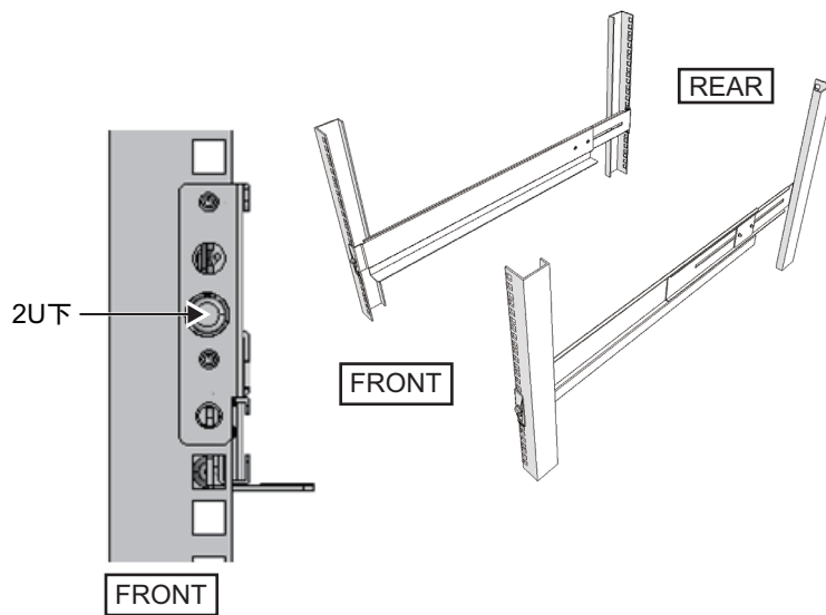
図 3-19 レールの取り付け：ねじの固定位置
