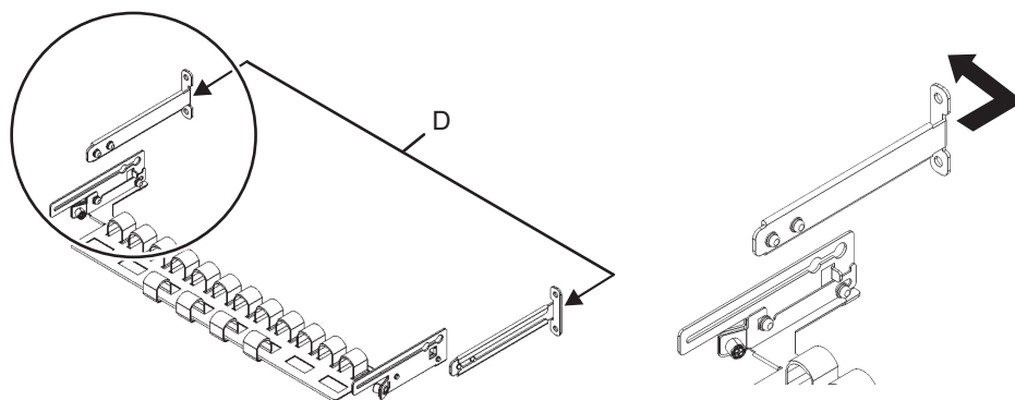
図 3-21 ケーブルサポート固定金具の取り外し (2)
