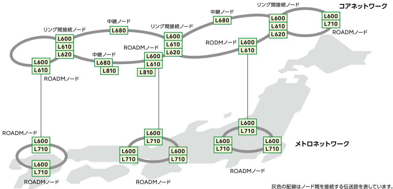
灰色の配線はノード間を接続する伝送路を表しています。
