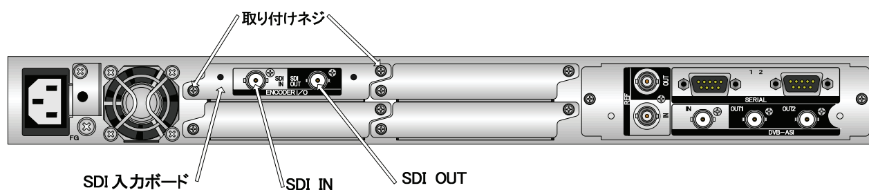
I P - 9 6 1 0 装置背面図
