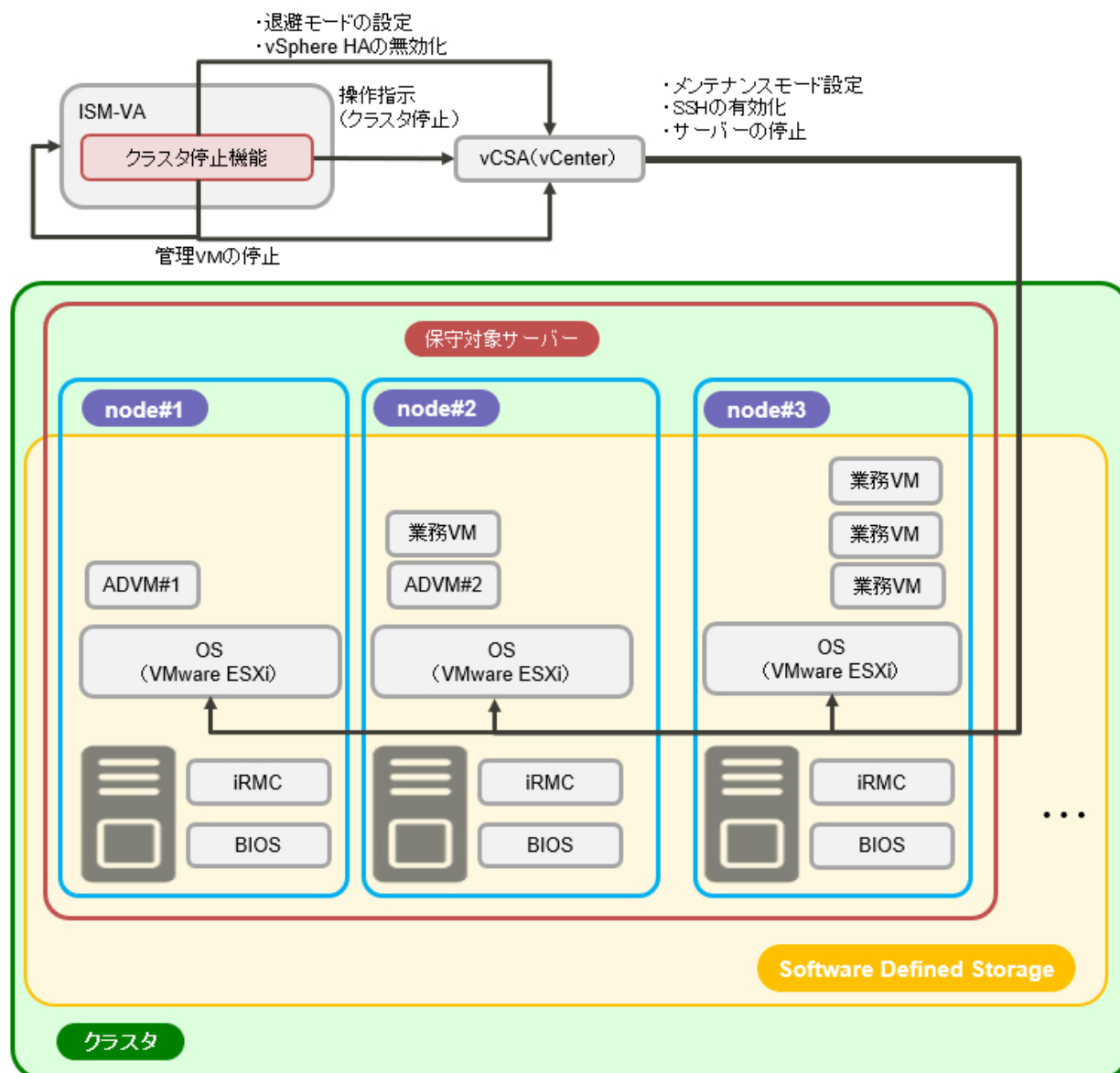
図2.35 クラスタ停止の動作概要
