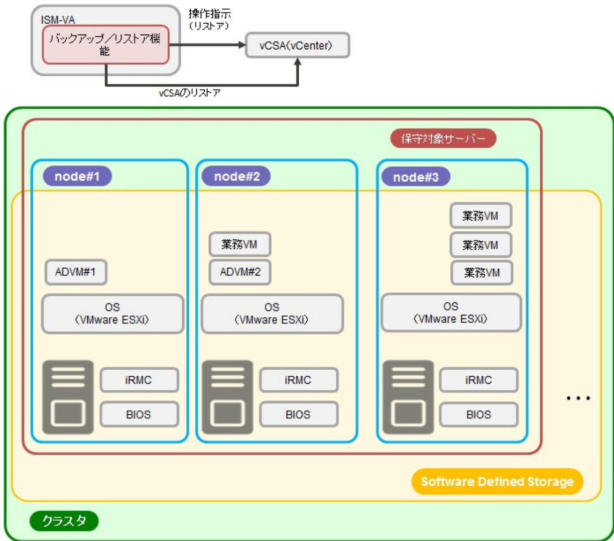
図2.34 リストア機能の動作概要
