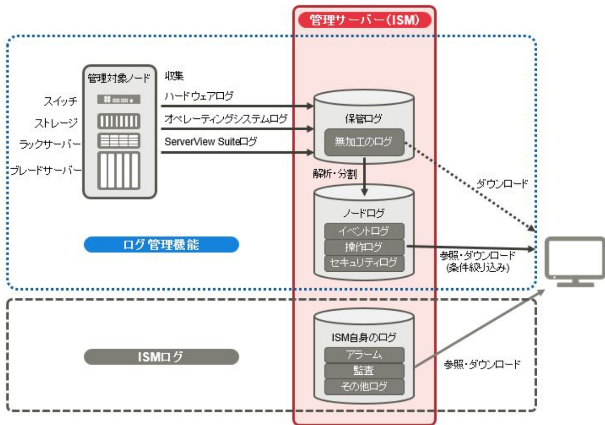
図2.12 ログ管理機能のイメージ
