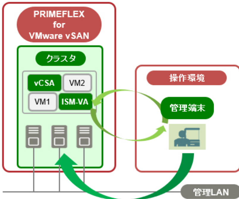
図2.37 ISM-VAとvCSAをクラスタに配置した構成での動作
