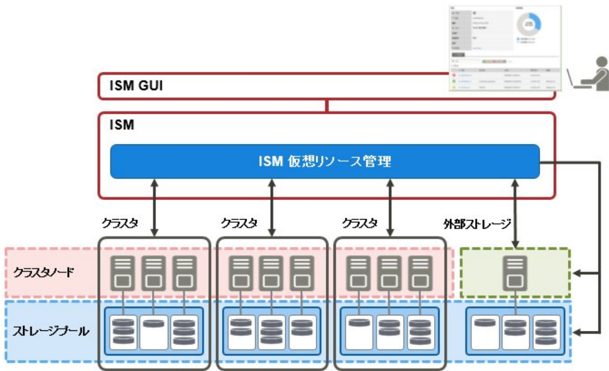
図2.17 仮想リソース管理機能の動作環境の構成
