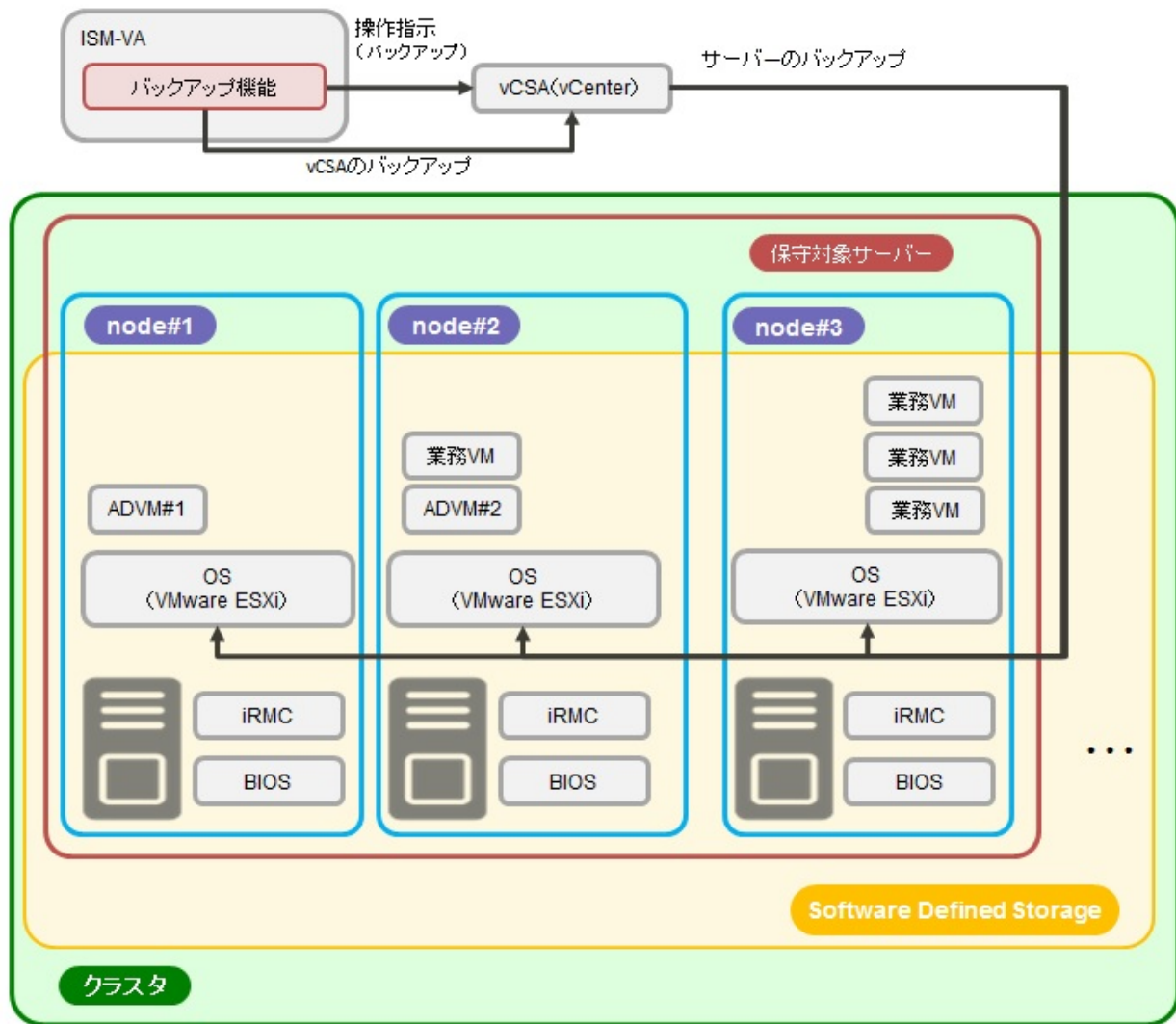
図2.33 バックアップ機能の動作概要
