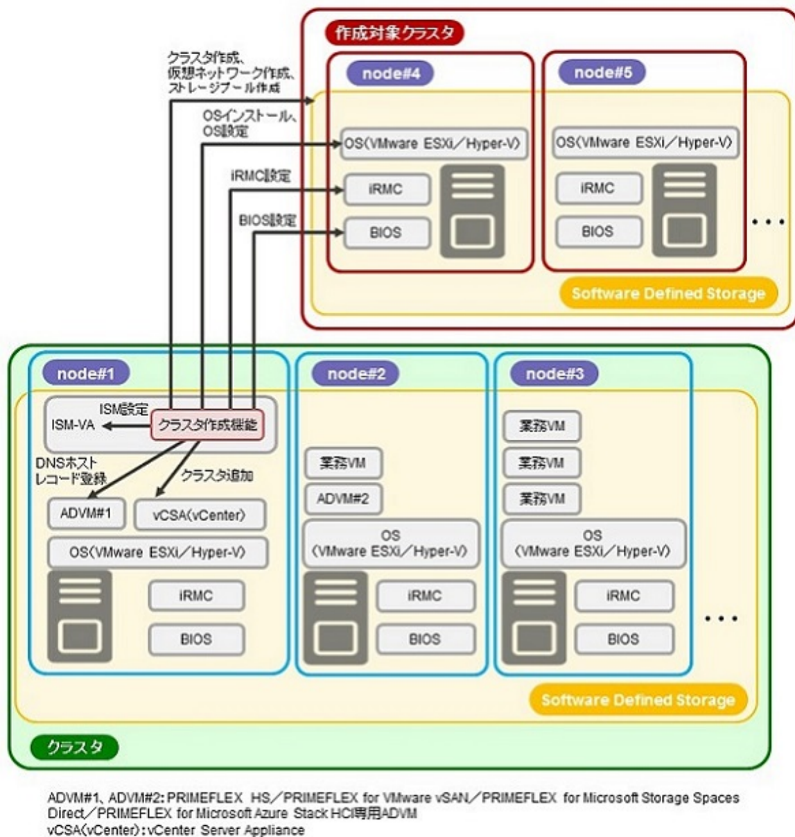
図2.26 クラスタ作成機能の動作概要
