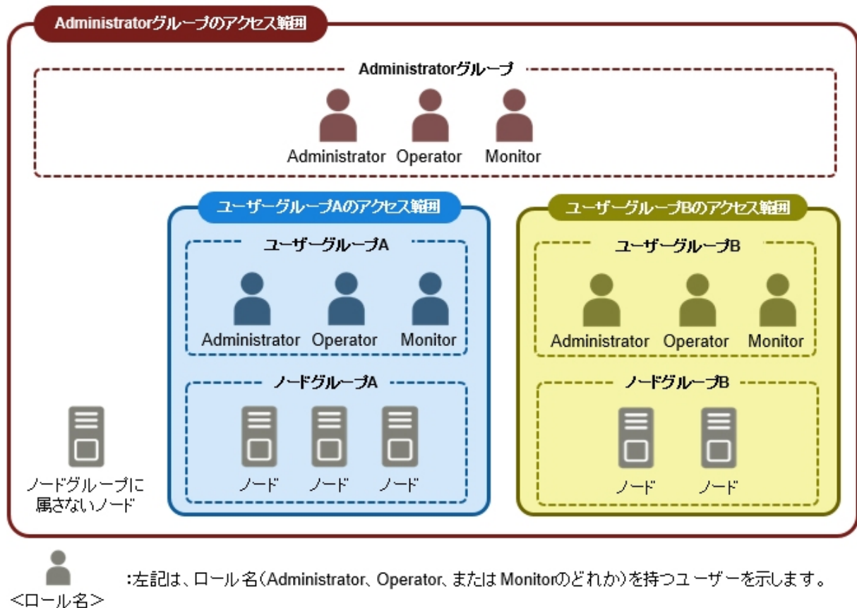
図2.38 ユーザーグループ、ノードグループ、ロールの関係
