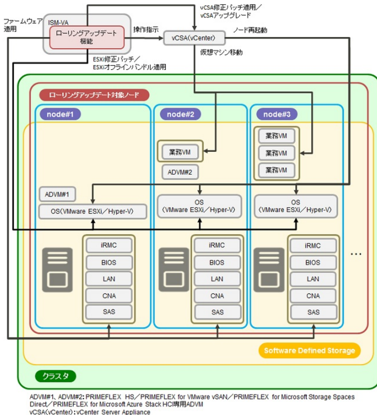
図2.30 ローリングアップデート機能の動作概要
