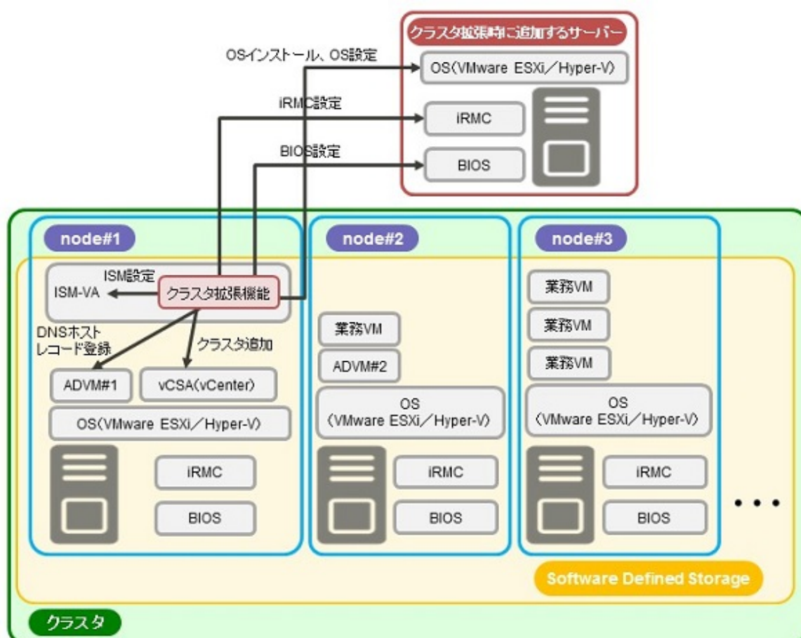
図2.28 クラスタ拡張機能の動作概要
