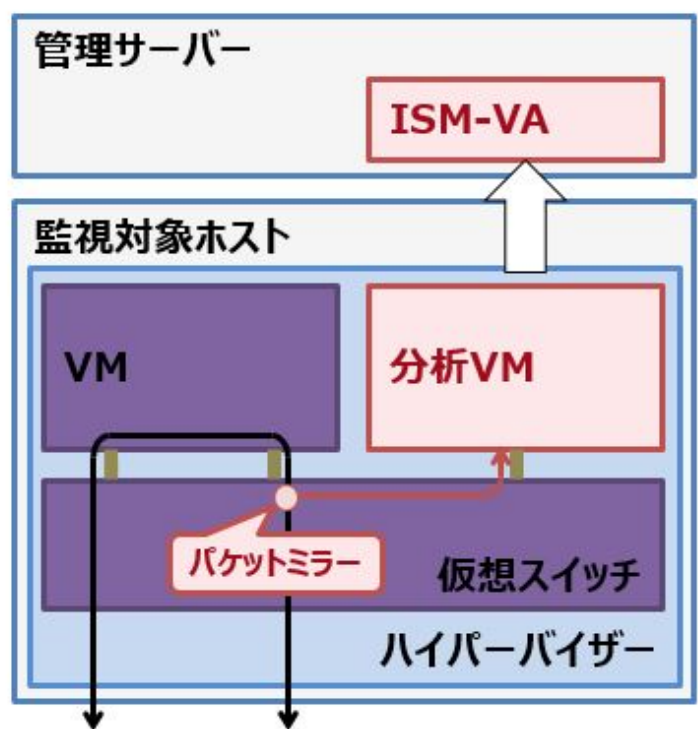
図2.20 仮想ネットワーク パケット分析の動作イメージ
