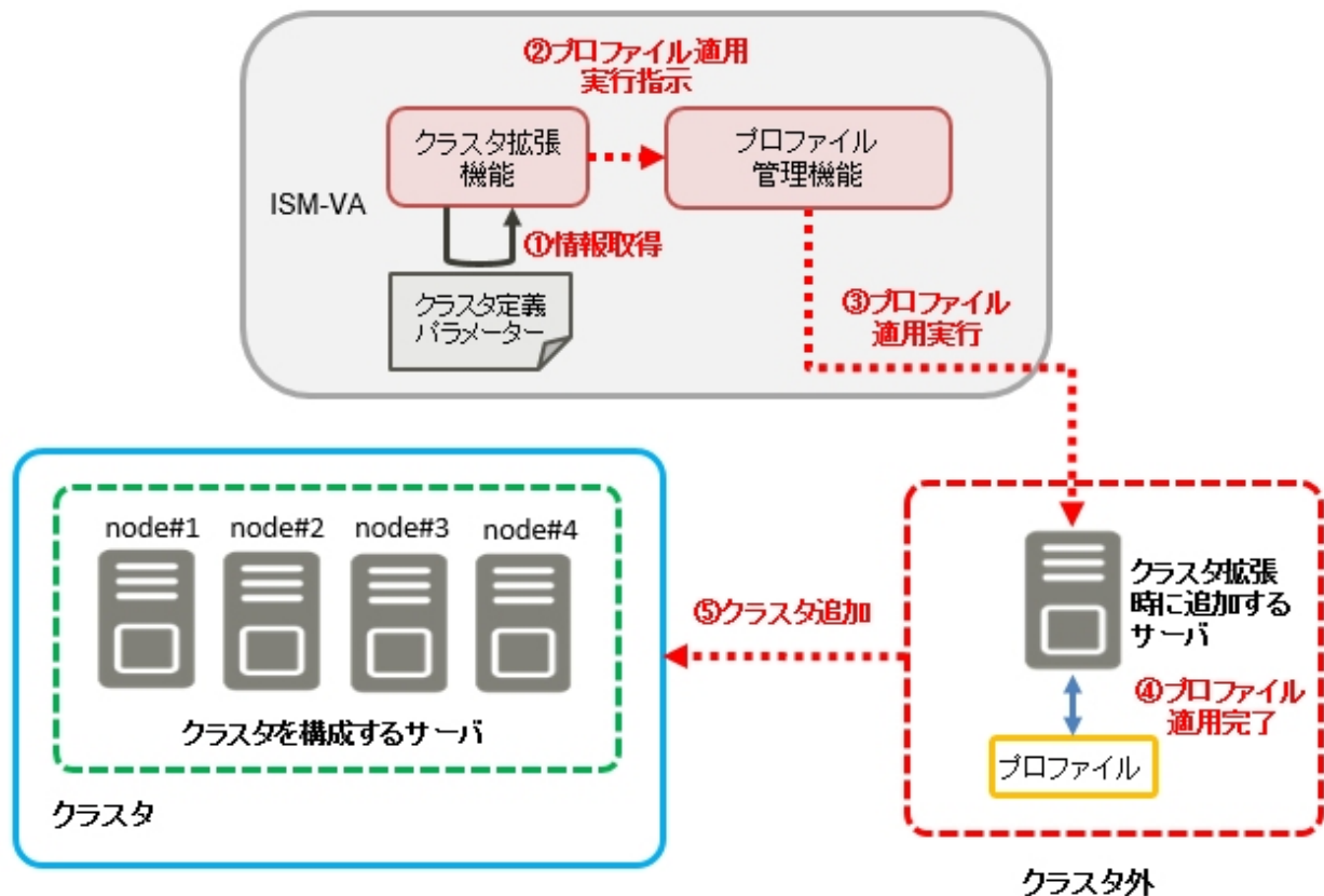
図2.23 クラスタ拡張機能とプロファイル管理機能の連携
