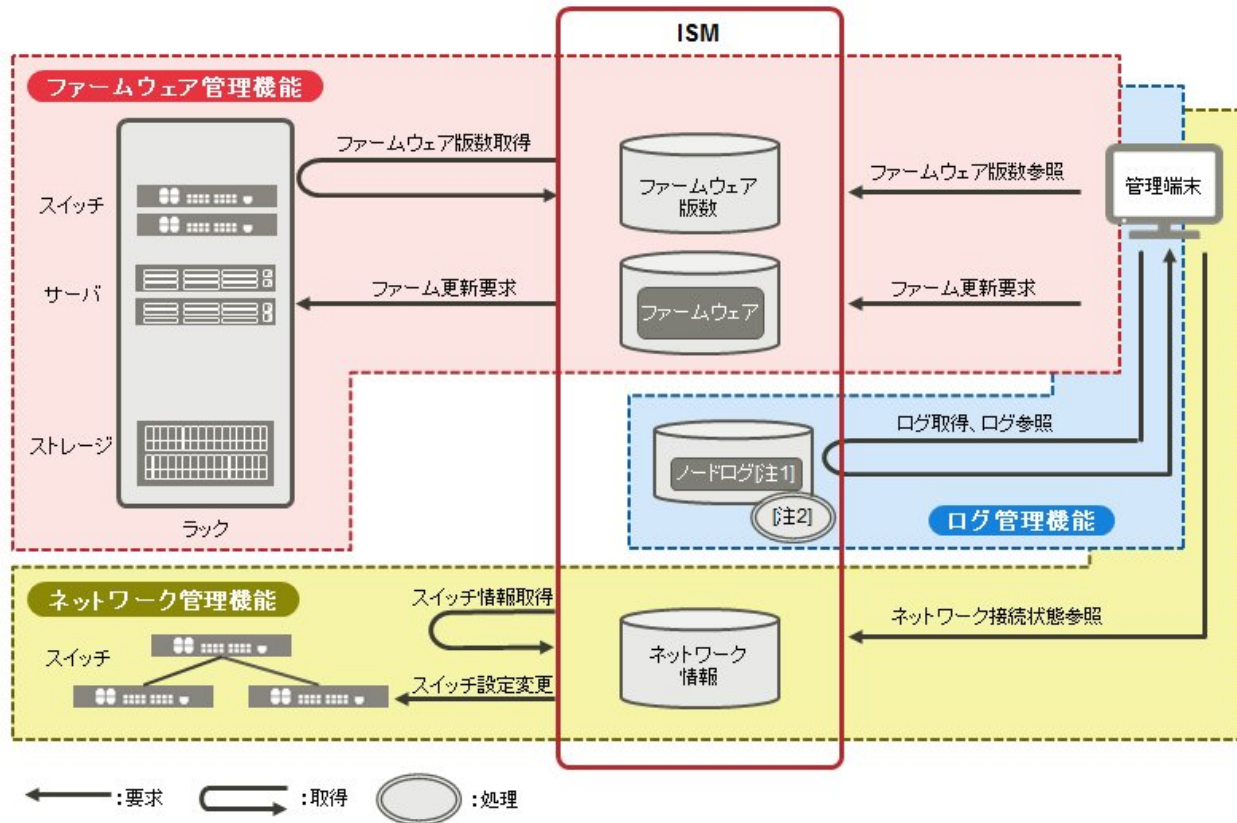
図1.7 機能イメージ(管理対象ノードの保守)
