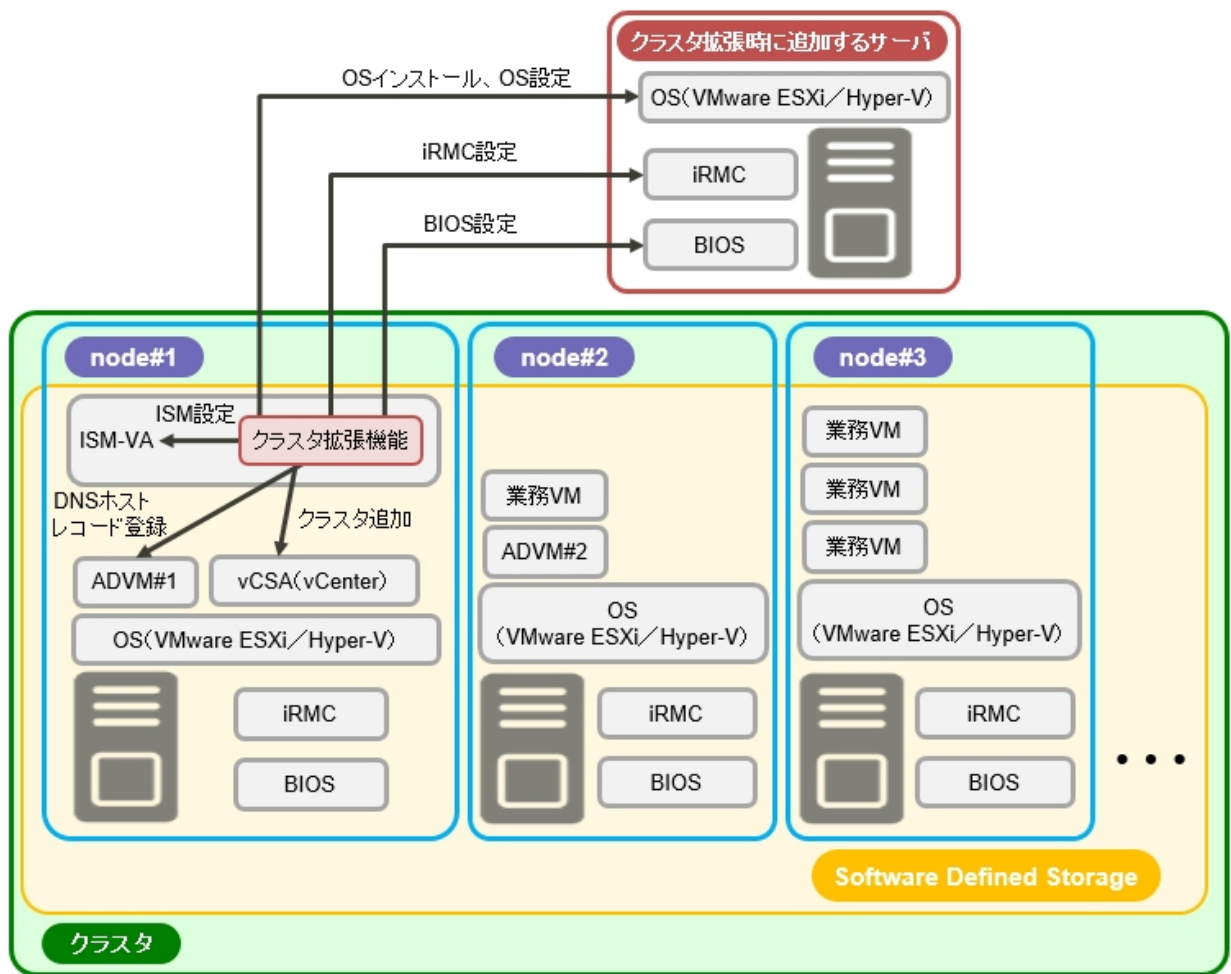
図2.22 クラスタ拡張機能の概要
