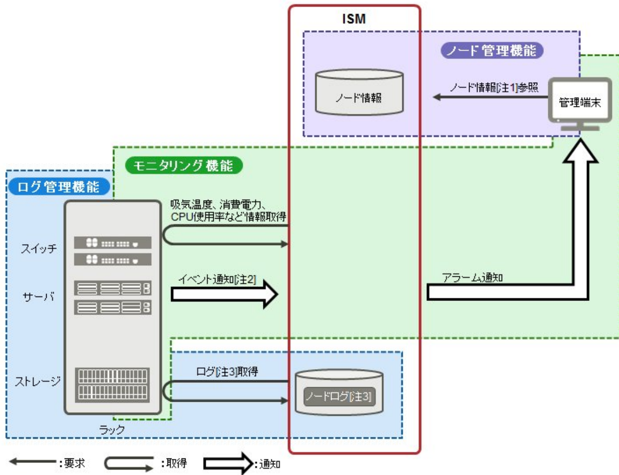
図1.6 機能イメージ(管理対象ノードの監視運用)
