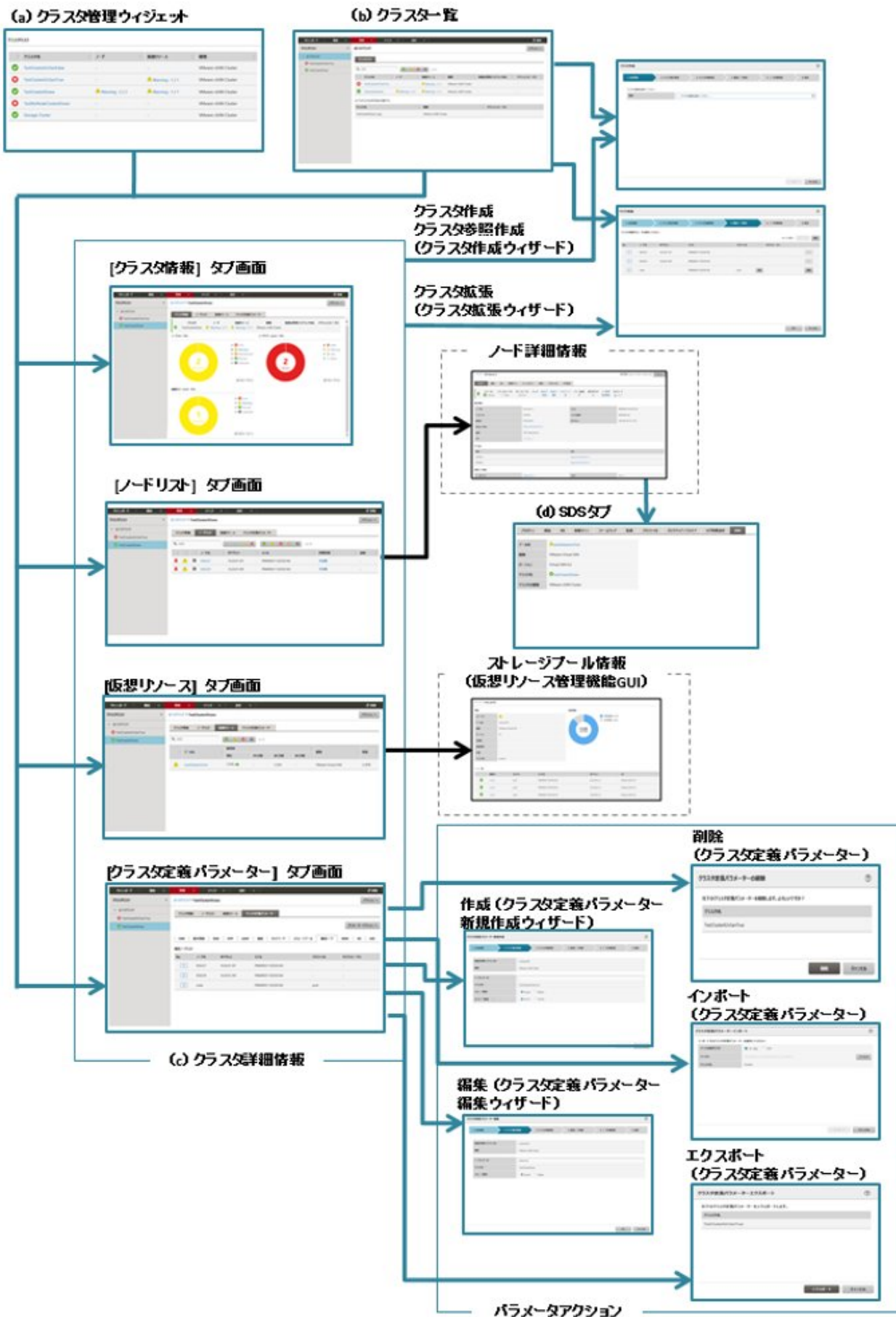
図2.17 クラスタ管理GUI
