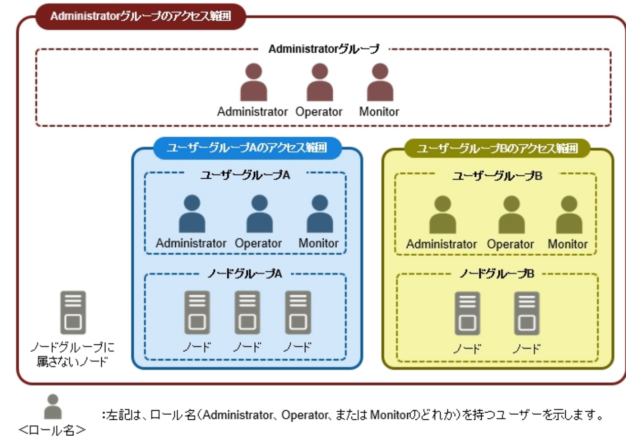
図2.24 ユーザーグループ、ノードグループ、ロールの関係
