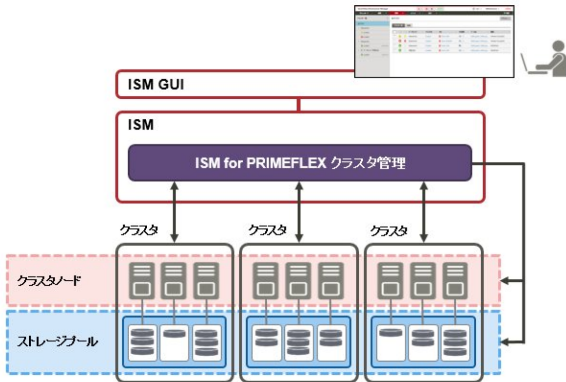
図2.16 クラスタ管理機能の動作環境の構成
