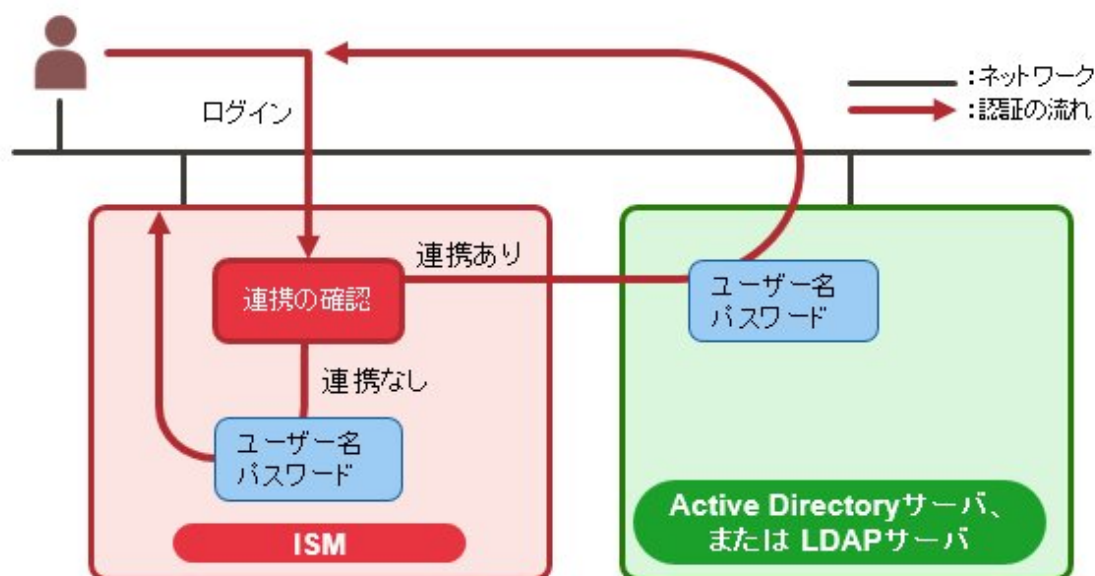
図2.25 ISMとMicrosoft Active Directory／LDAPとの連携イメージ
