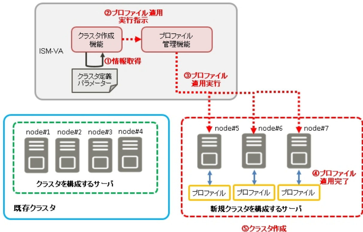
図2.21 クラスタ作成機能とプロファイル管理機能の連携
