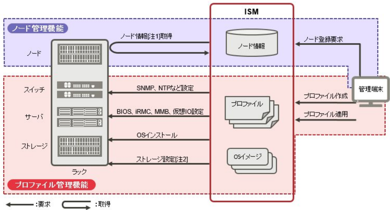
図1.5 機能イメージ(システムの構築)
