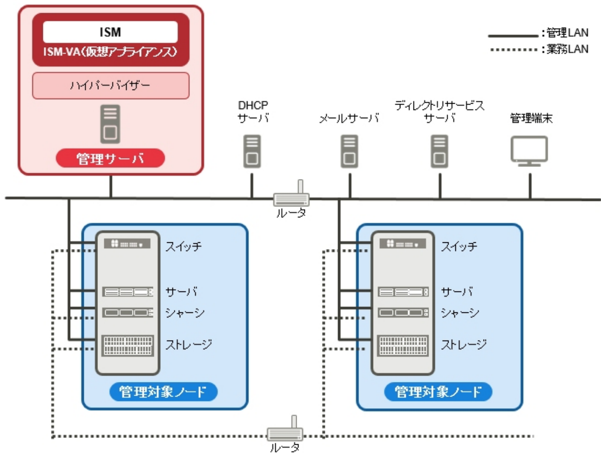
図1.8 ネットワーク構成
