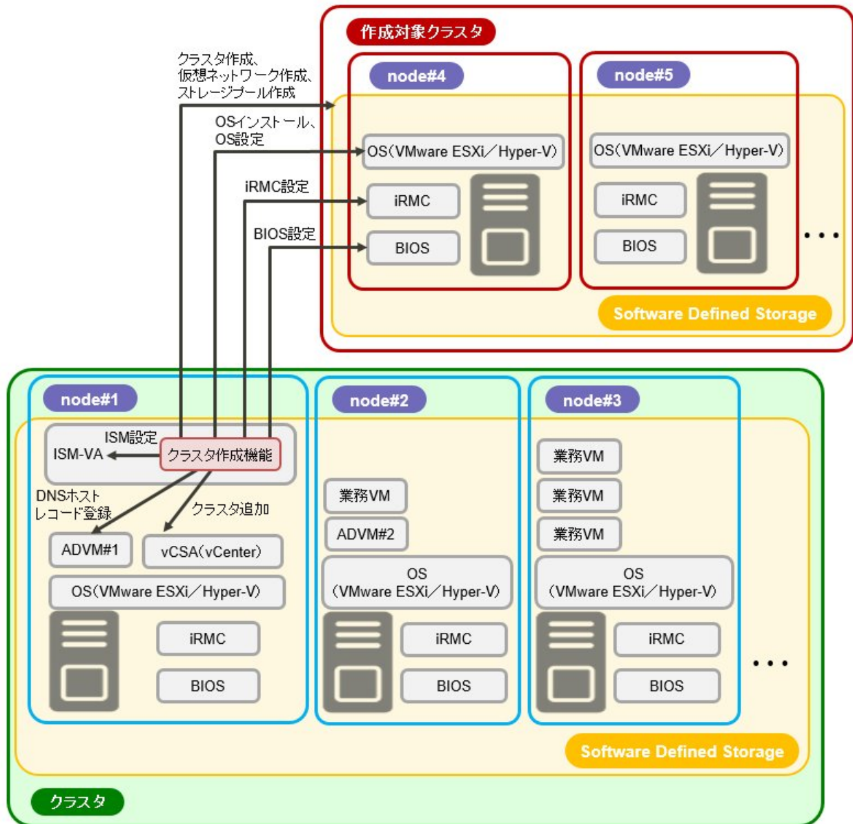
図2.20 クラスタ作成機能の概要
