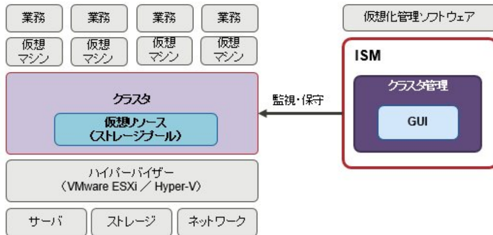
図2.15 クラスタ管理機能の概要
