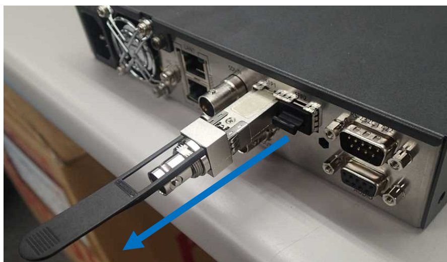
図 2-17 SFP モジュール取り外し方法
