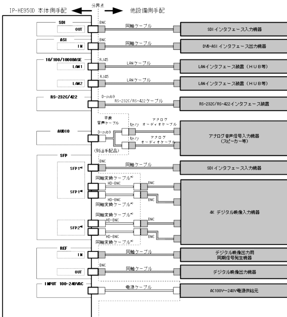
図 4-2 IP-HE950D 工事手配区分図
