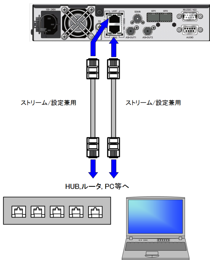
図 2-11 LAN 接続図
