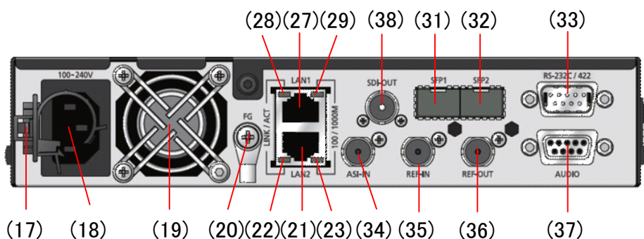
図 1-6 装置背面図 (IP-HE950D)
