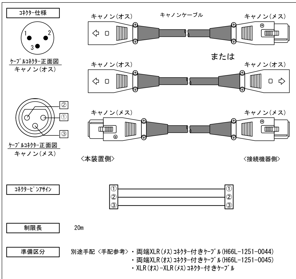
図 4-9 アナログオーディオケーブル図
