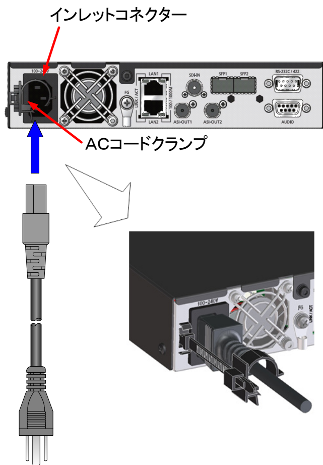
図 2-4 電源ケーブル接続図
