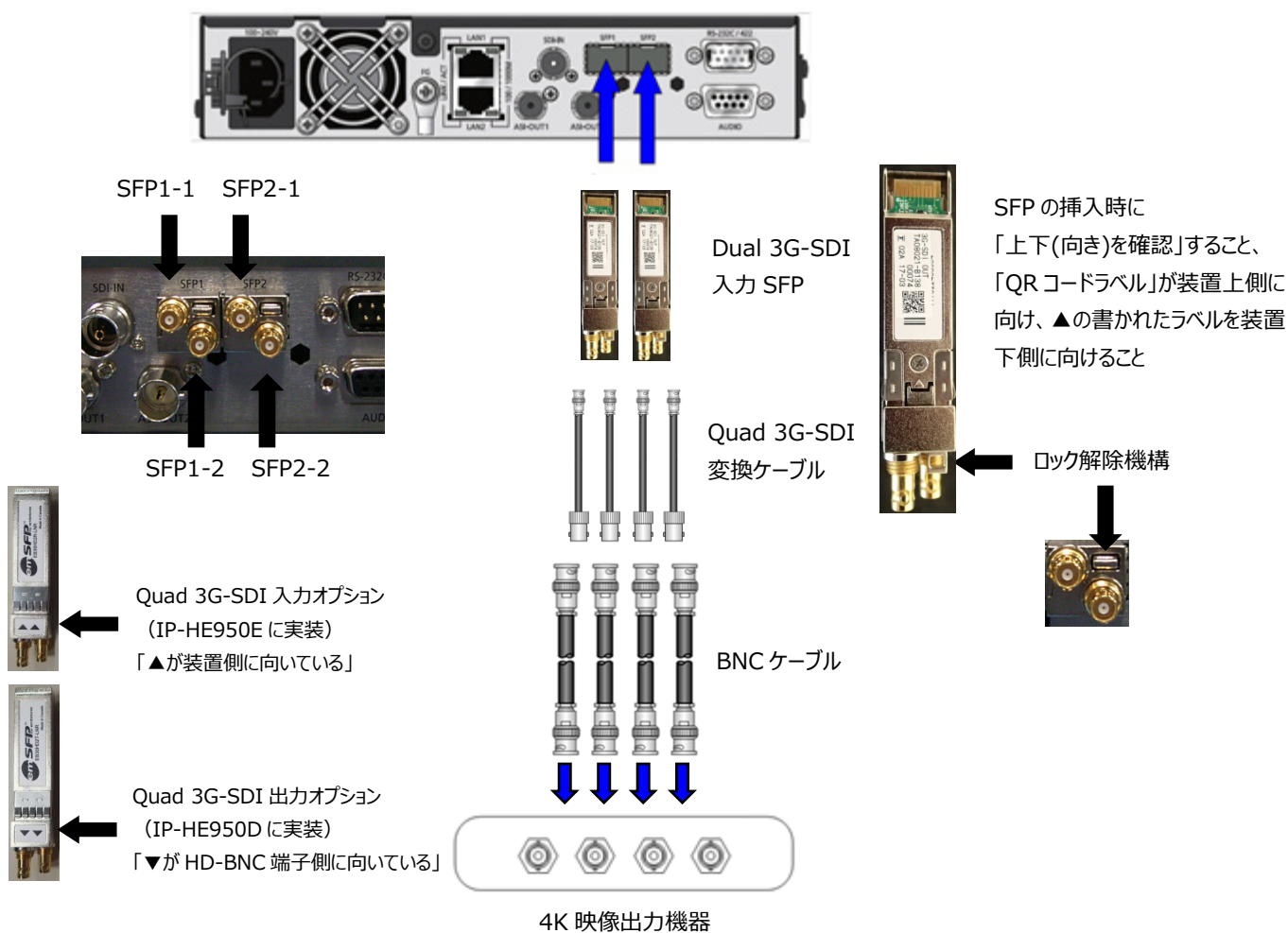
図 2-14 4K 映像出力機器 接続図
