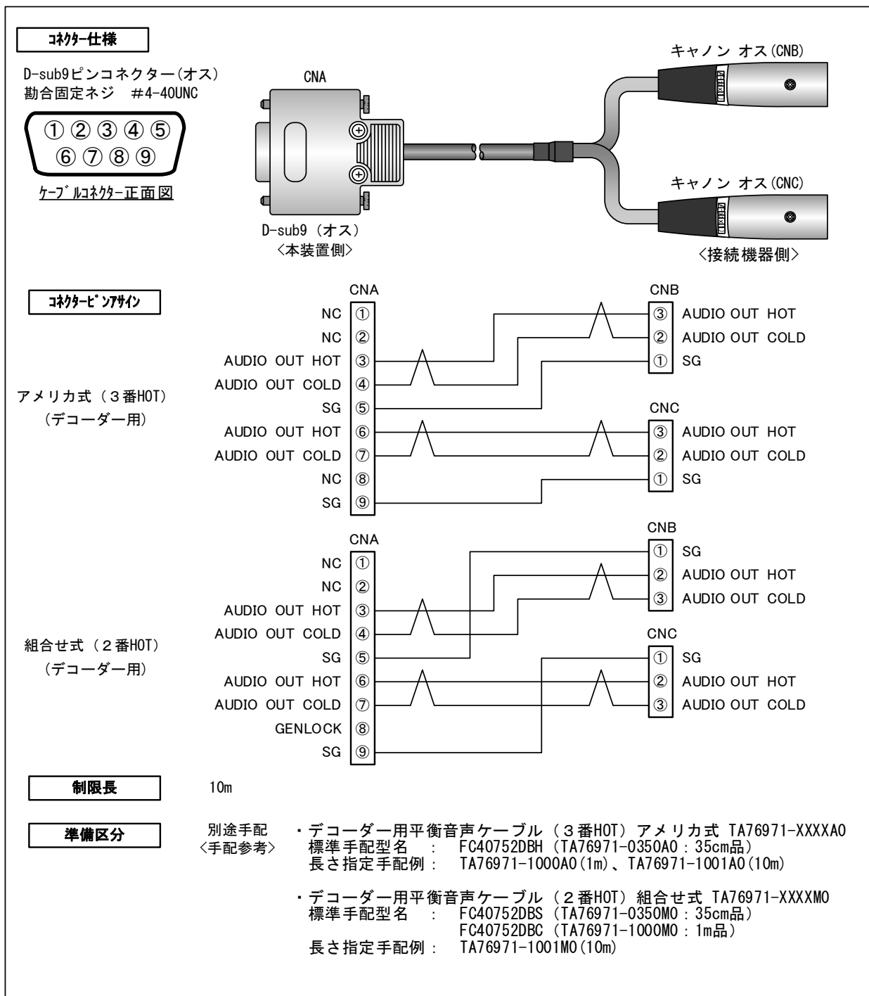
図 4-11 デコーダー用平衡音声ケーブル図
