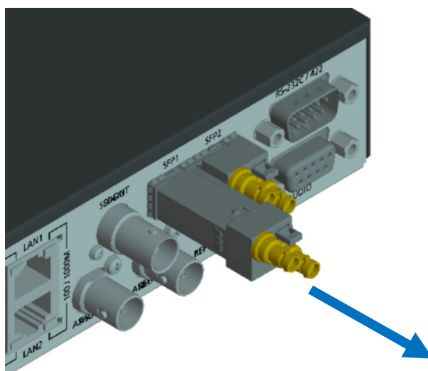
図 2-15 SFP モジュール取り外し方法
