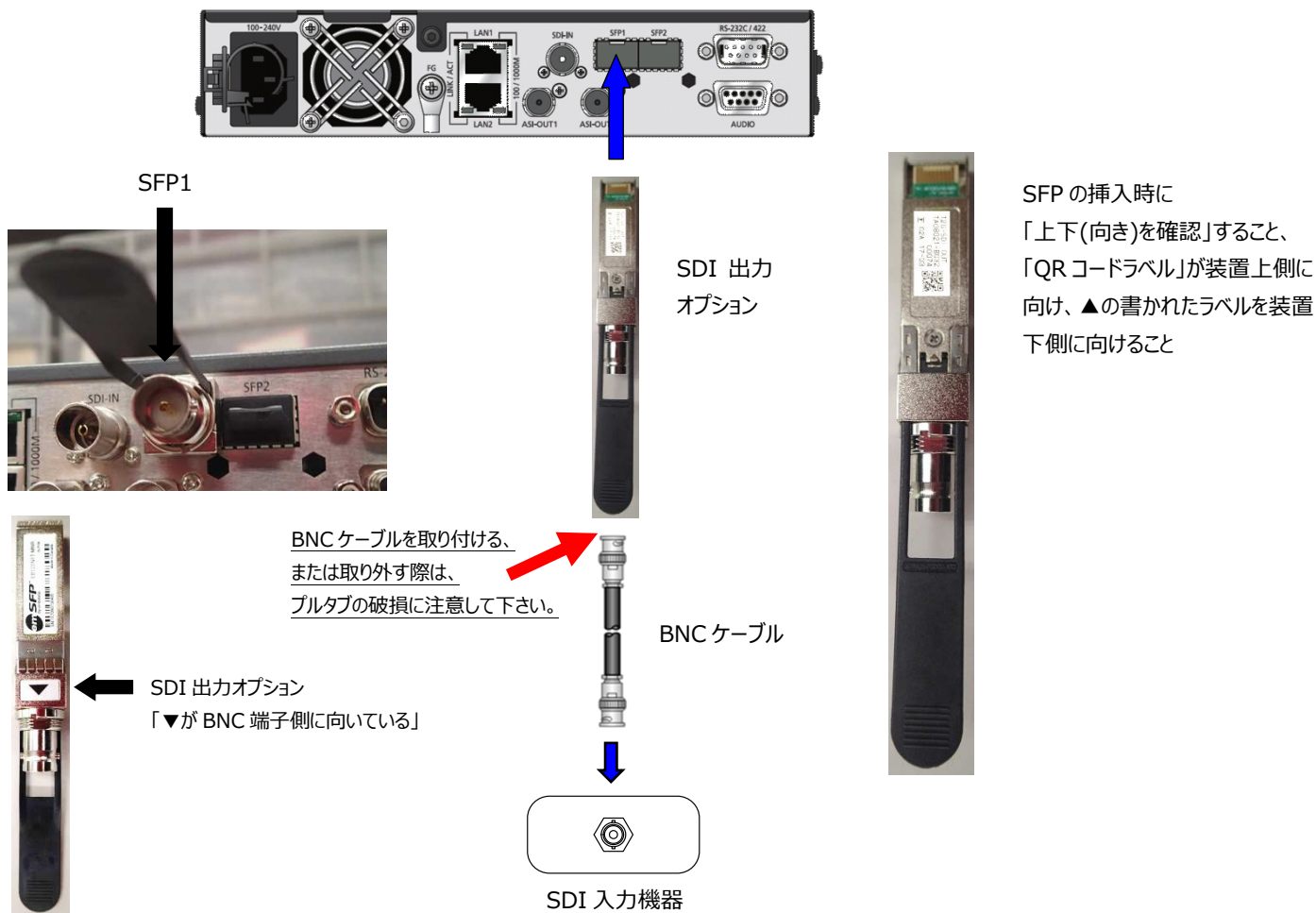
図 2-16 SDI 入力機器 接続図
