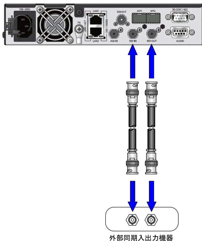
図 2-8 外部同期入出力機器 接続図
