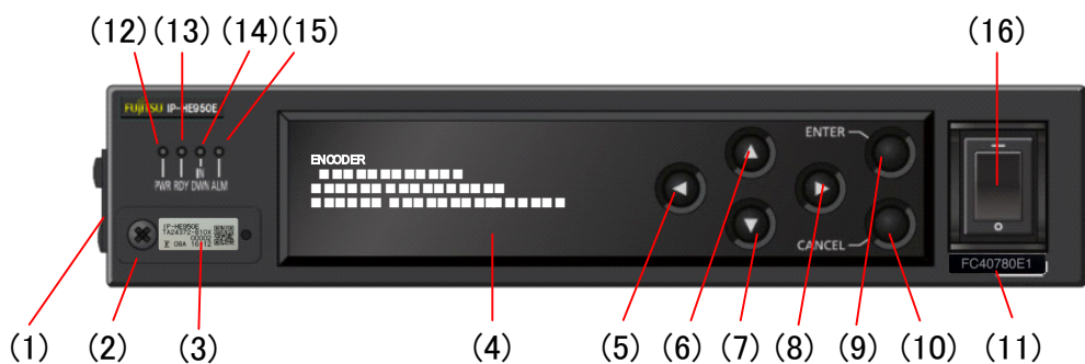
図 1-4 装置前面図 (IP-HE950E, IP-HE950D 共通)
