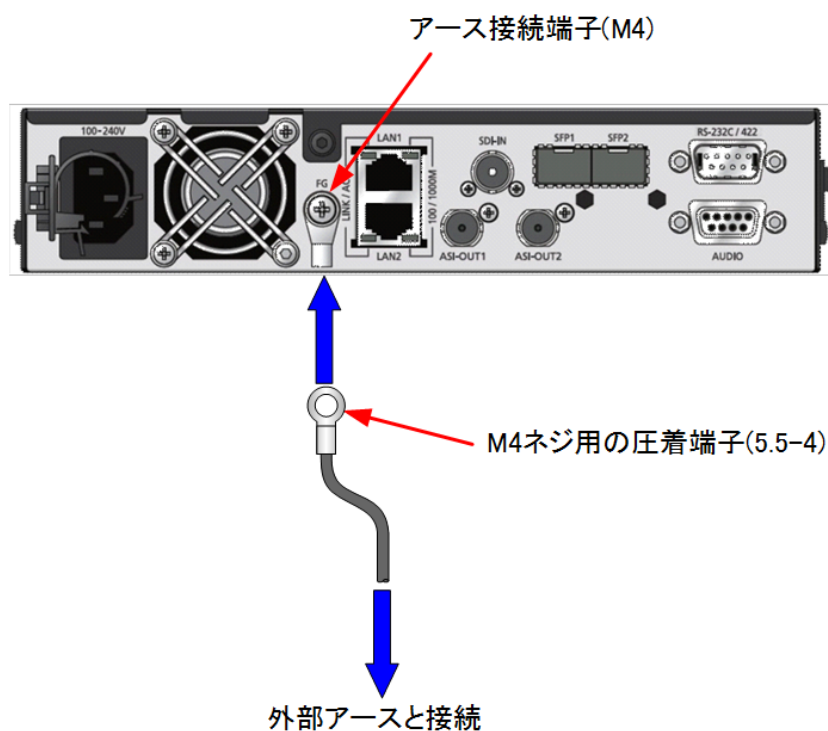
図 2-3 アース接続図
