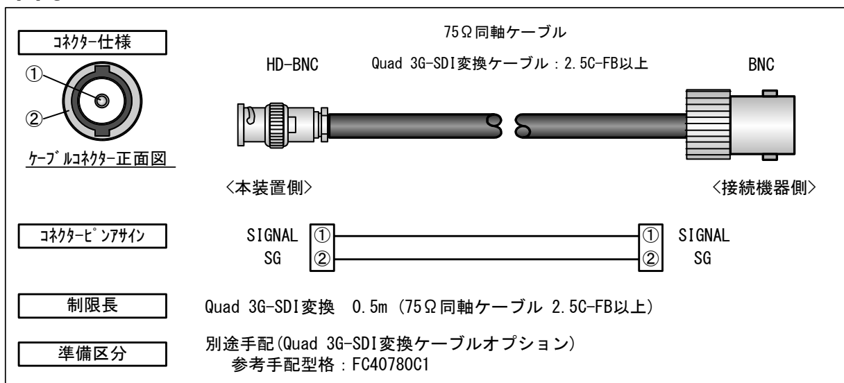
図 4-8 Quad 3G-SDI 変換ケーブル図
