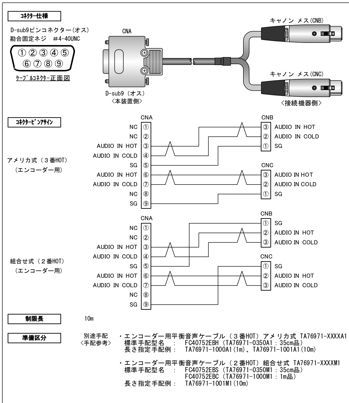
図 4-10 エンコーダー用平衡音声ケーブル図
