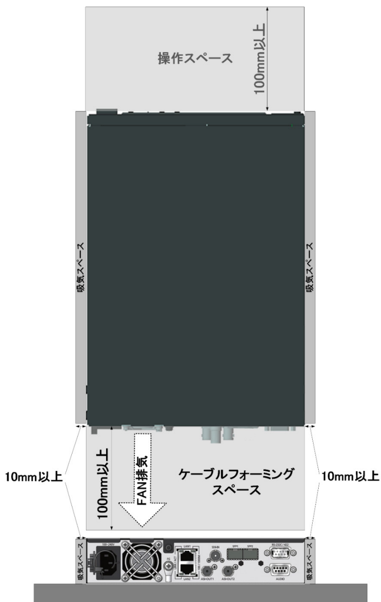
図 2-2 設置必要スペース図
