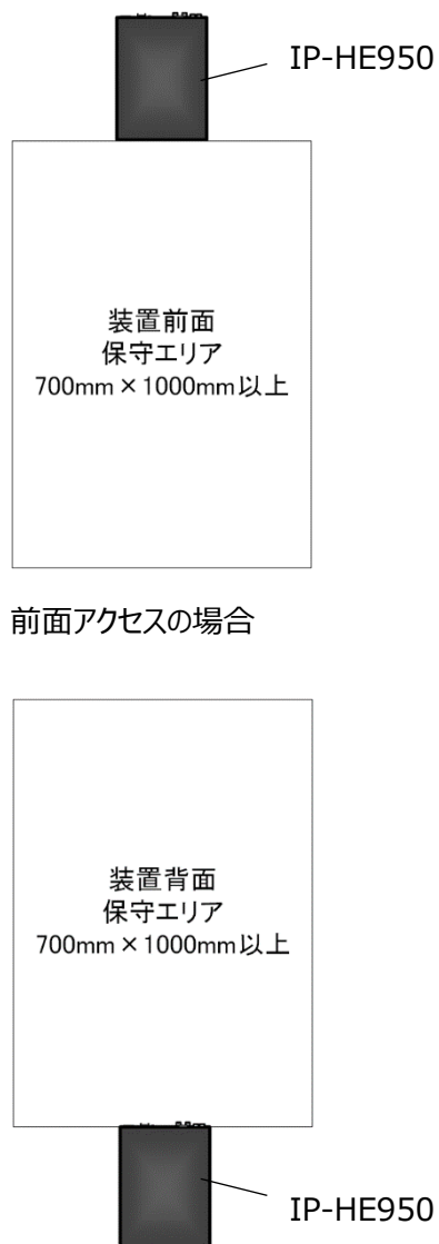
図 5-1 保守エリア (卓上設置)
