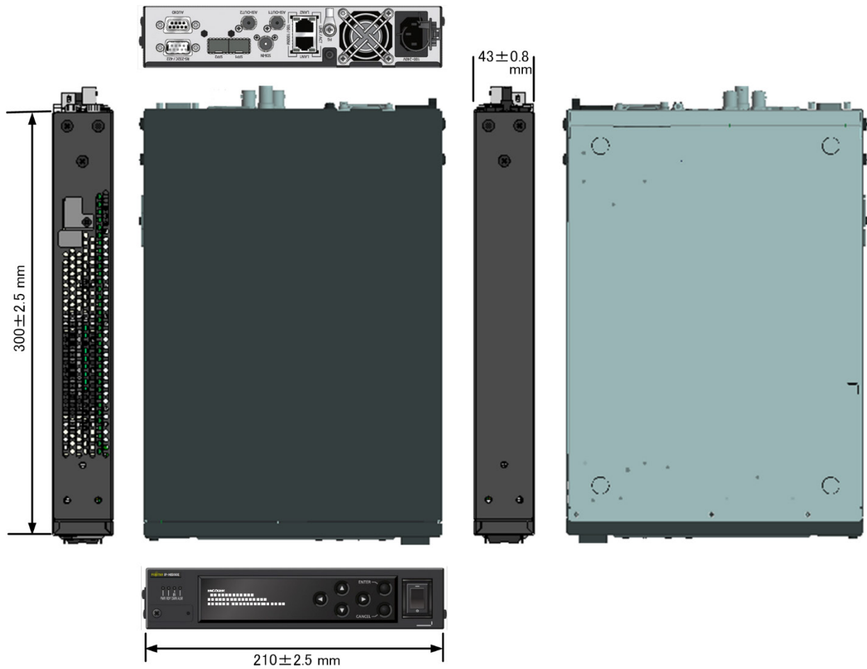
図 付録 1-1 IP-HE950E 装置外観図
