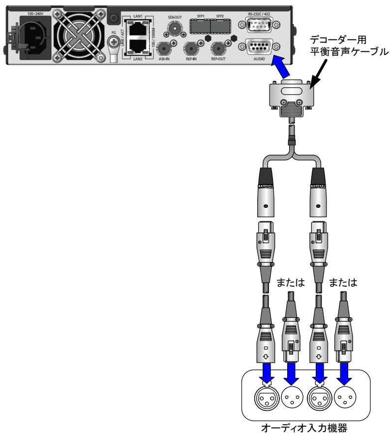
図 2-13 アナログオーディオ入力機器 接続図
