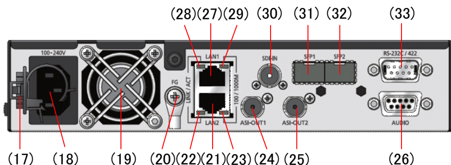
図 1-5 装置背面図 (IP-HE950E)
