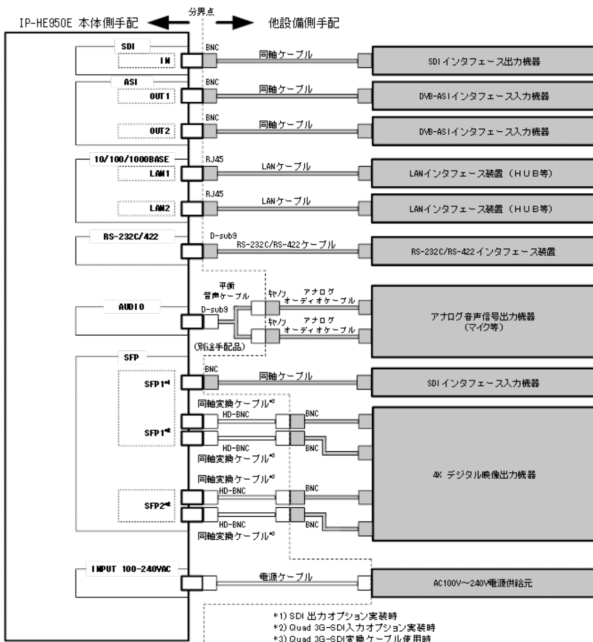
図 4-1 IP-HE950E 工事手配区分図
