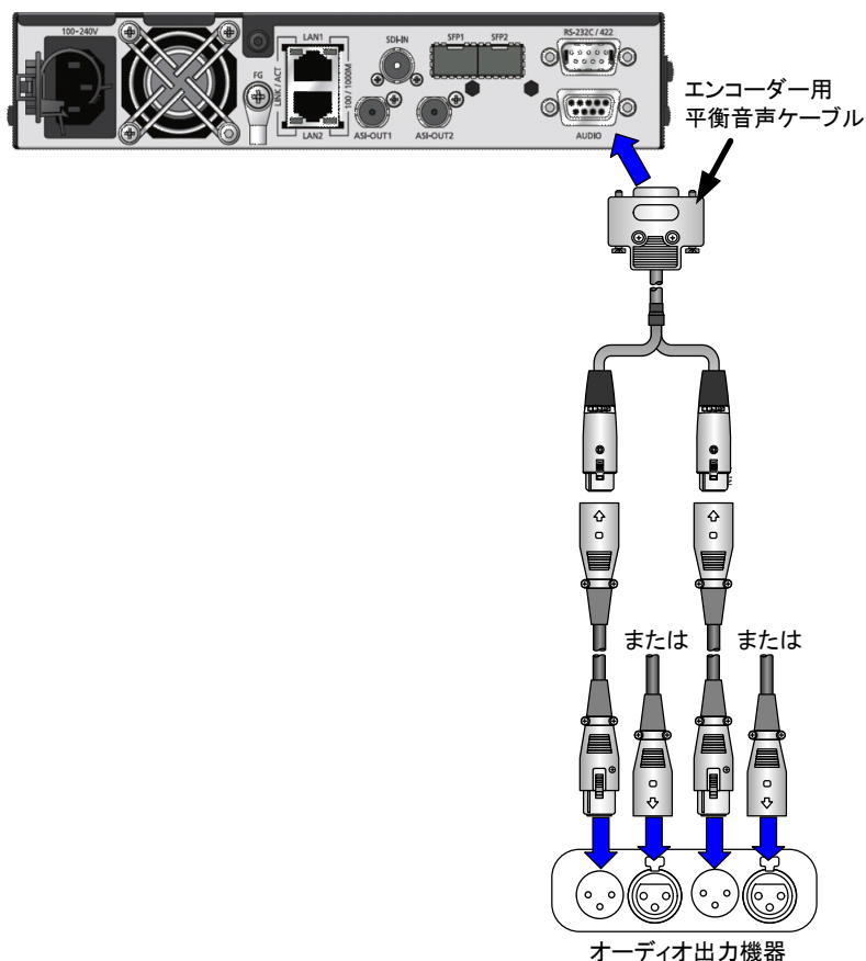
図 2-12 アナログオーディオ出力機器 接続図
