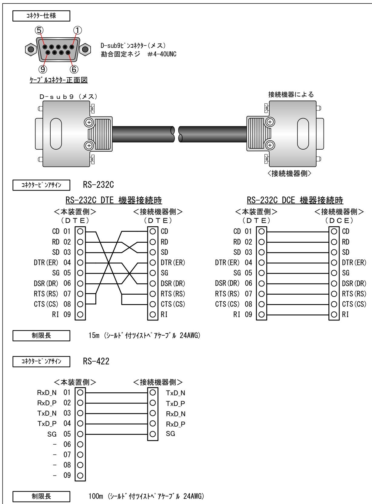
図 4-12 RS-232C/RS-422 ケーブル図
