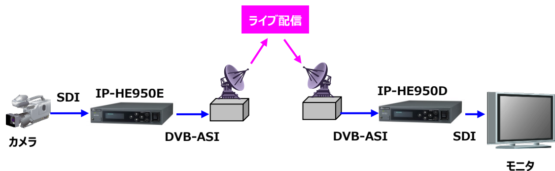
図 1-3 システム構成例:SNG
