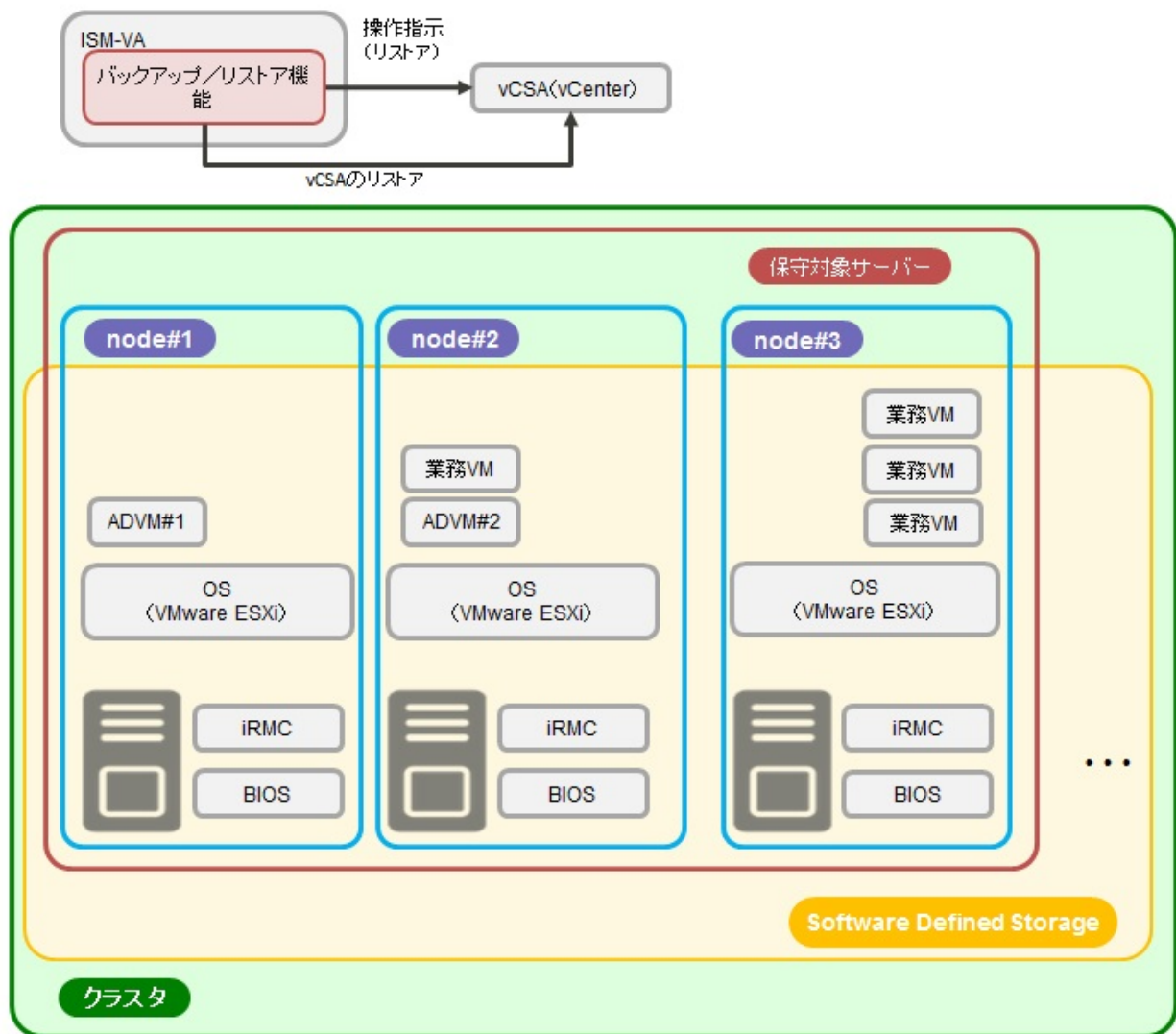
図2.45 リストア機能の動作概要
