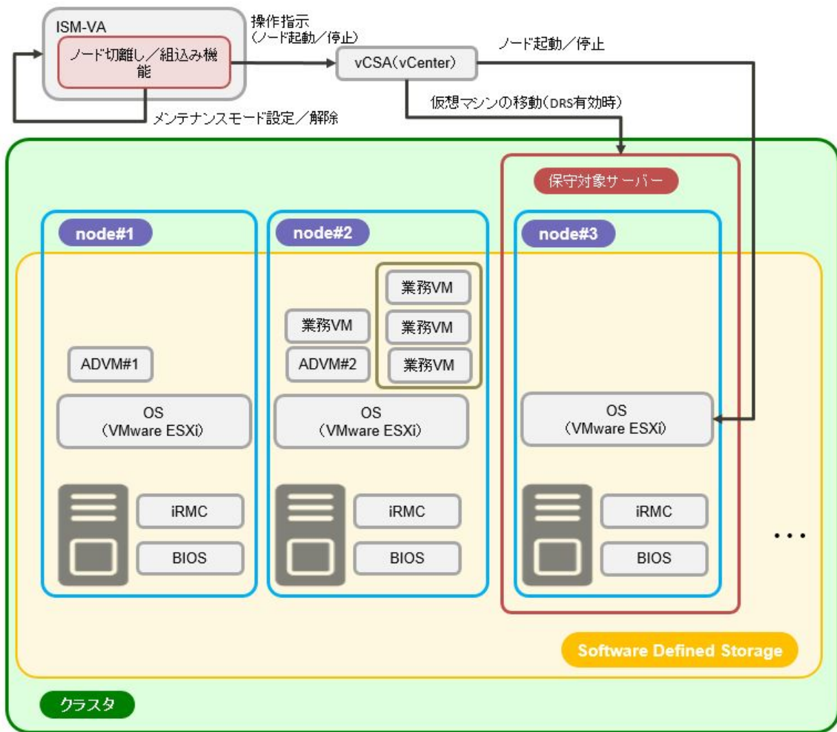
図2.43 ノード切離し／組込み機能の動作概要
