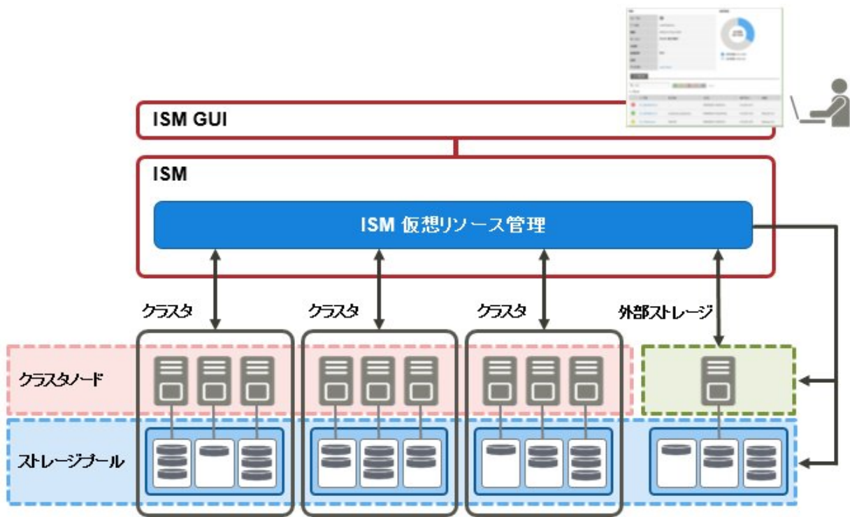
図2.26 仮想リソース管理機能の動作環境の構成
