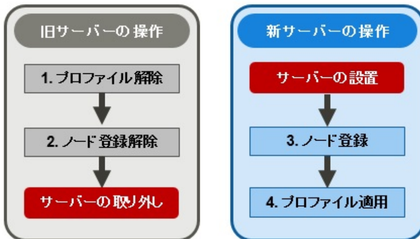
図2.19 仮想IOを設定した管理対象サーバーの交換
