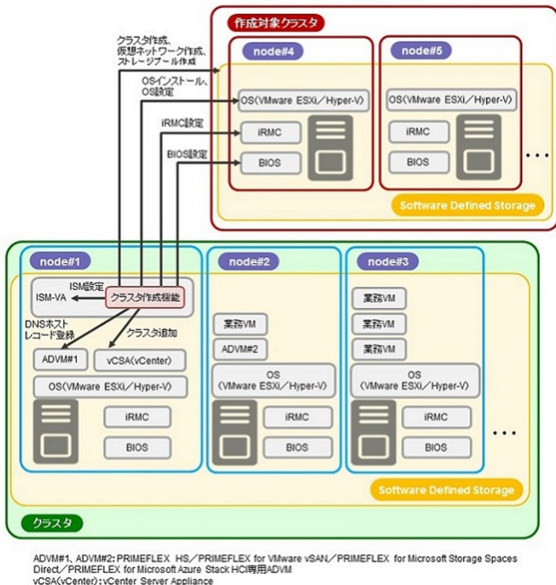
図2.37 クラスタ作成機能の動作概要
