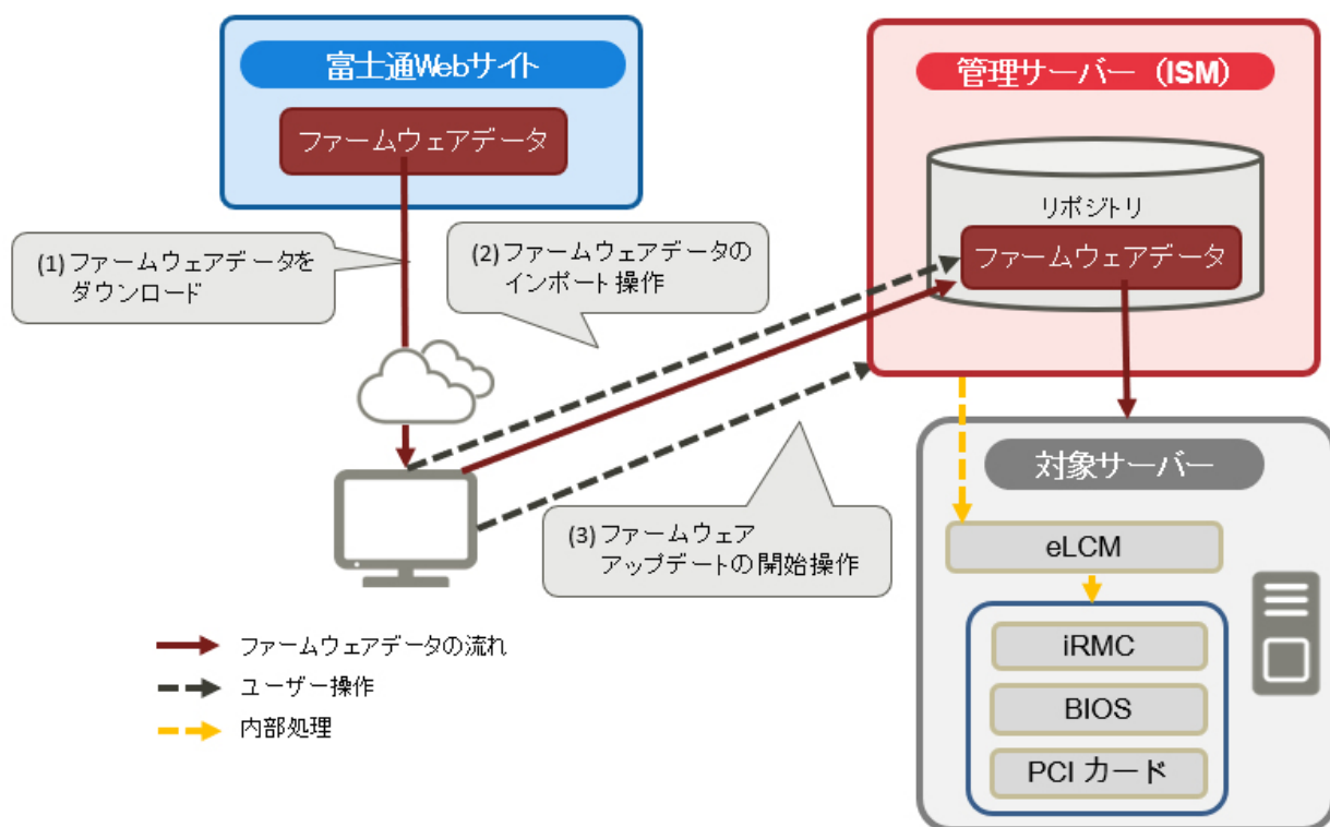
図2.24 ISMにインポートしたファームウェアデータを利用したアップデートの流れ
