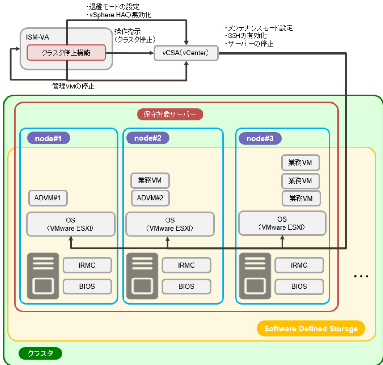
図2.46 クラスタ停止の動作概要
