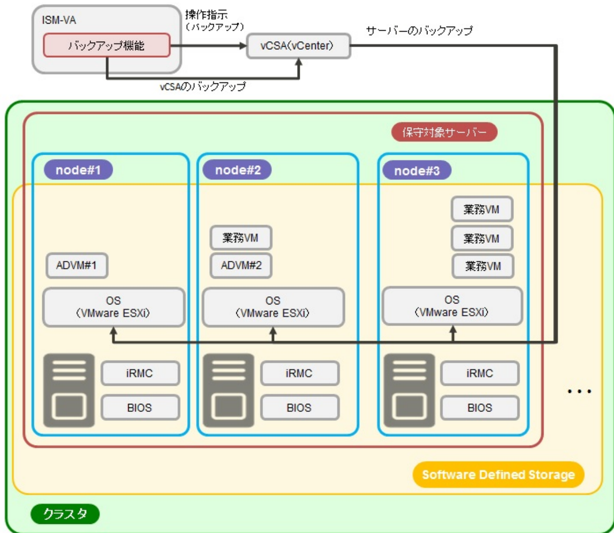
図2.44 バックアップ機能の動作概要
