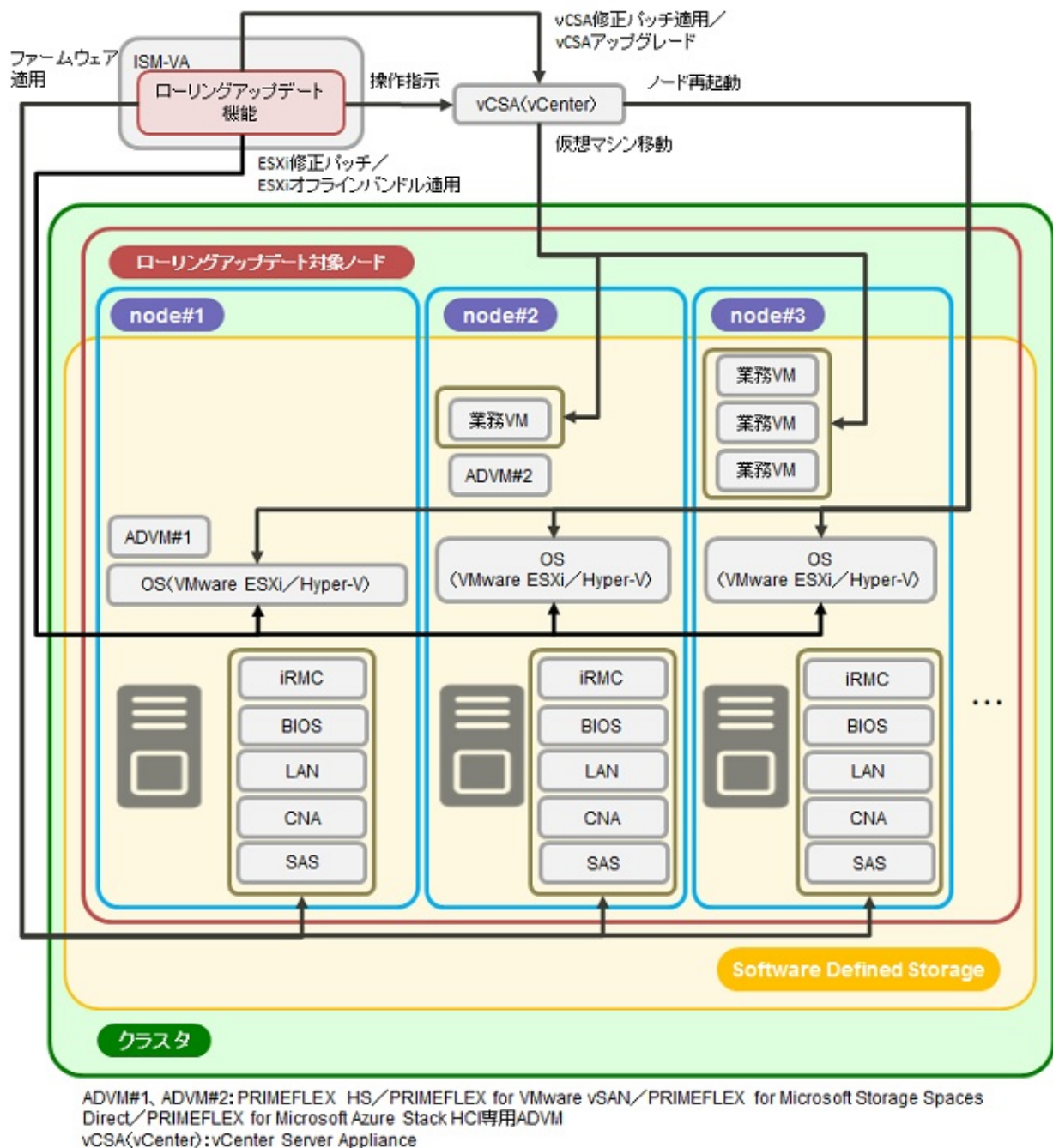
図2.41 ローリングアップデート機能の動作概要
