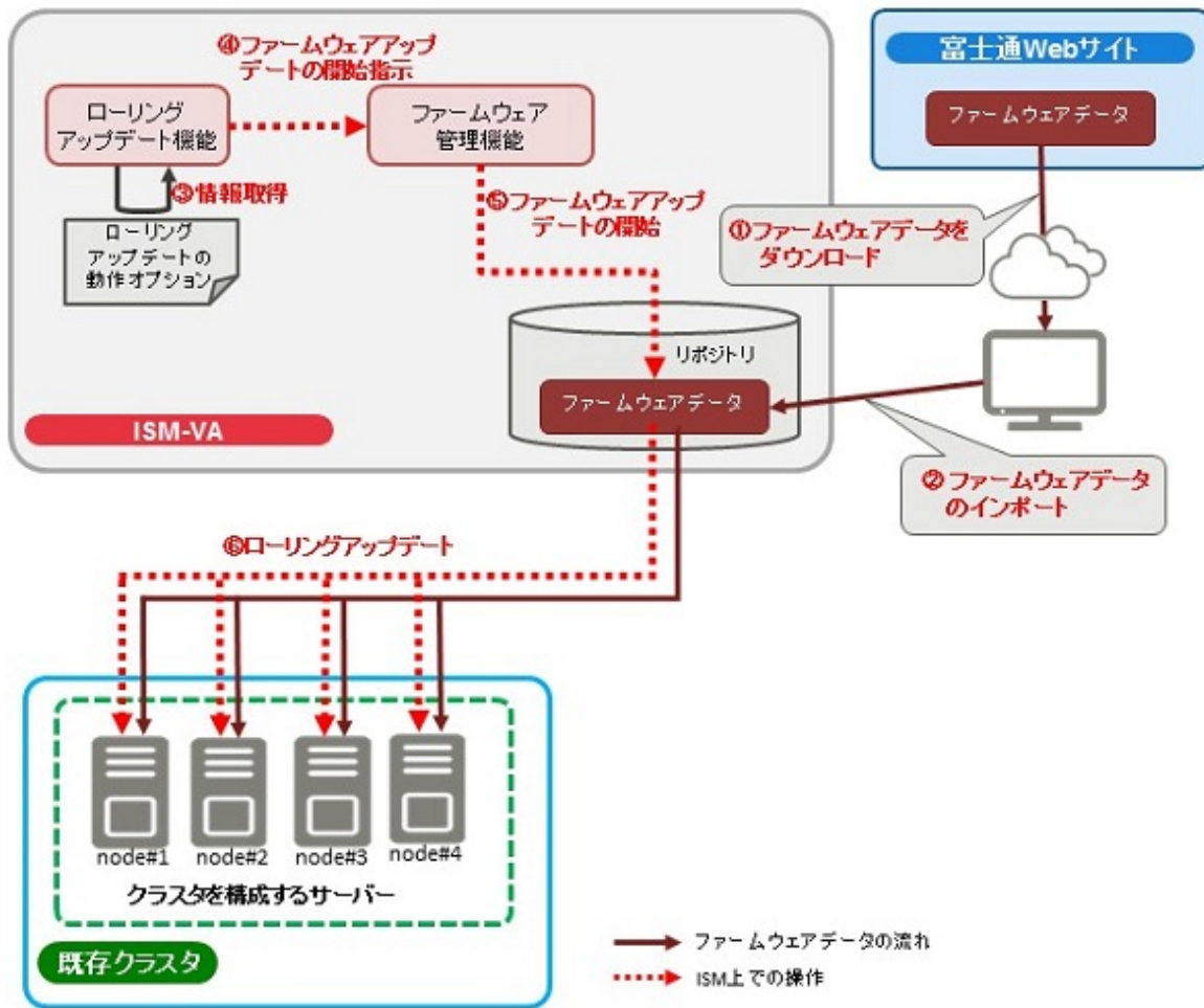
図2.42 ローリングアップデート機能とファームウェア管理機能の連携
