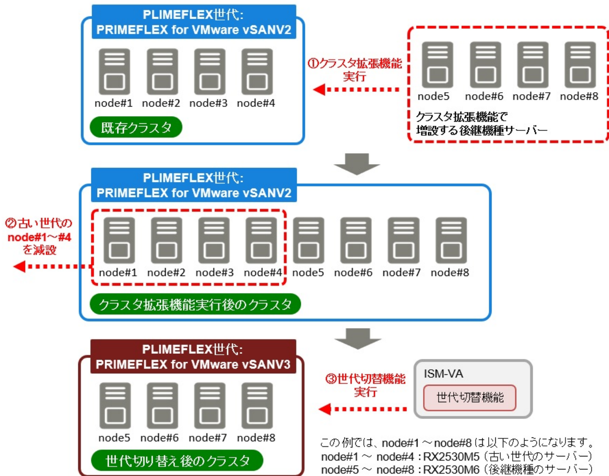
図2.49 世代切替機能の全体像
