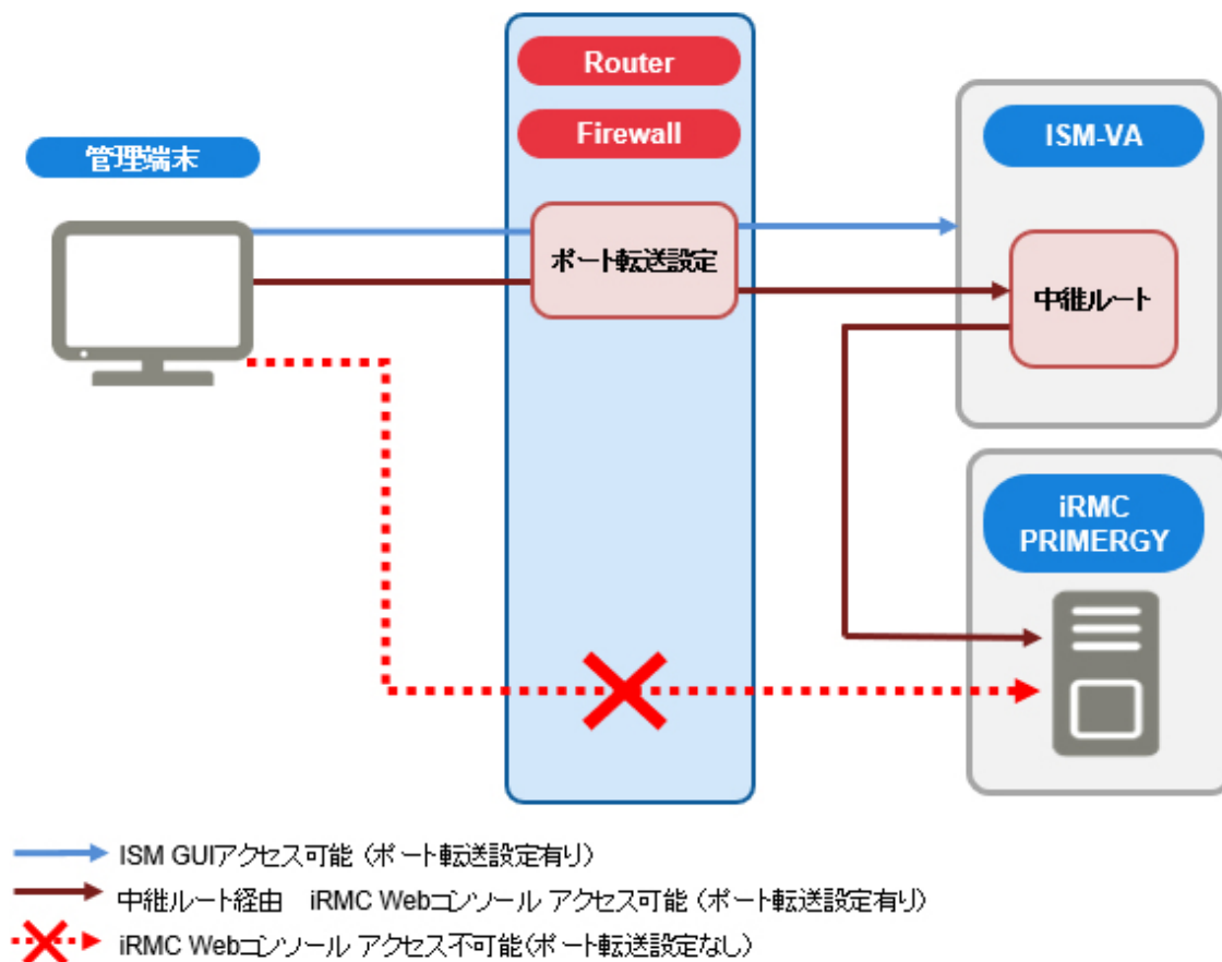
図2.12 中継ルート設定
