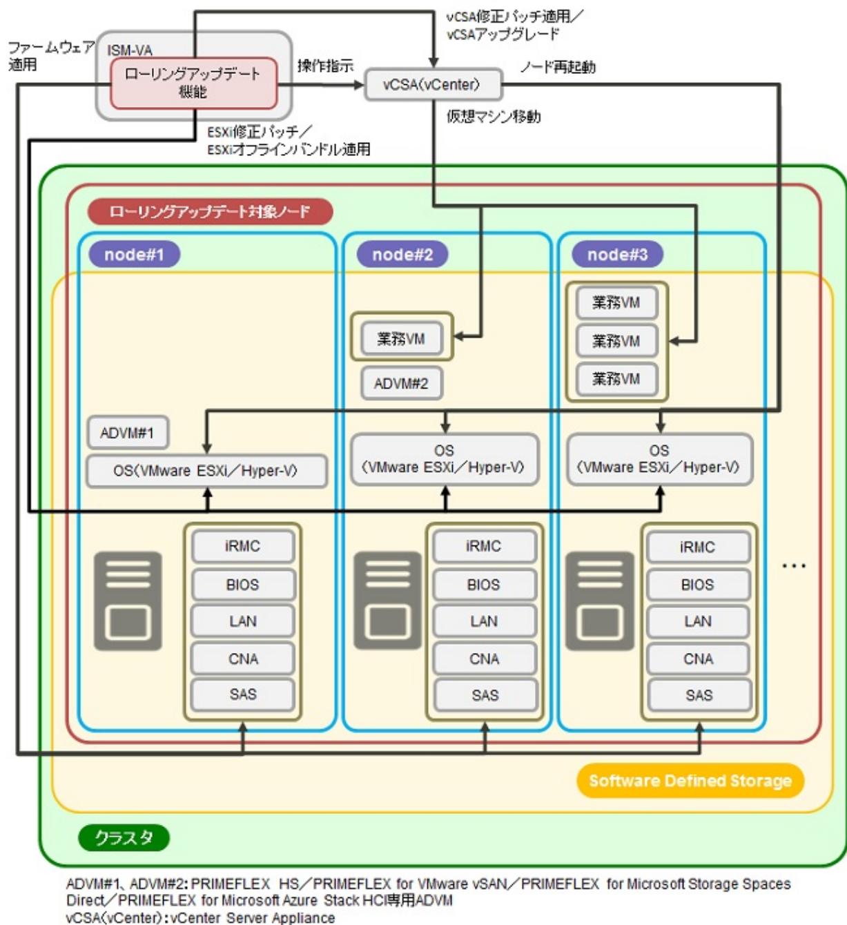
図2.37 ローリングアップデート機能の動作概要
