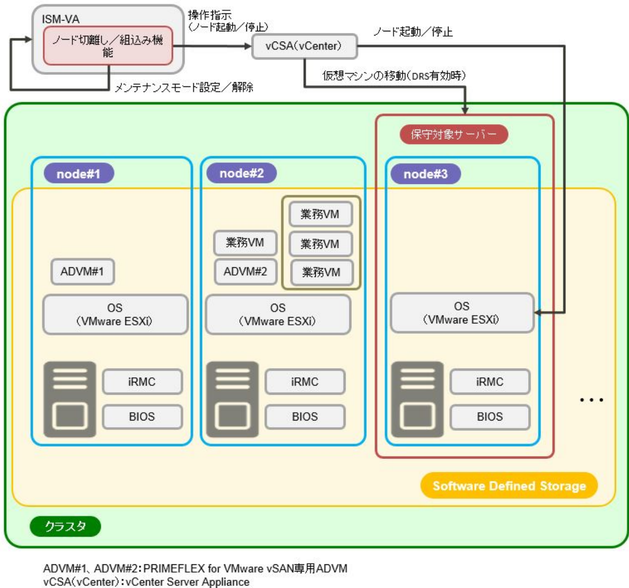
図2.39 ノード切離し／組込み機能の動作概要
