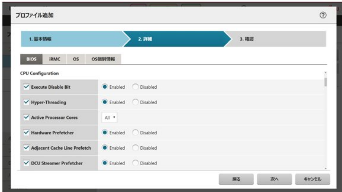
図2.12 「プロファイル作成」画面例 (GUI)
