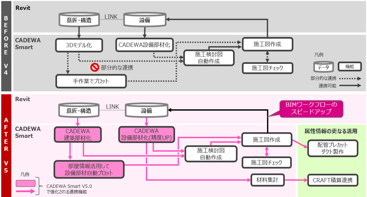
図2：RevitとCADEWA Smart V5.0の互換強化による高度機能の利活用
