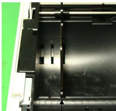
60mm セット溝
