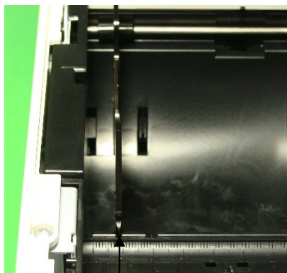
70mm セット溝
