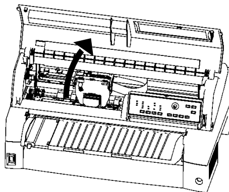
Preparación para instalar la cinta
