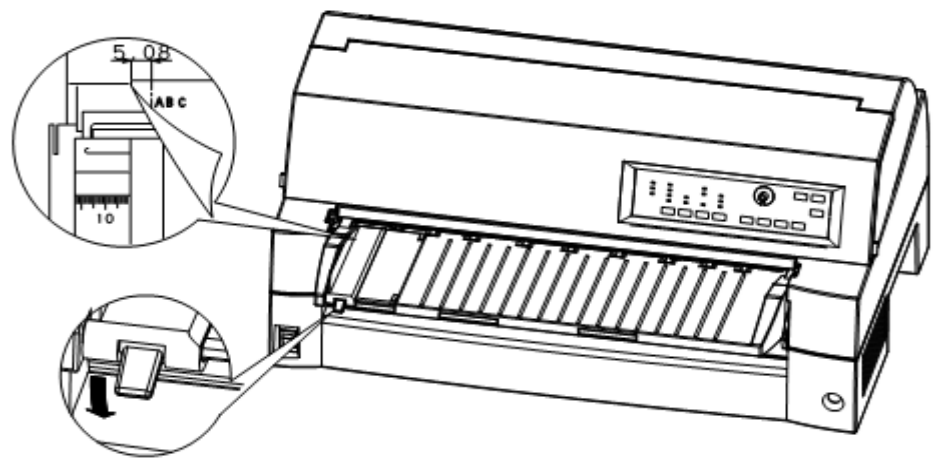
Preparación para cargar una hoja de papel
