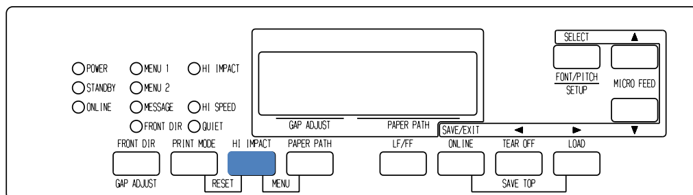
Panel de control de impresión
