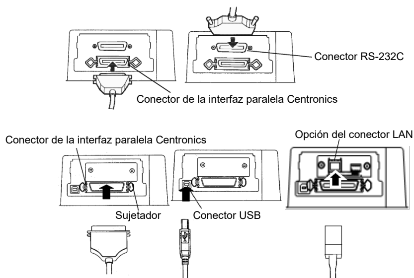
Conexión de la interfaz
