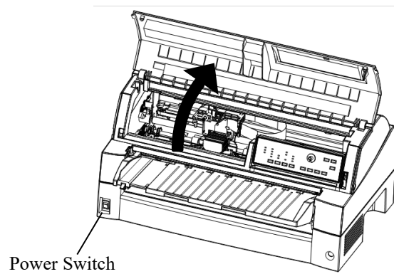
Preparación para instalar la cinta
