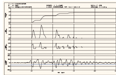
滑動変位の時刻歴図
