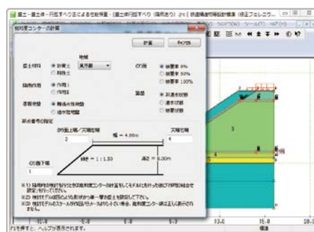
降雨時の飽和度コンター計算
