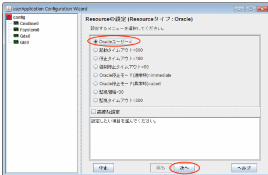
図14.49 Oracleインスタンス設定画面
