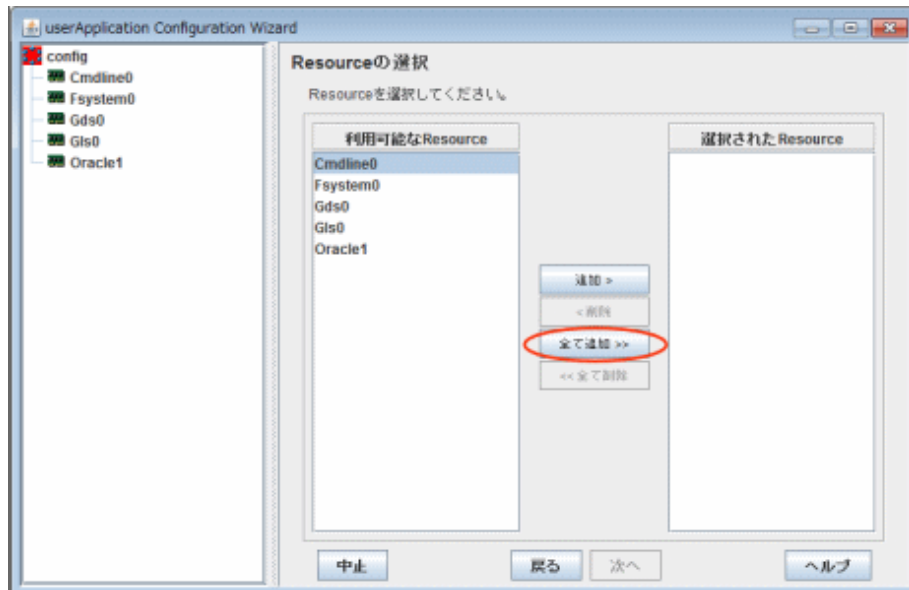
図14.61 “Resourceの選択”画面
