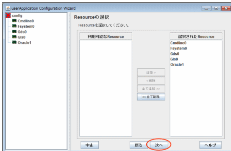
図14.62 “Resourceの選択”追加後の画面
