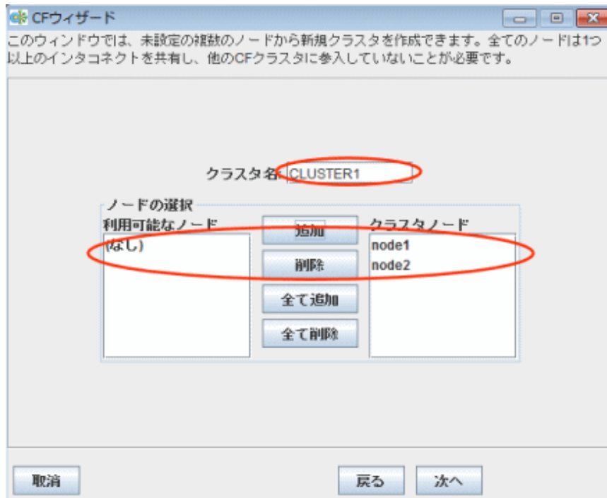
図5.8 クラスタ作成画面
