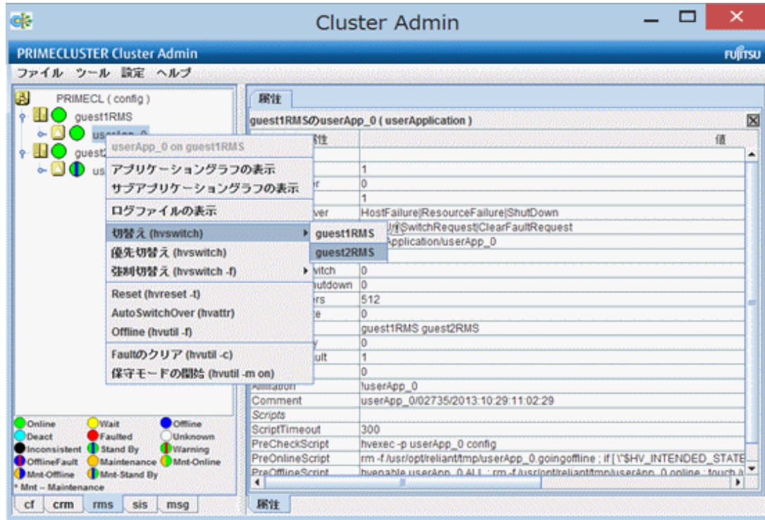
図14.77 クラスタアプリケーション切替メニュー
