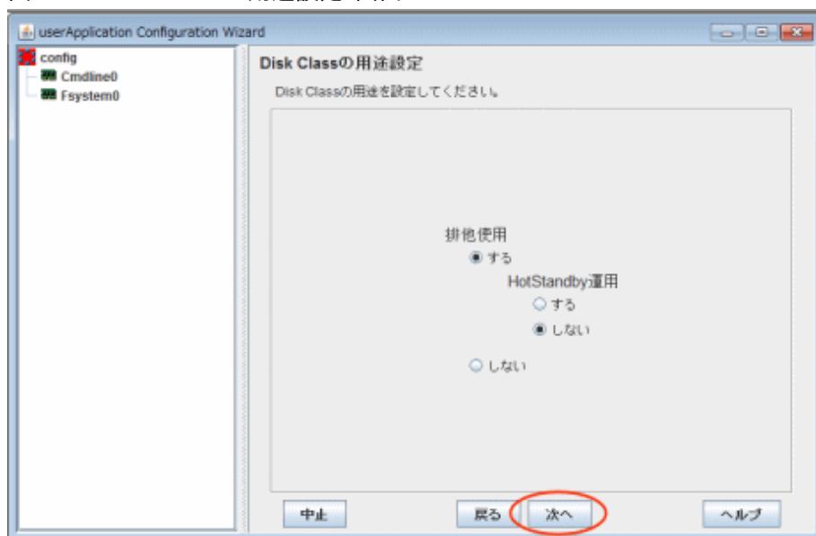
図14.35 “Disk Classの用途設定”画面
