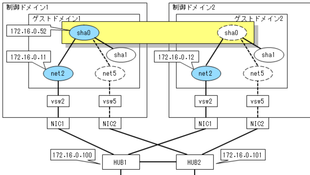
図14.1 ゲストドメインでのGLSの環境設定例
