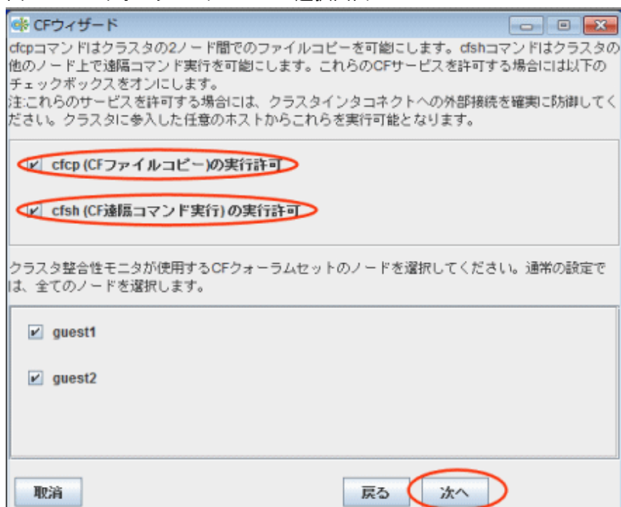
図11.13 CFクォーラムセットのノード選択画面
