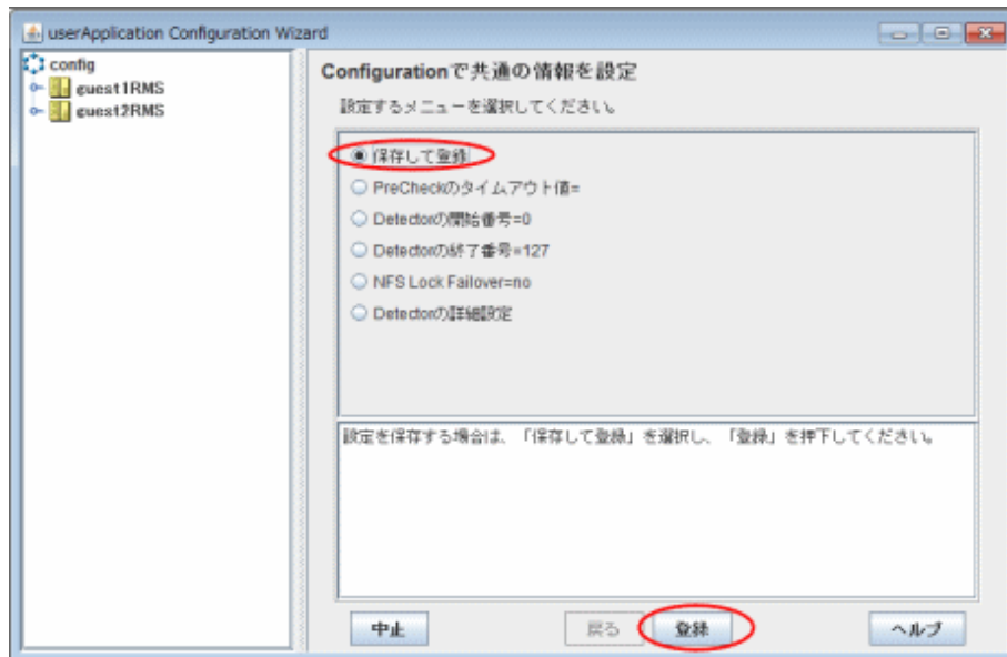
図14.66 “Configuration内の共通情報を設定”画面
