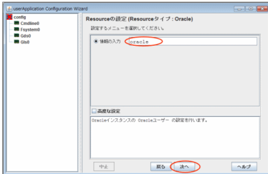
図14.50 Oracleユーザー名設定画面
