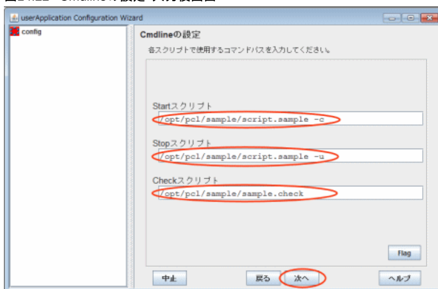
図14.22 “Cmdlineの設定”入力後画面
