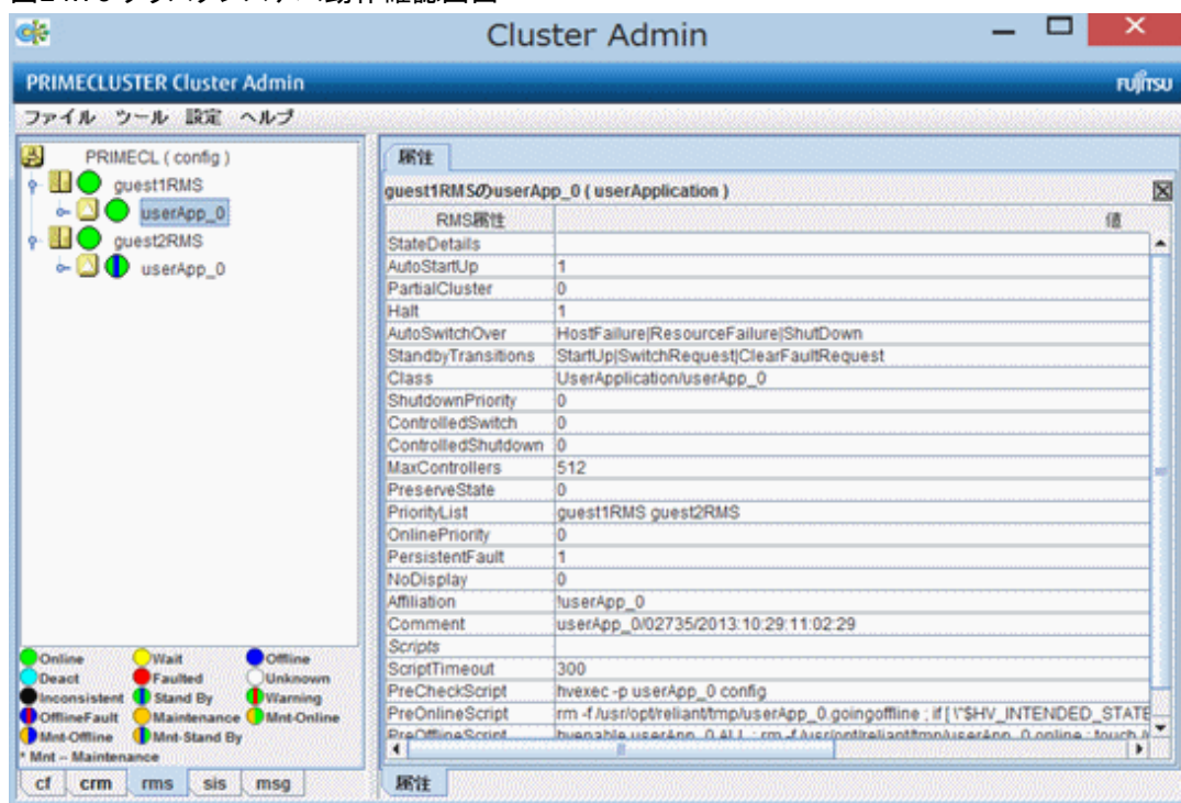
図14.76 クラスタシステム動作確認画面
