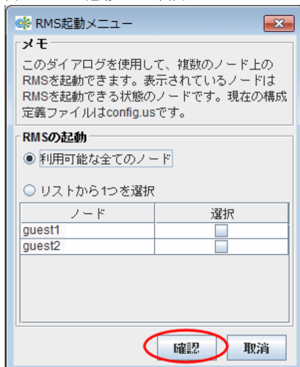
図14.73 RMS起動メニュー画面
