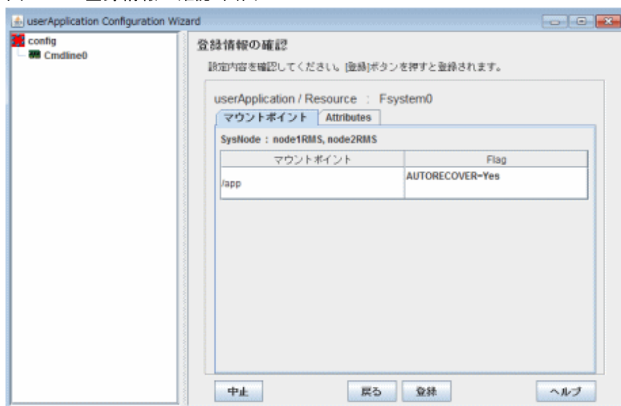
図14.29 “登録情報の確認”画面
