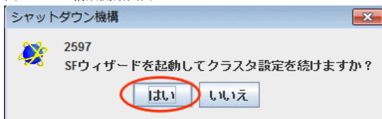
図11.18 SF構成開始画面
