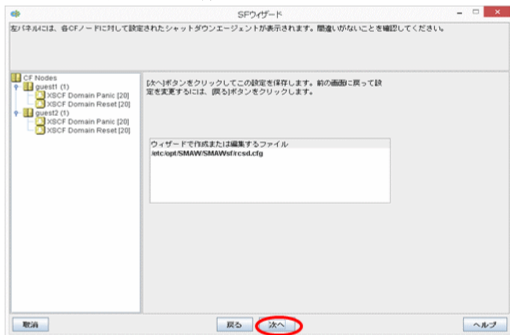
図12.4 シャットダウンエージェント確認画面
