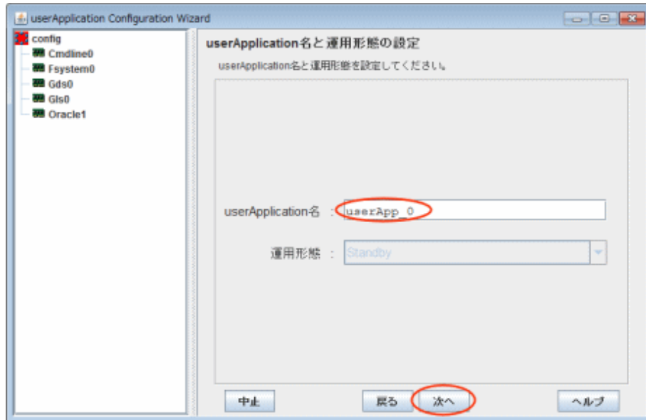
図14.58 “userApplication名と運用形態の設定”画面
