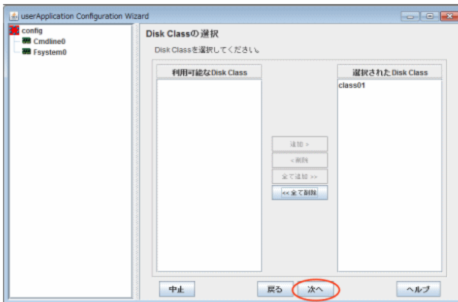
図14.33 “Disk Classの選択”追加後画面
