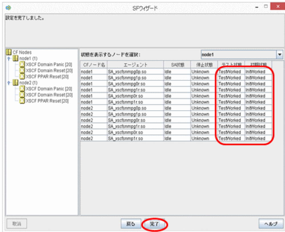
図6.6 シャットダウン機構の構成状態表示画面
