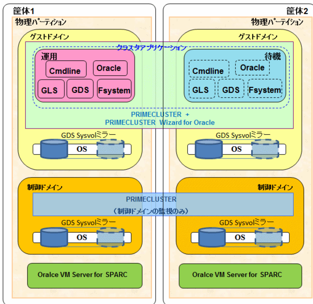
図1.1 ゲストドメイン間クラスタ
