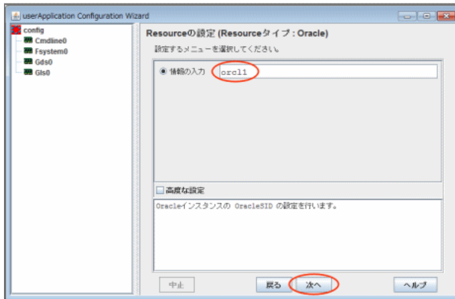
図14.48 OracleSID入力画面
