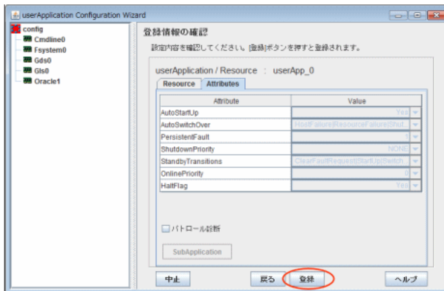
図14.64 設定内容登録確認画面
