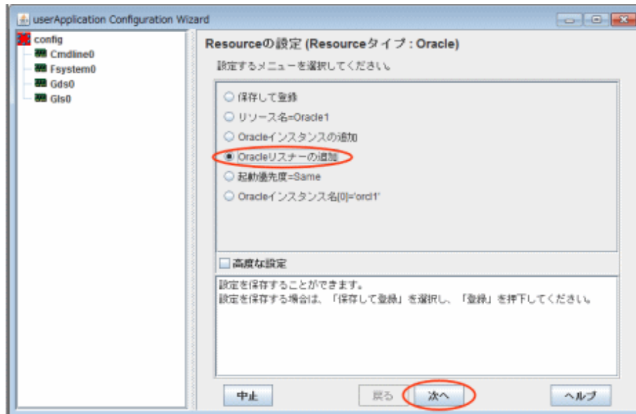
図14.52 Oracleリスナー追加選択画面
