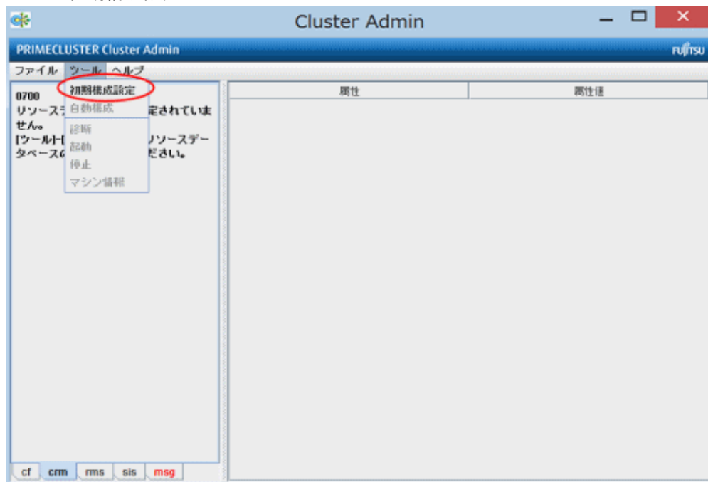
図13.2 初期構成設定メニュー画面
