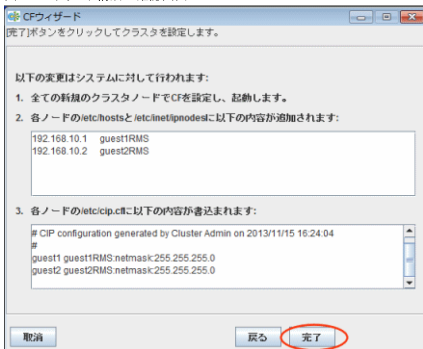
図11.14 クラスタ構成の確認画面
