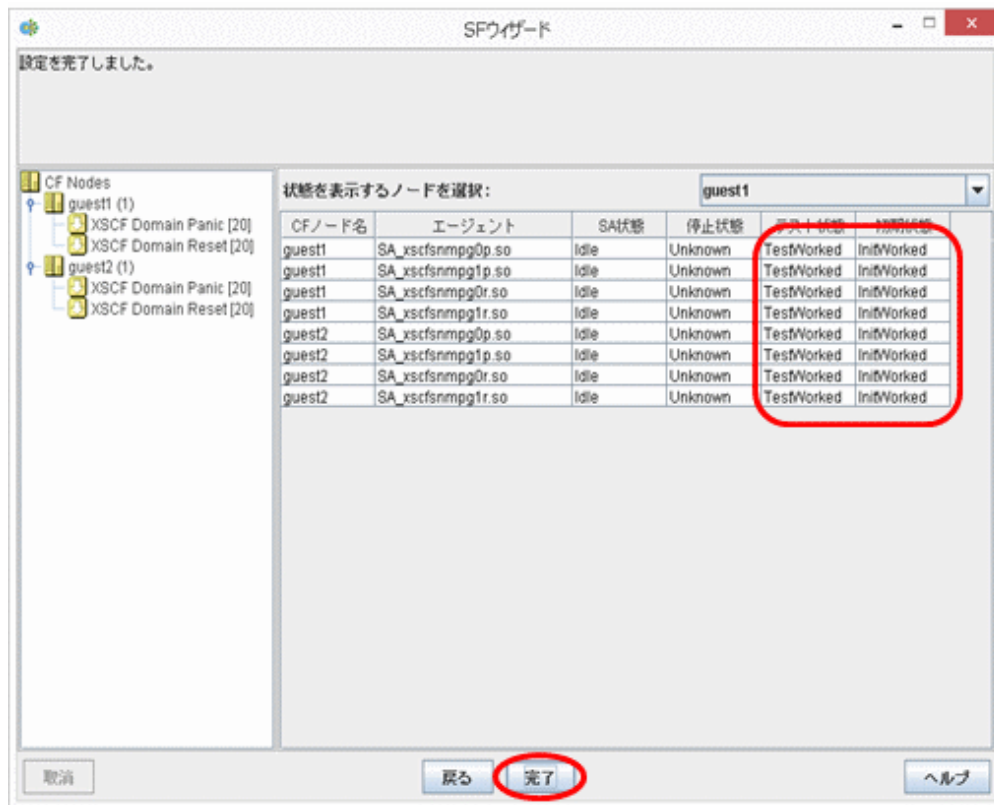
図12.6 シャットダウン機構の構成状態表示画面
