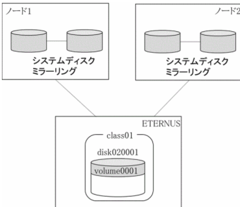
図14.2 GDS共用クラスイメージ
