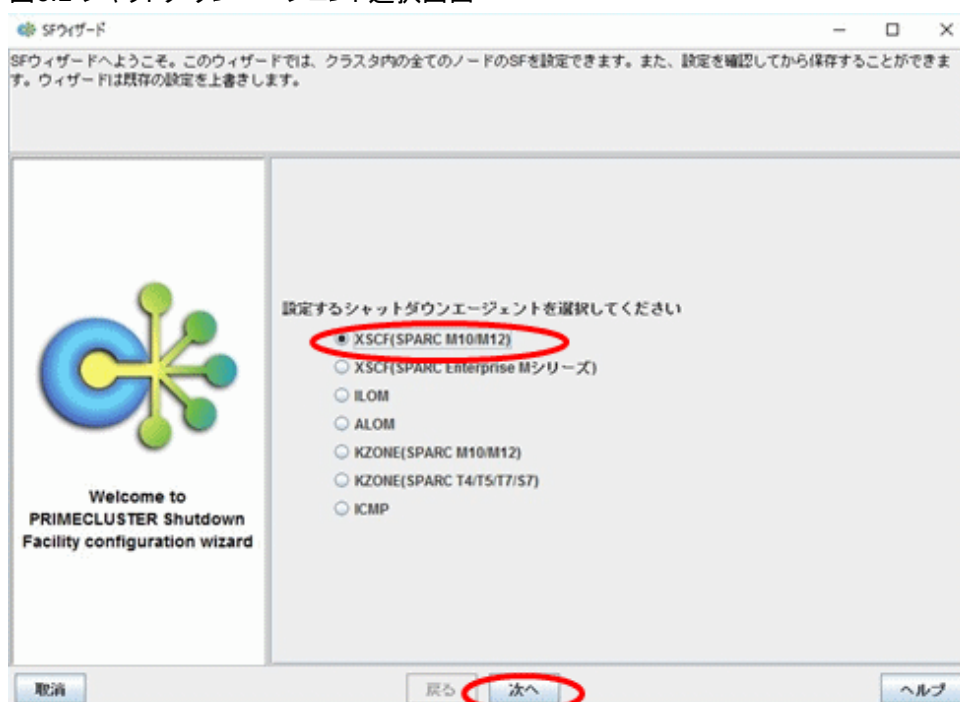
図6.1 シャットダウンエージェント選択画面
