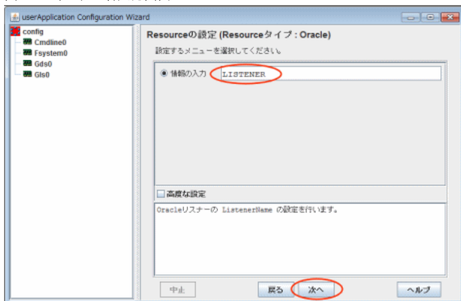
図14.53 リスナー名入力画面
