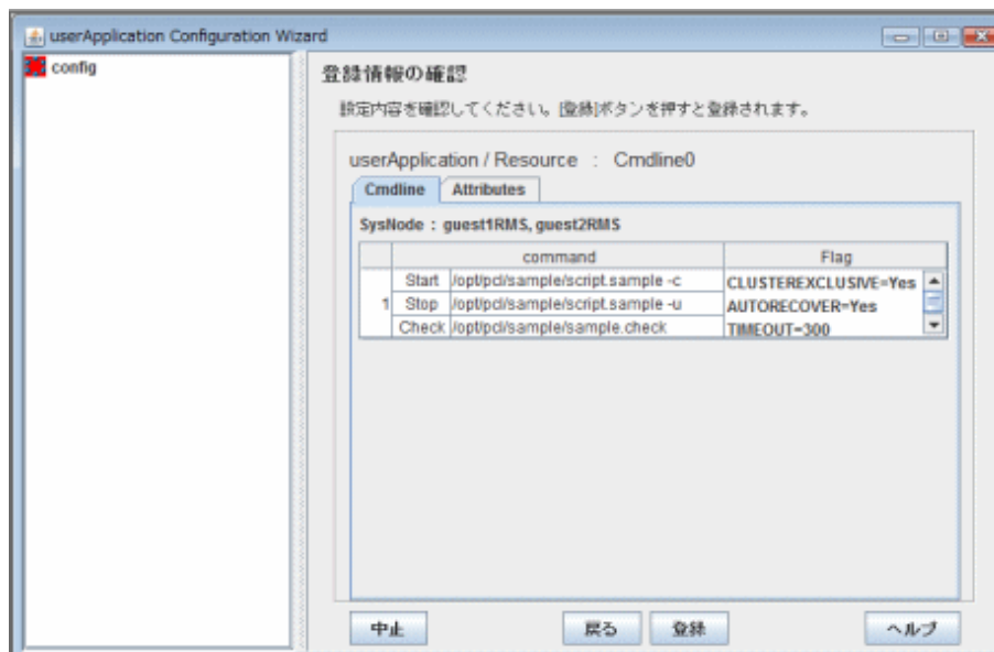
図14.23 “登録情報の確認”画面
