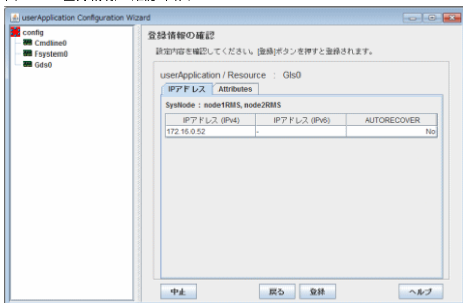
図14.42 “登録情報の確認”画面
