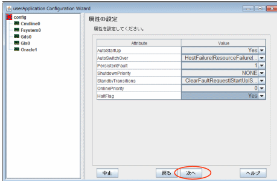
図14.60 “属性の設定”画面
