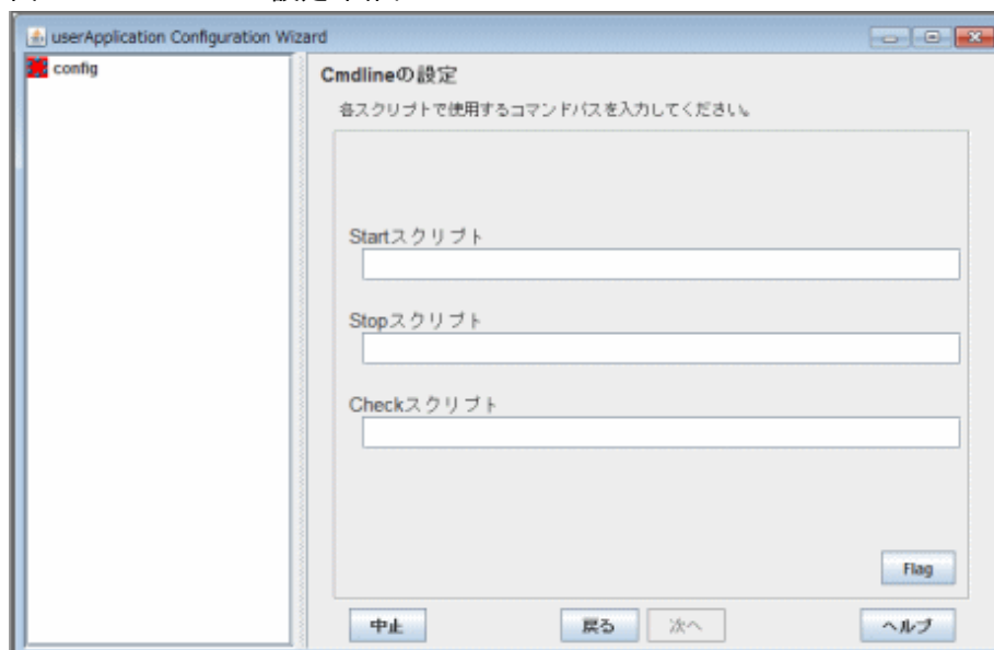
図14.21 “Cmdlineの設定”画面
