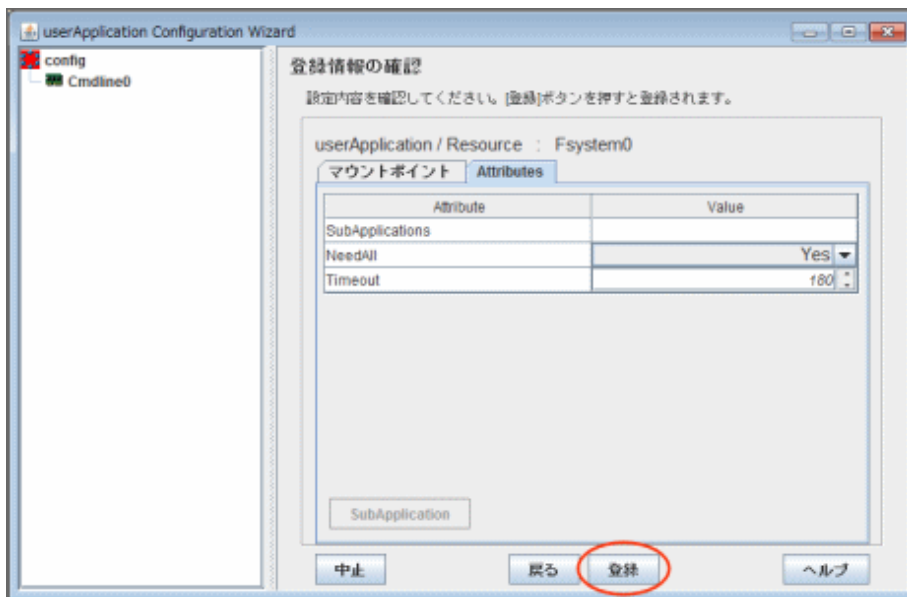
図14.30 設定内容登録確認画面
