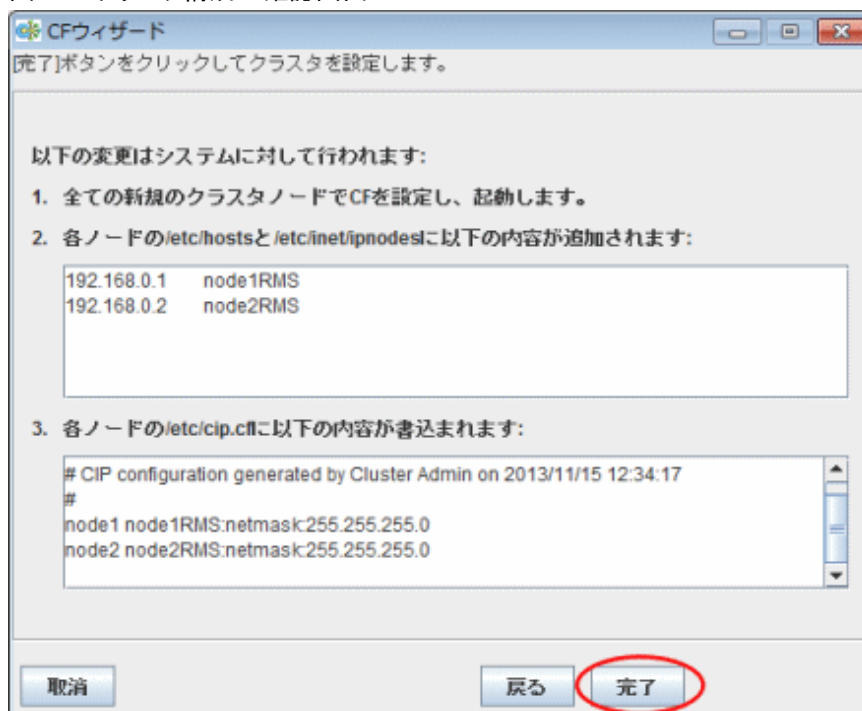
図5.14 クラスタ構成の確認画面
