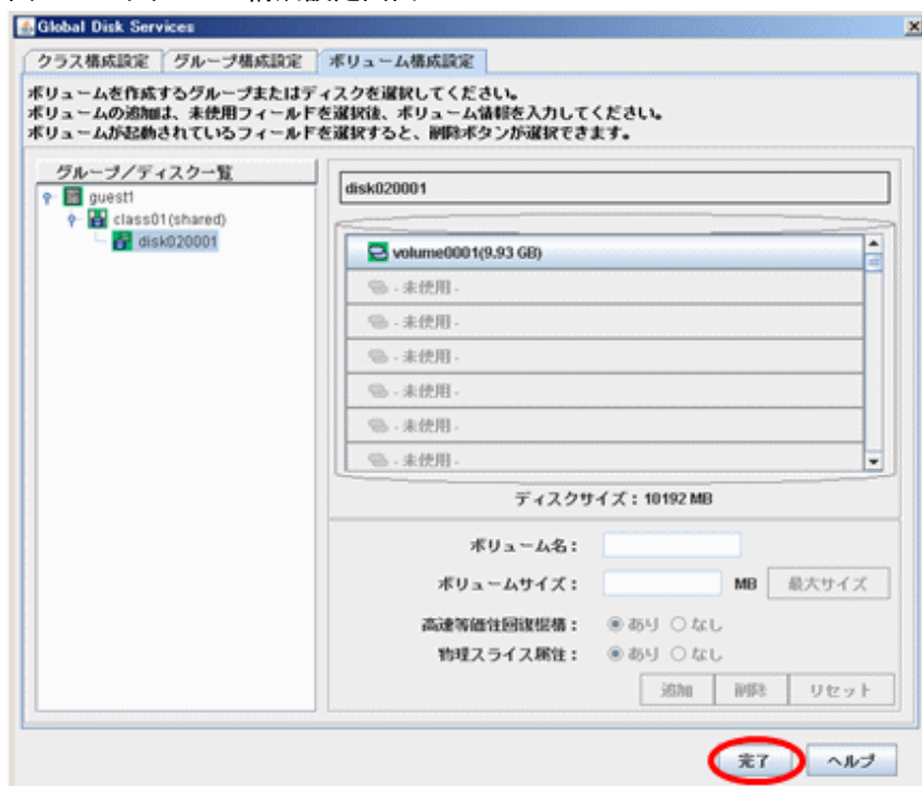
図14.13 ボリューム構成設定画面3
