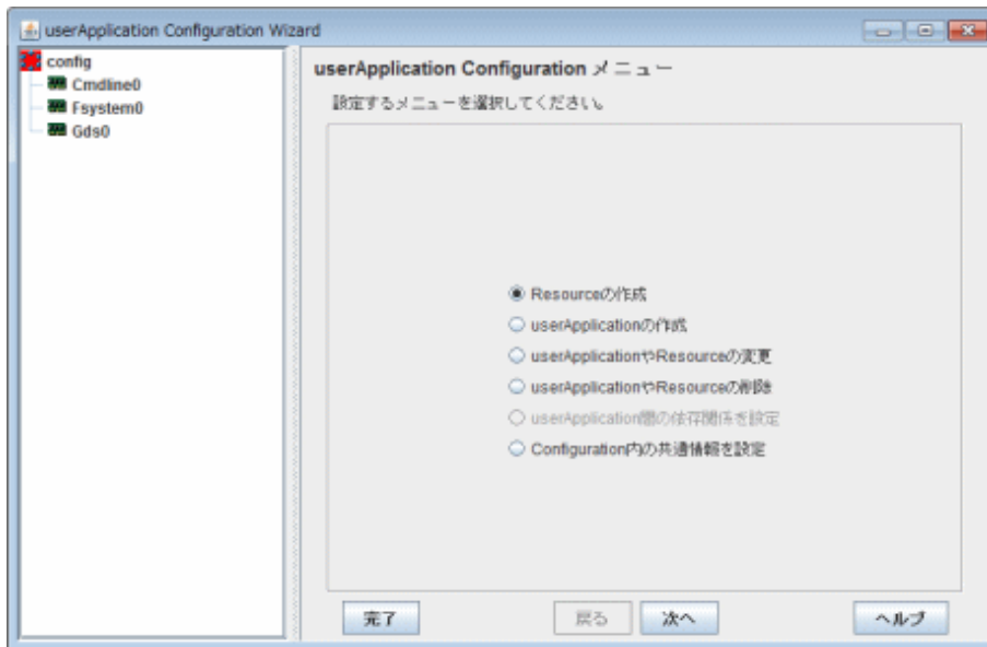
図14.38 リソース登録完了画面
