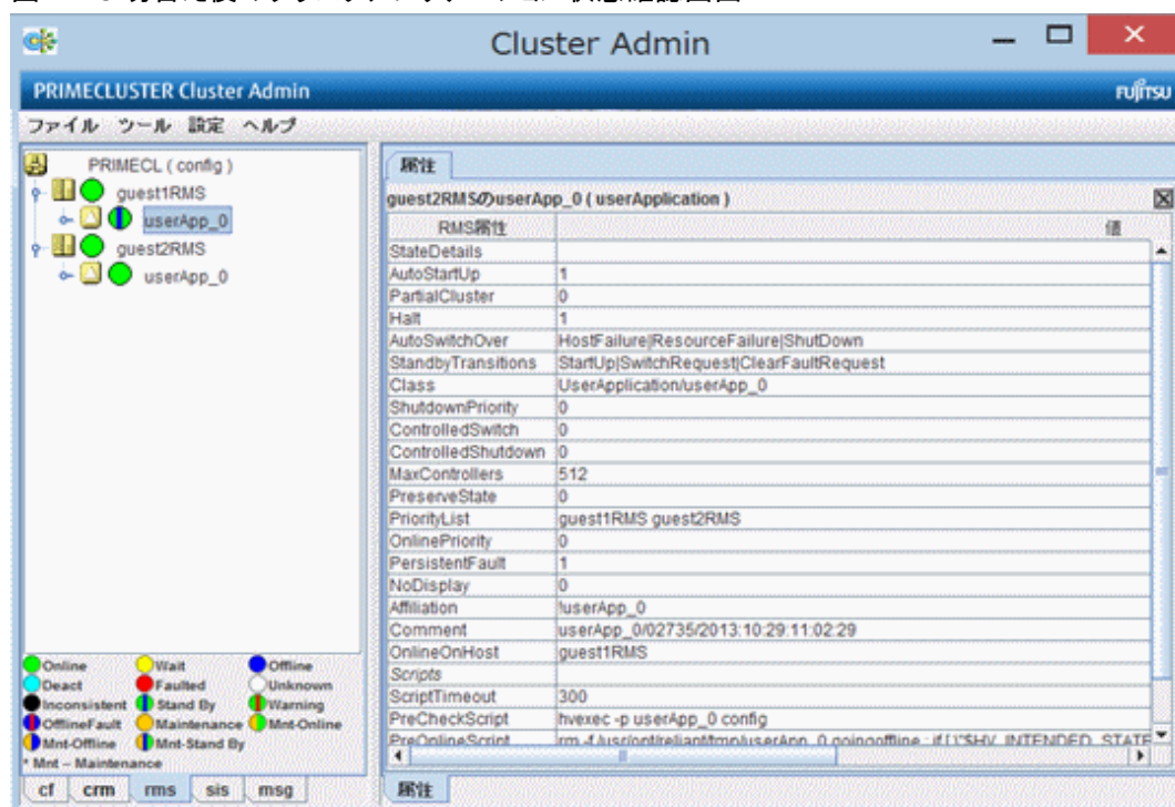
図14.78 切替え後のクラスタアプリケーション状態確認画面
