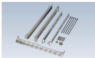
ラックマウントキット 製品型名: IX119RM1 標準価格: ¥30,000 備考: EX1100/1300用 ラック搭載用キット
