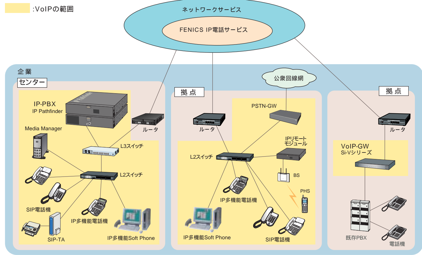
VoIP全体図
