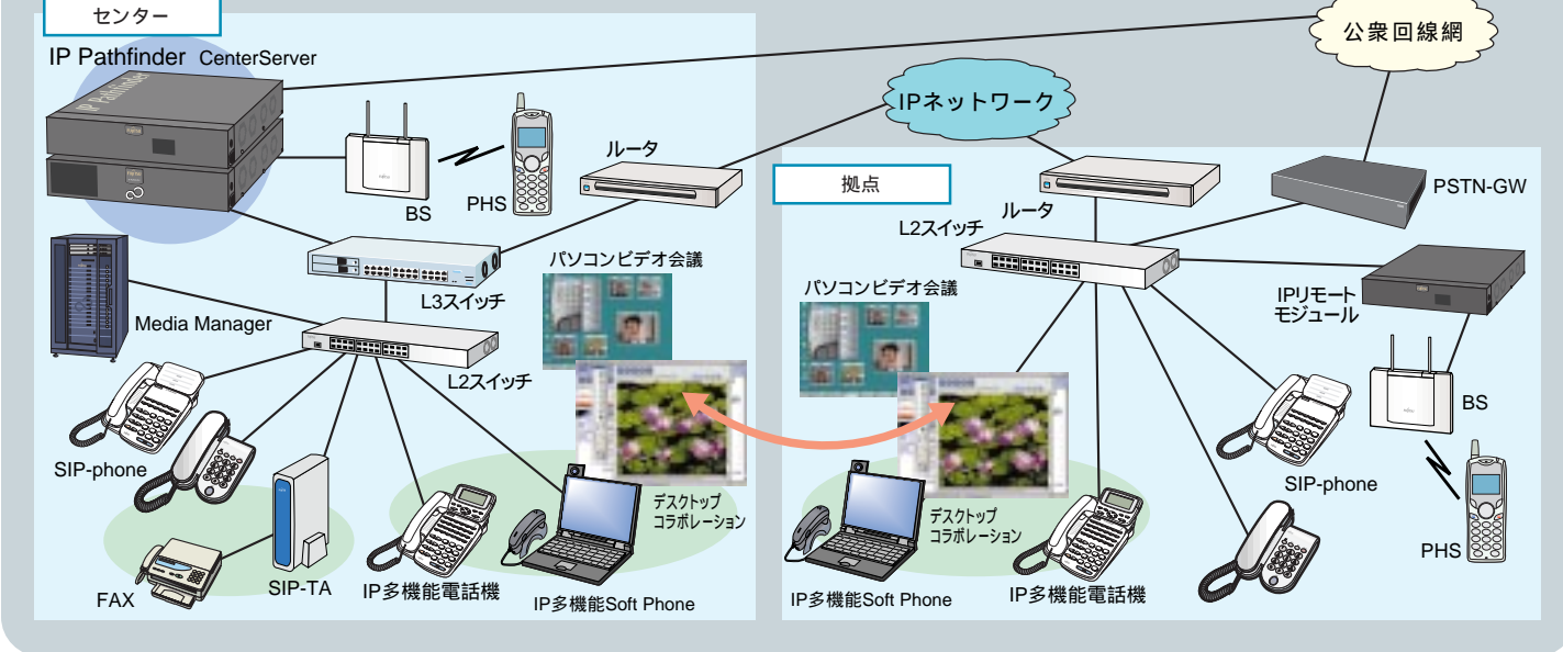
IP Pathfinderシステム構成図
