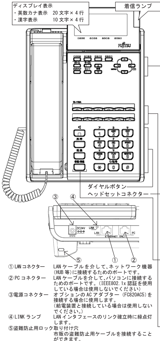
＜SS-190A2Wの外観図および各ボタンの説明＞
