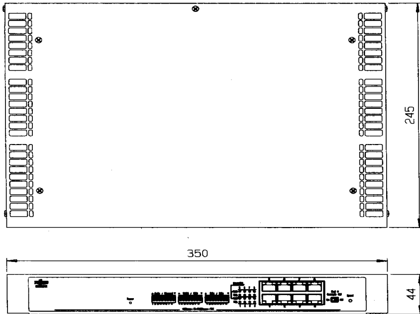
図 1-1 SH1511スイッチングハブ外觀図 (単位: mm)
