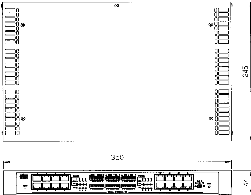
図 1-2 SH1531スイッチングハブ外觀図 (単位: mm)
