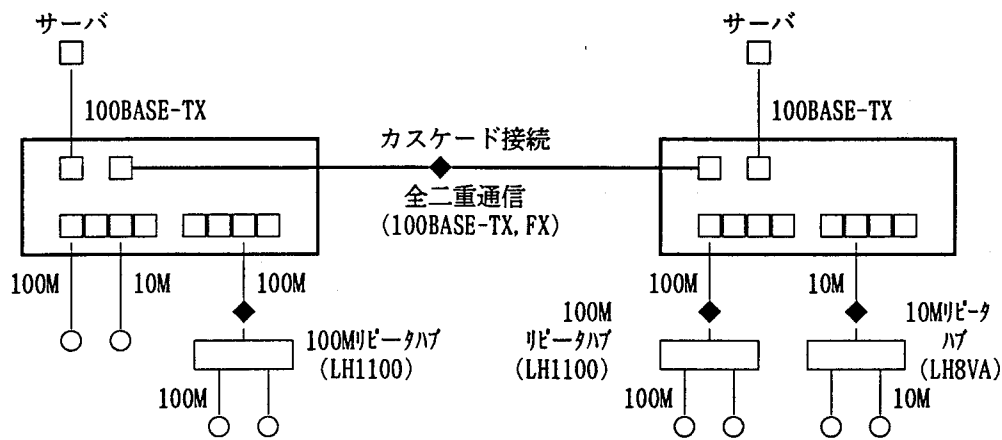
図3.2 中規模システムの運用形態
