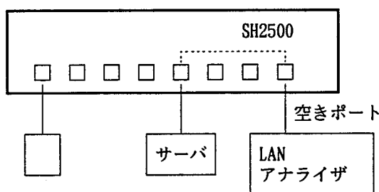
図2.6 ポートモニタリング機能
