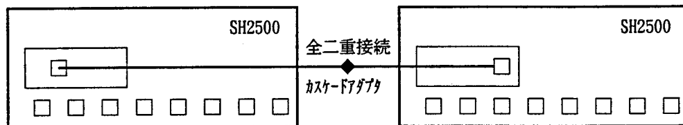
図2.5 全二重通信
