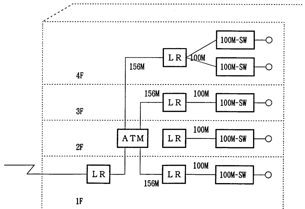
図3.3 大規模システムの運用形態
