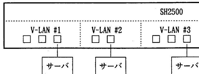
図2.2 SVLAN 機能
