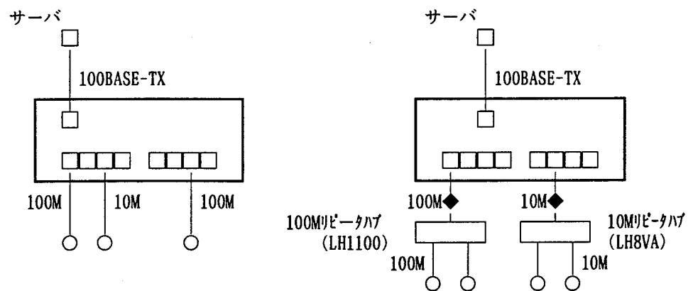
図3.1 小規模システムの運用形態
