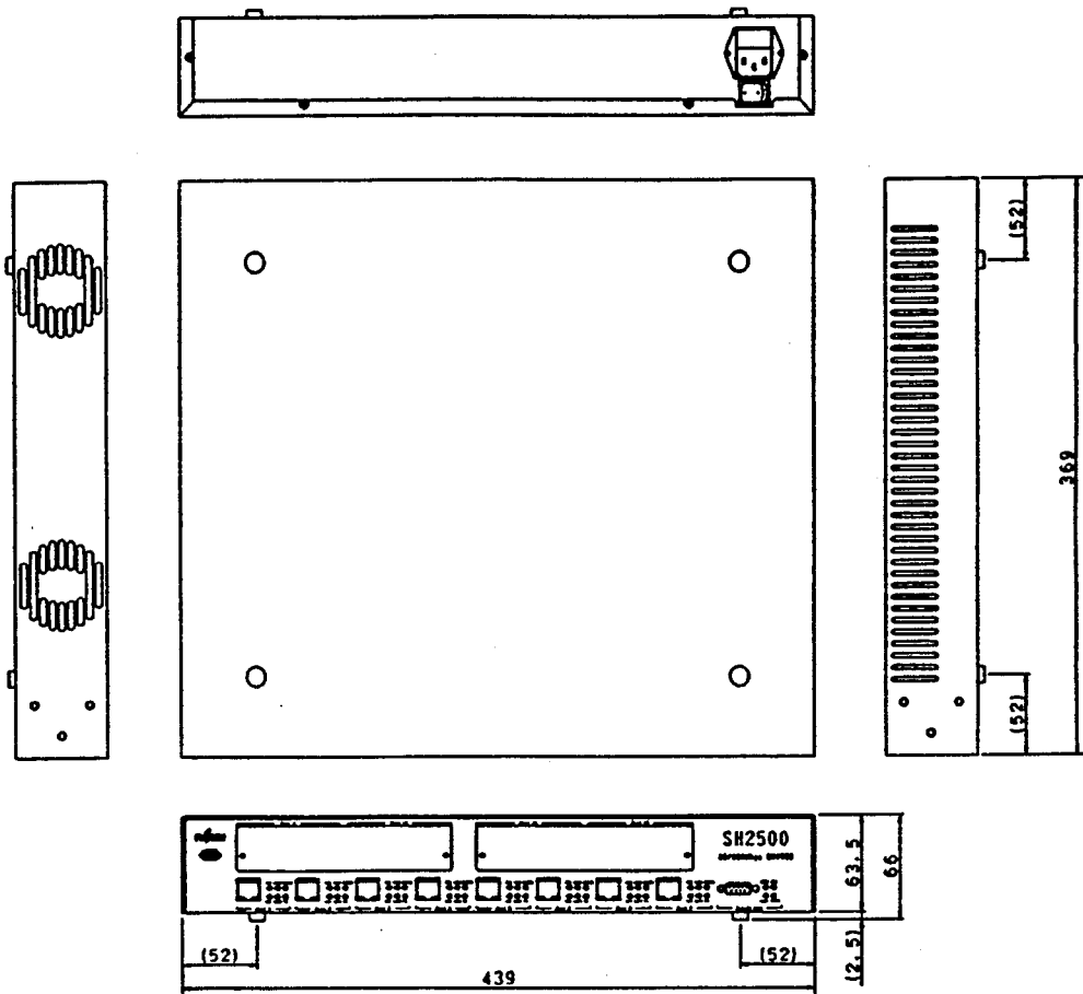
図1.1 装置の外観
