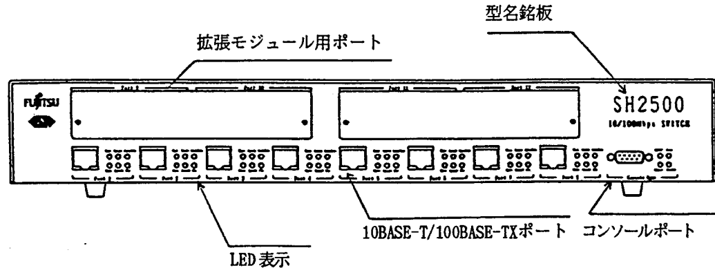
図1.2 装置前面
