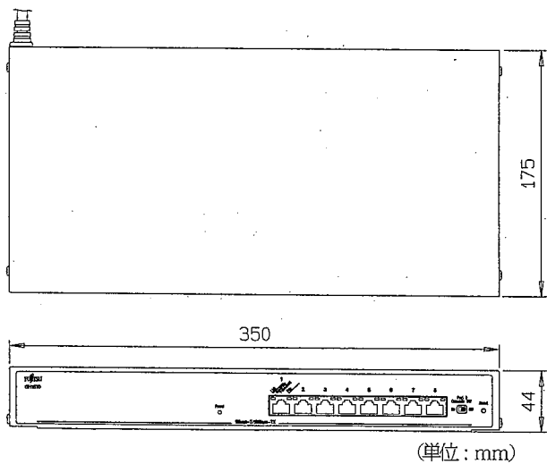
图1-1 SH1510外观图
