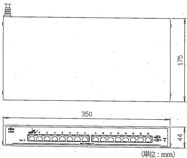
图1-2 SH1530外观图
