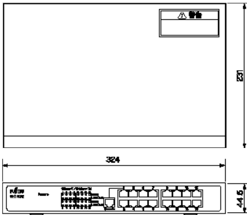
図 1-1 SH1532スイッチングハブ外觀図 (単位: mm)
