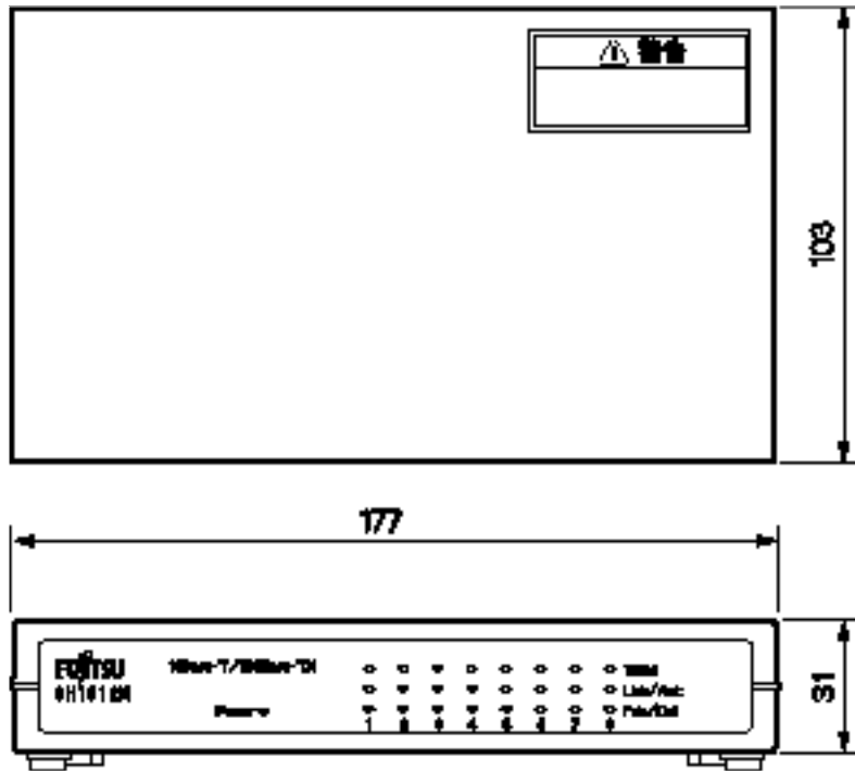
図 1-1 SH1512Mスイッチングハブ外觀図 (単位：mm)
