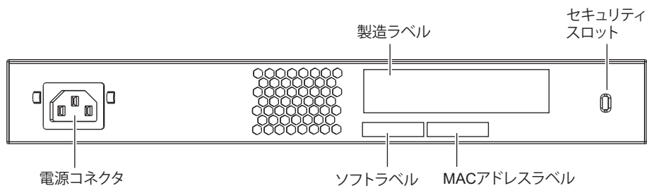
[SR-S318TL2の背面]
