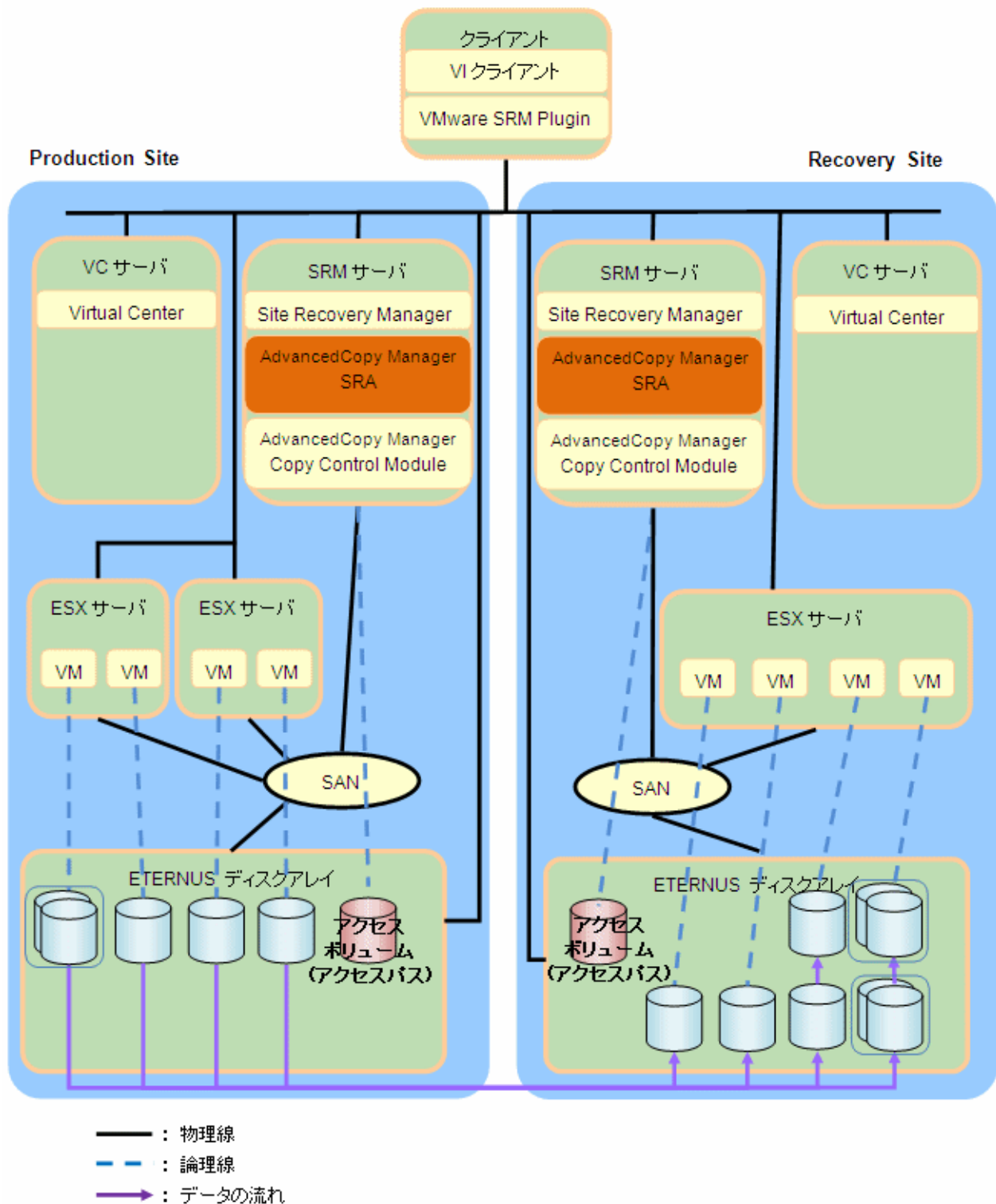
図1.6 AdvancedCopy Manager SRAのシステム構成例
