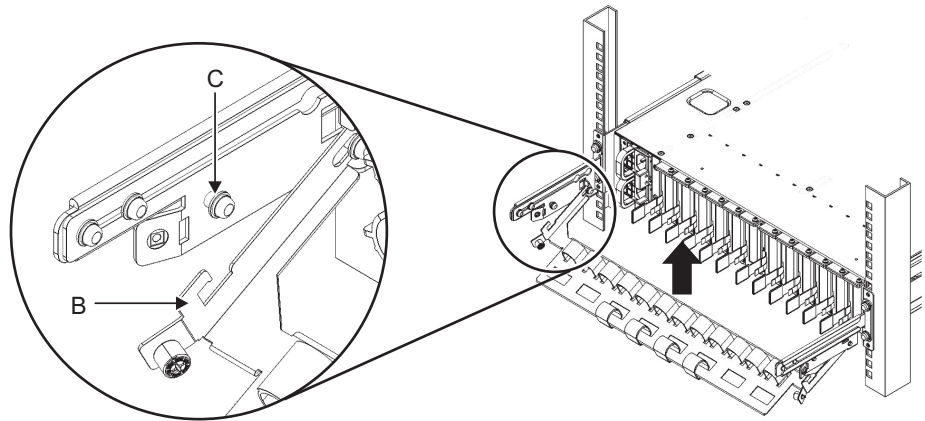
図 6-5 ケーブルサポートの操作
