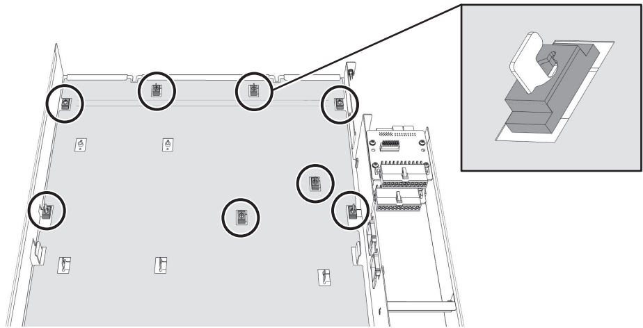
図 15-4 スペーサーの取り付け
