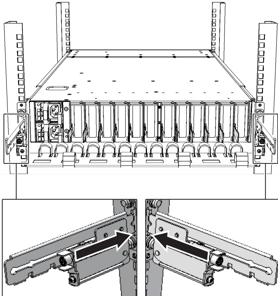
図 6-4 ケーブルサポートのロック
