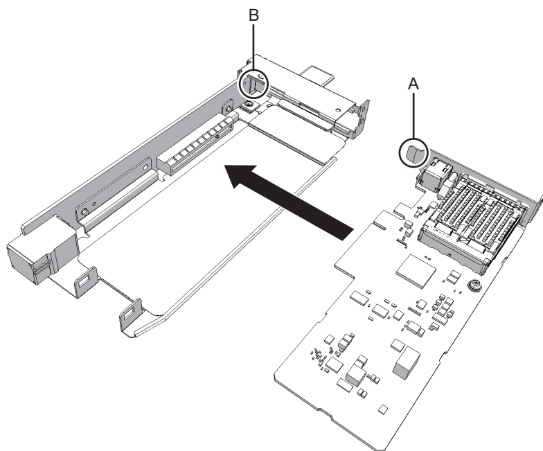
図 9-6 リンクボードの取り付け
