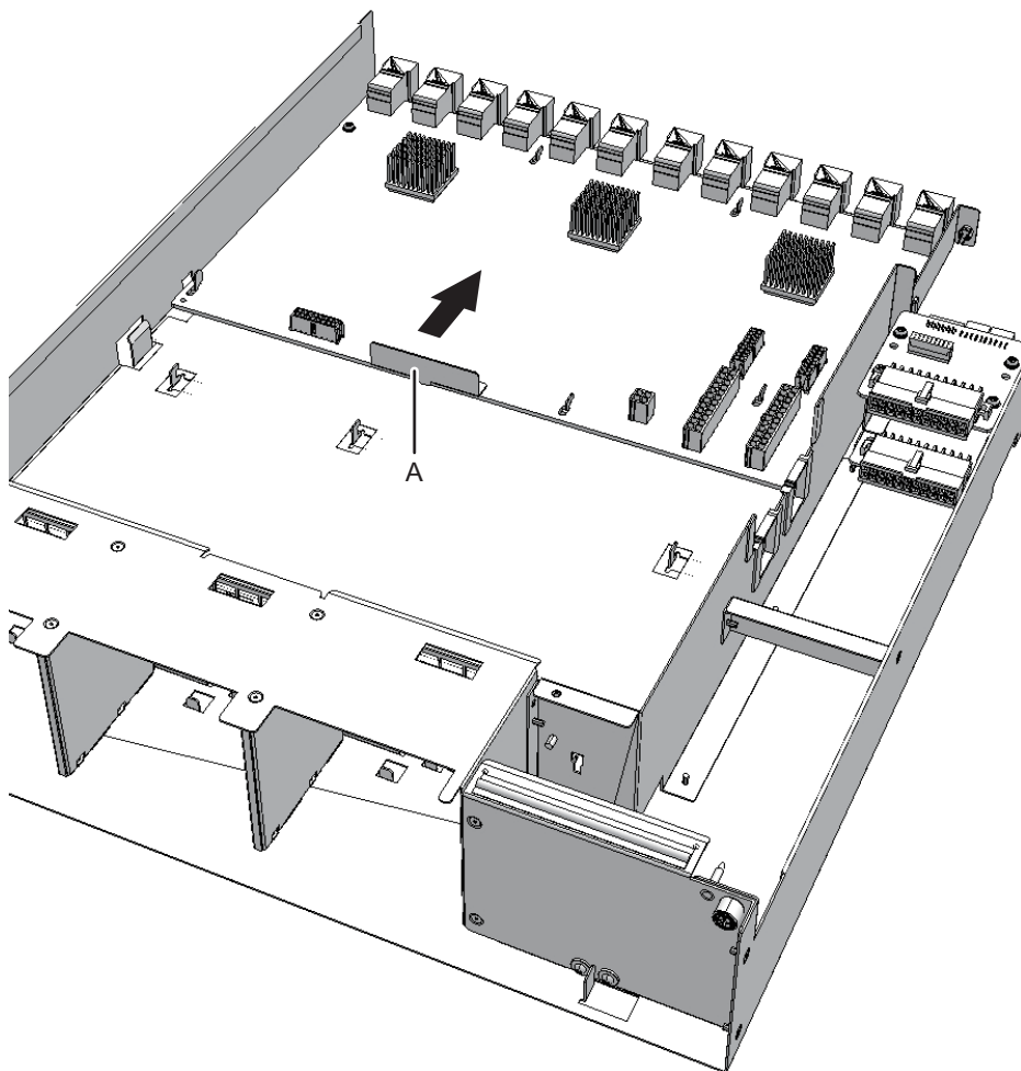
図 16-4 I/Oボードの取り外し
