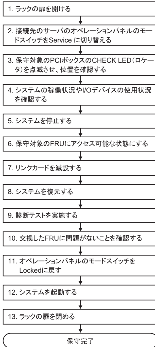
図 7-25 停止減設のながれ（システム停止によるリンクカードの減設）
