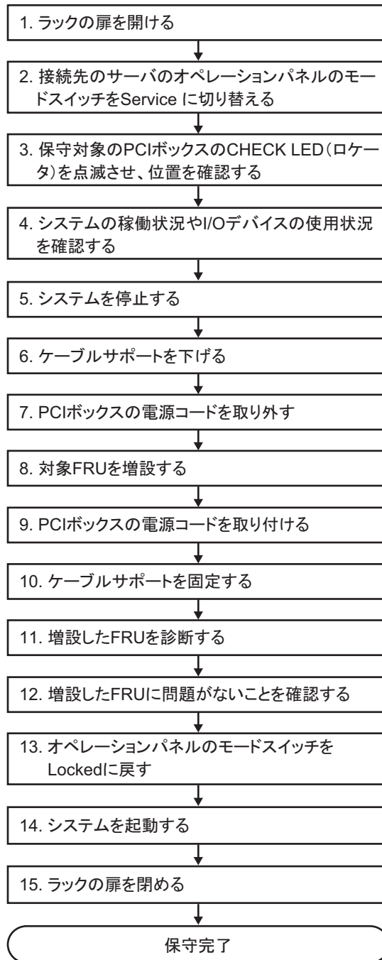
図 7-7 停電増設のながれ（システム停止によるリンクカードの切り離し）
