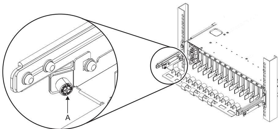
図 5-2 ケーブルサポートのねじの位置
