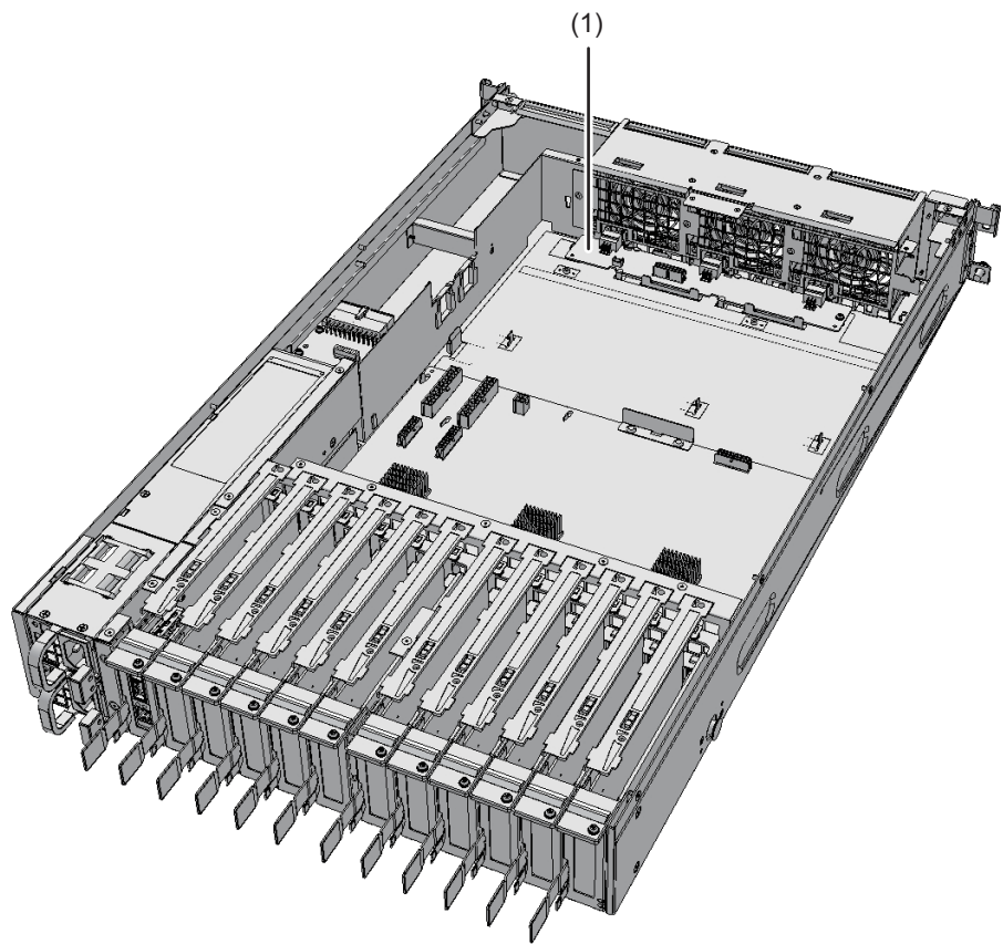
図 17-1 ファンバックプレーンの位置
