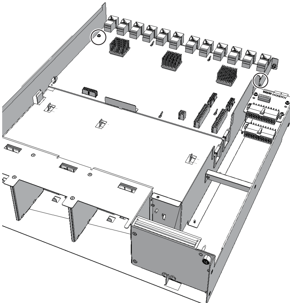
図 16-6 I/Oボードのねじ
