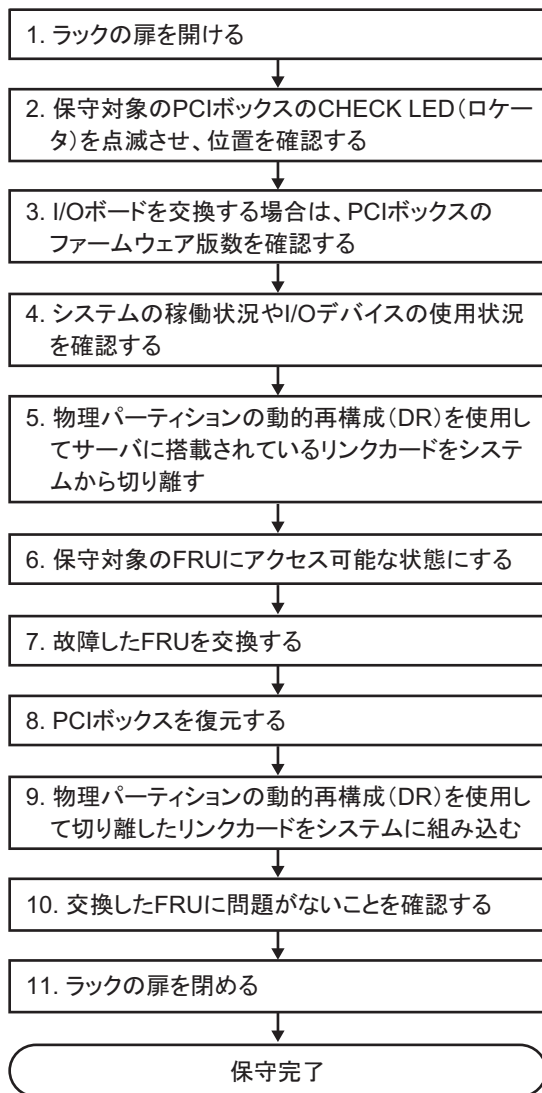
図 7-5 停電交換のながれ（DRによるリンクカードの切り離し）
