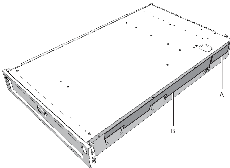
図 1-1 システム銘板ラベル／規格ラベルの位置
