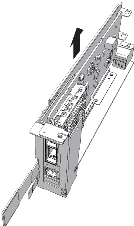
図 9-5 リンクボードの取り外し
