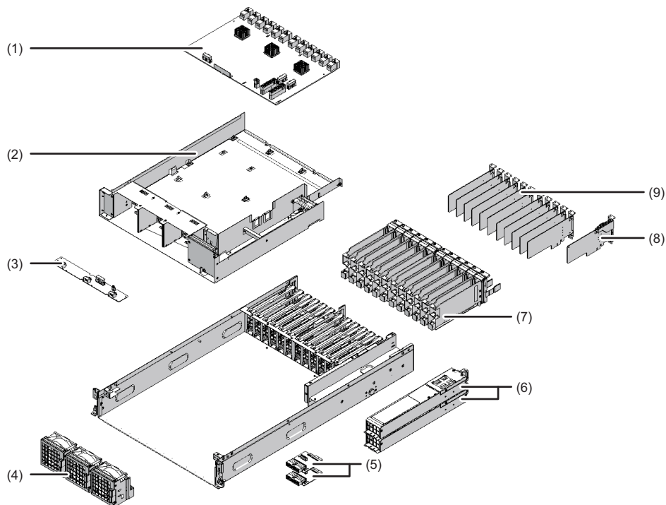
図 A-1 コンポーネントの位置
