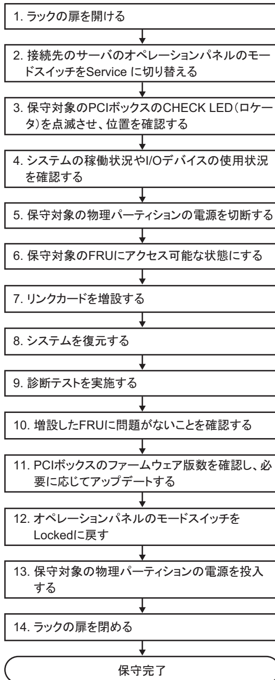
図 7-21 非活性増設のながれ（物理パーティション停止によるリンクカードの増設）
