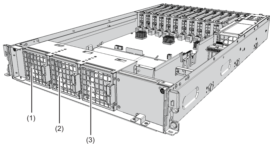
図 14-1 ファンユニットの位置
