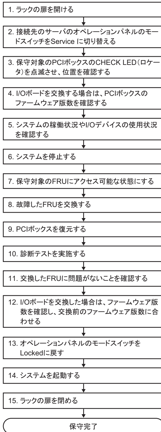
図 7-3 停電交換のながれ（システム停止によるリンクカードの切り離し）
