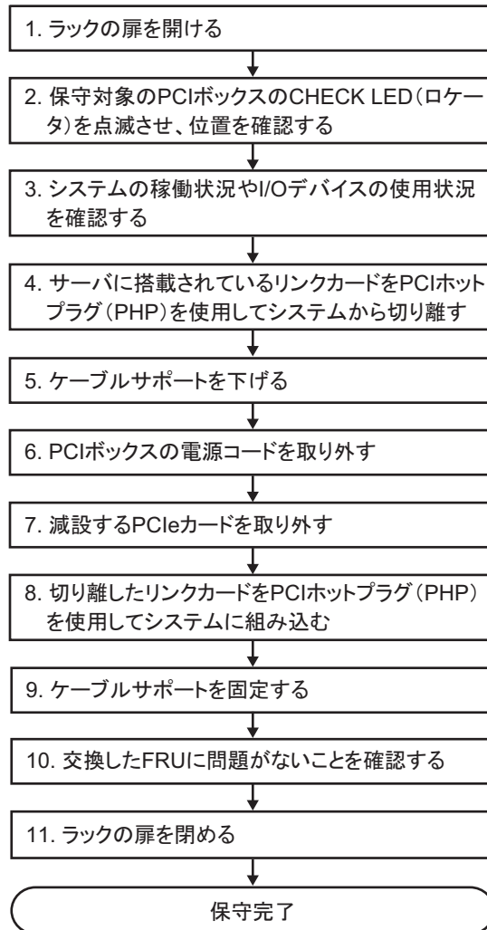
図 7-12 停電減設のながれ（PHPによるリンクカードの切り離し）
