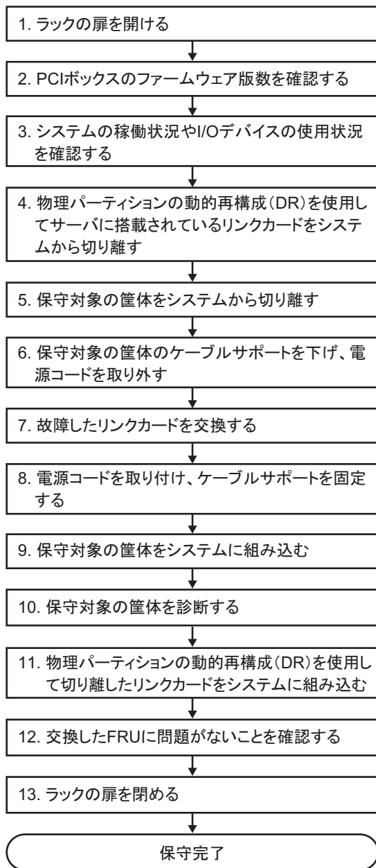
図 7-15 活性交換のながれ（DRによるリンクカードの交換の場合）
