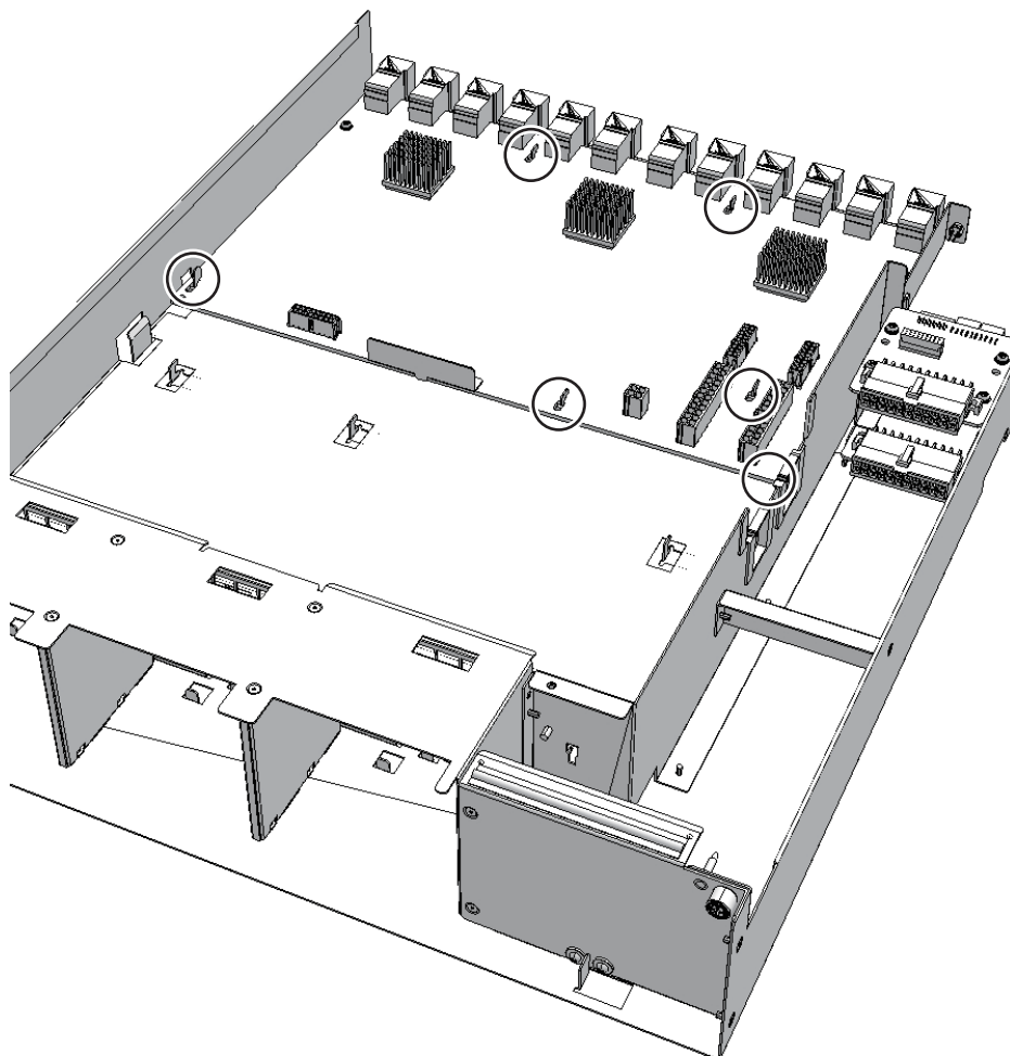
図 16-5 I/Oボードのつめ
