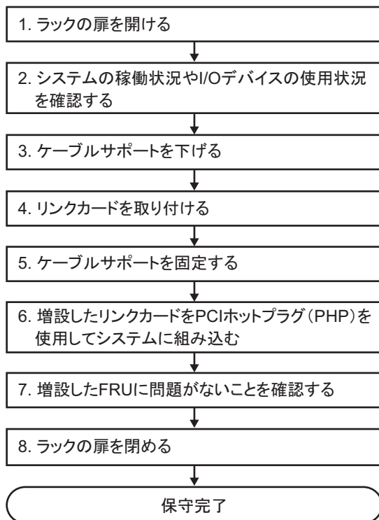
図 7-16 活性増設のながれ（PHPによるリンクカードの増設の場合）
