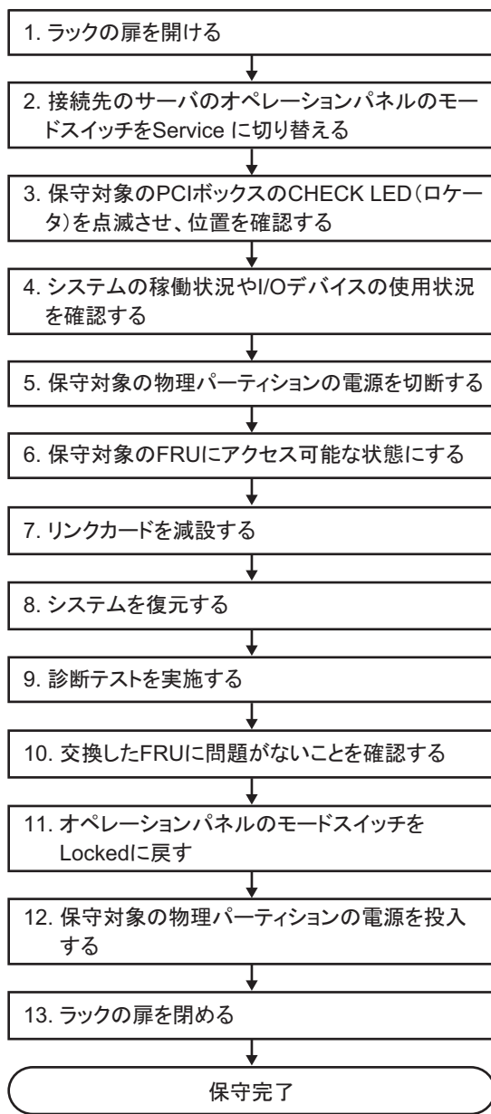
図 7-22 非活性減設のながれ（物理パーティション停止によるリンクカードの減設）
