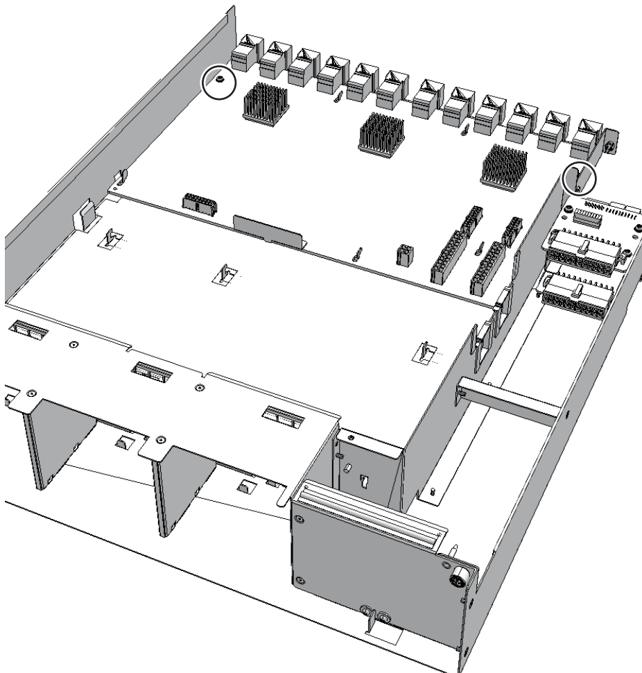
図 16-3 I/Oボードのねじ
