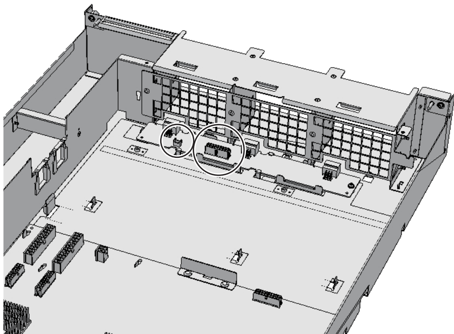
図 17-7 ファンバックプレーンのケーブル
