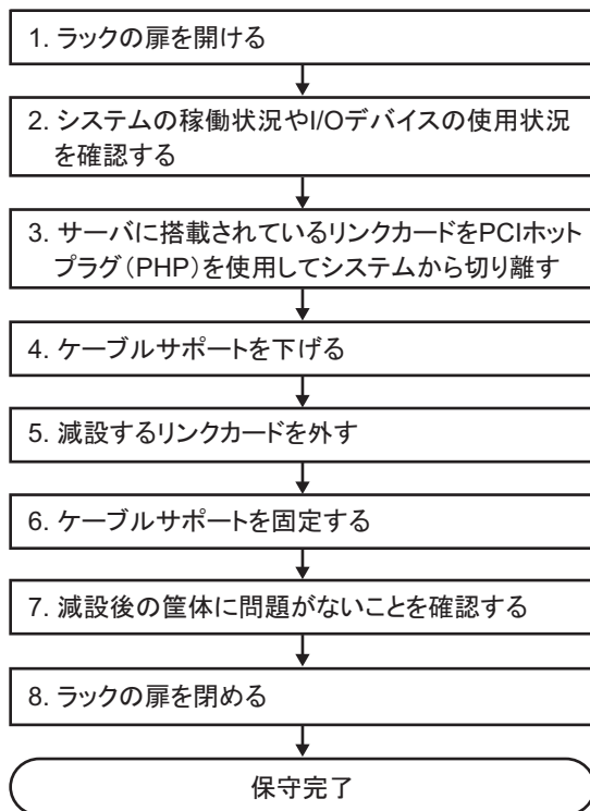
図 7-18 活性減設のながれ（PHPによるリンクカードの減設の場合）
