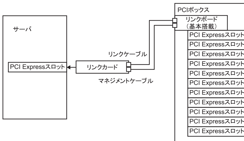
図 2-3 接続例
