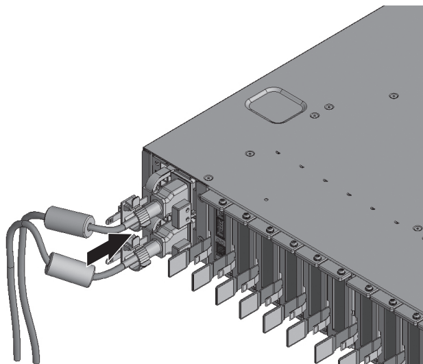
図 6-2 電源コードの取り付け
