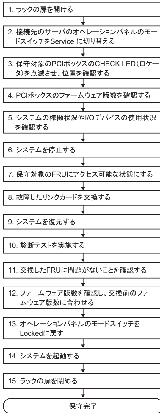
図 7-23 停止交換のながれ（システム停止によるリンクカードの交換）
