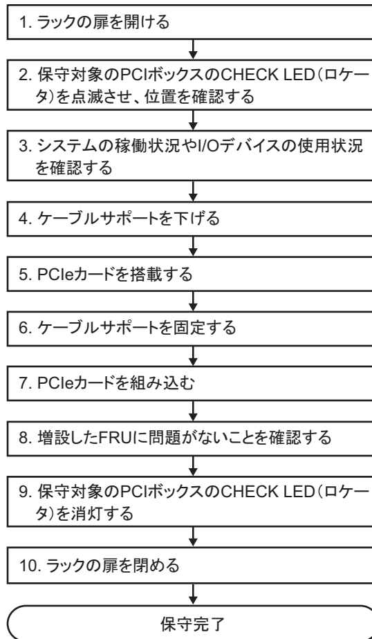
図 7-6 通電増設のながれ（PCI Expressカードの場合）
