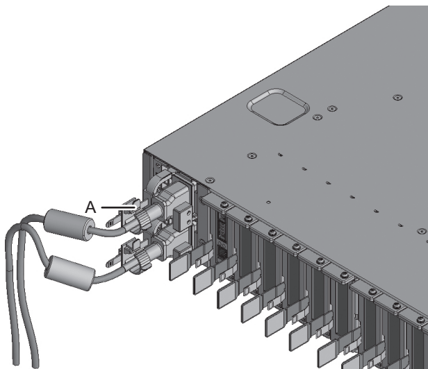
図 6-3 ケーブルクランプのロック
