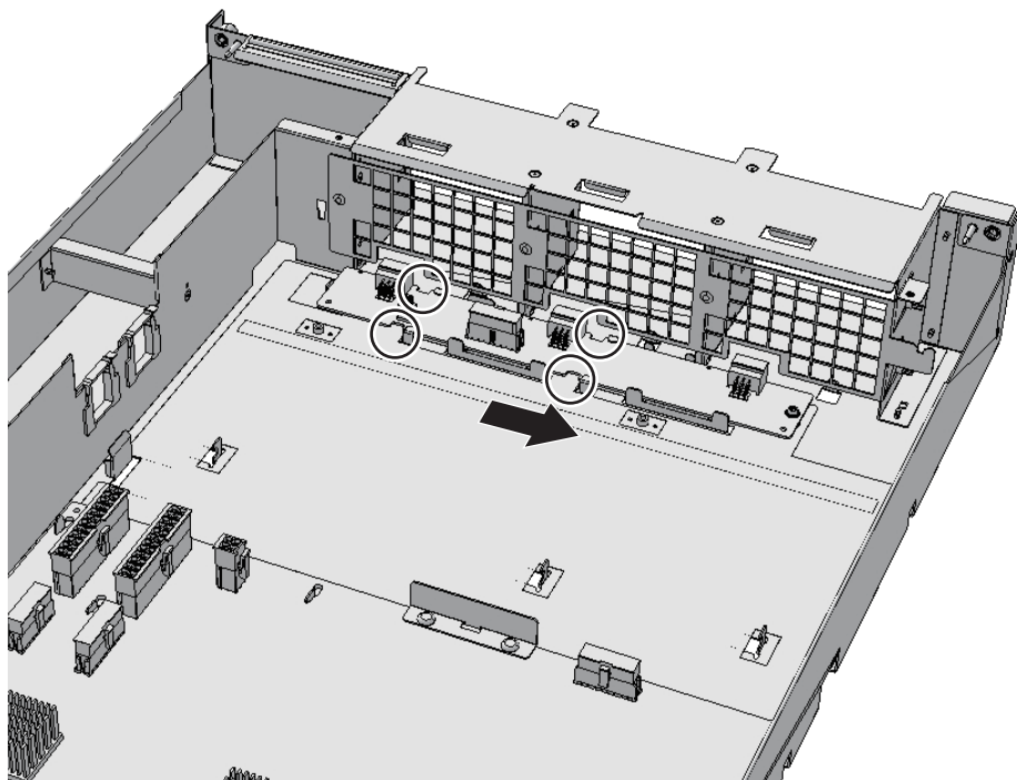
図 17-4 ファンバックプレーンの取り外し
