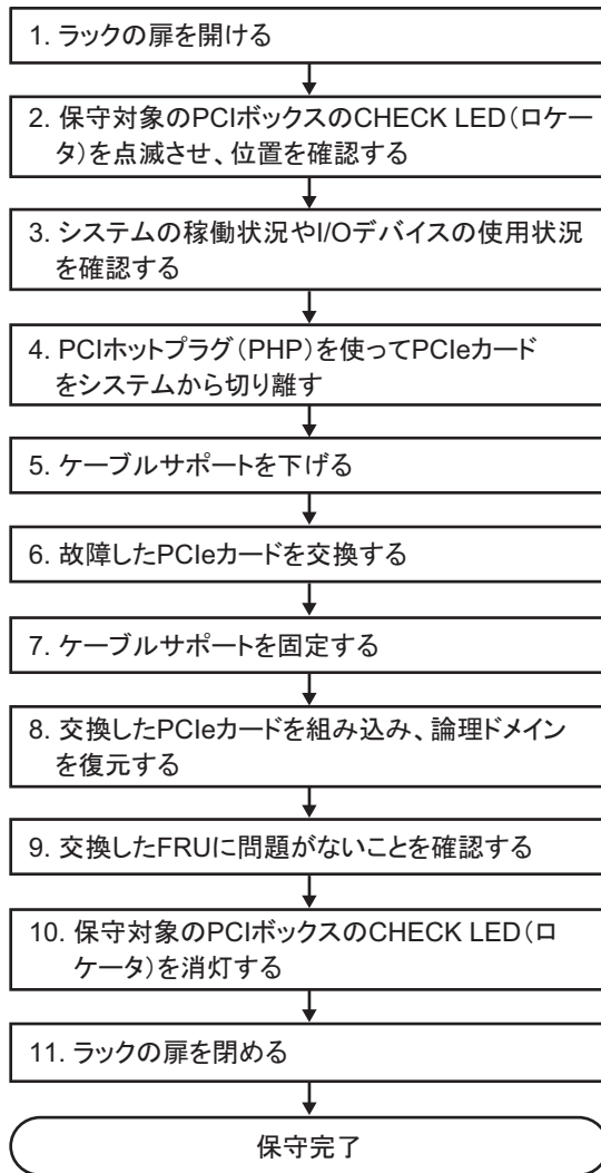
図 7-1 通電交換のながれ (PCI Expressカードの場合)
