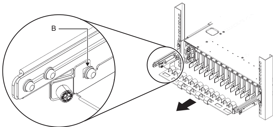
図 5-3 ケーブルサポートの解除
