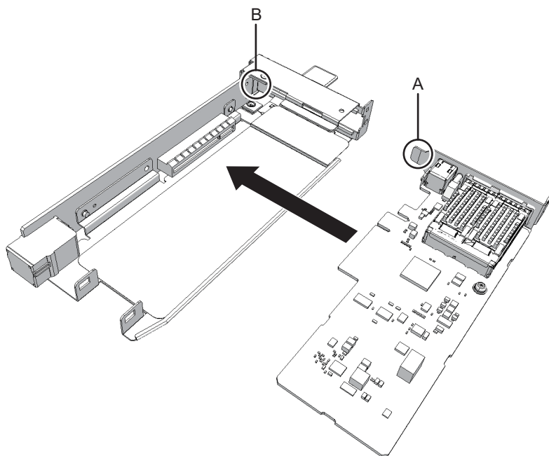
図 8-8 PCIeカードの取り付け
