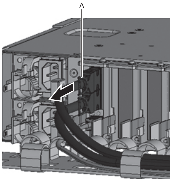
図 9-2 リンクケーブルの取り外し
