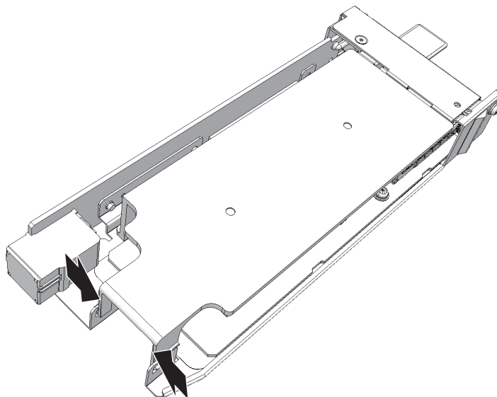
図 9-3 カバーのつめ
