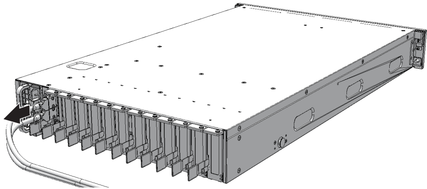
図 11-2 リンクケーブルの取り外し
