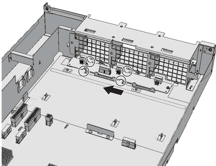
図 17-5 ファンバックプレーンの取り付け
