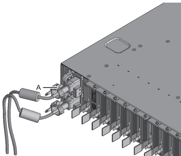
図 5-5 ケーブルクランプの解除
