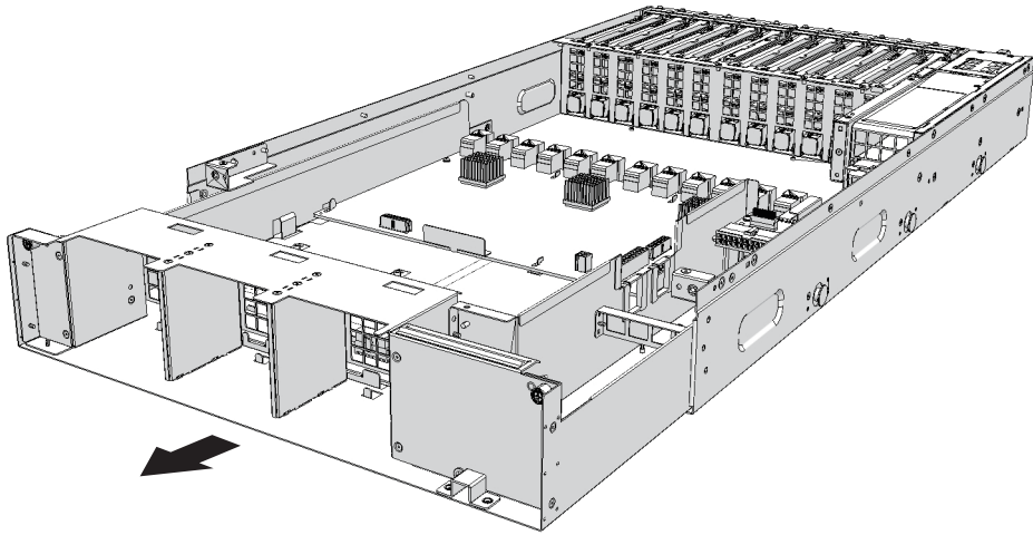
図 15-3 PCIトレイの取り外し
