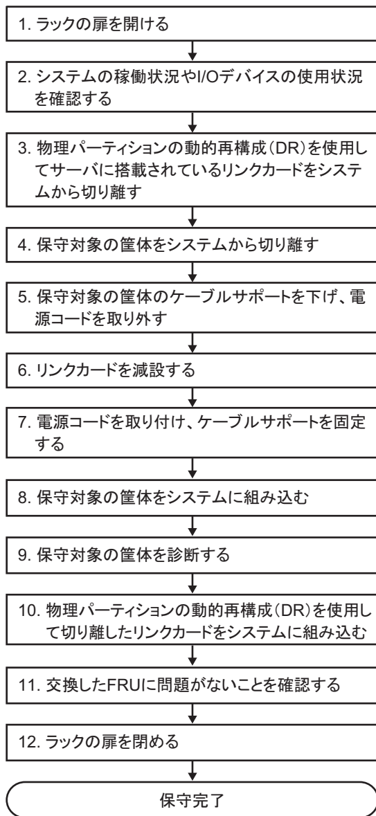
図 7-19 活性交換のながれ（DRによるリンクカードの交換の場合）
