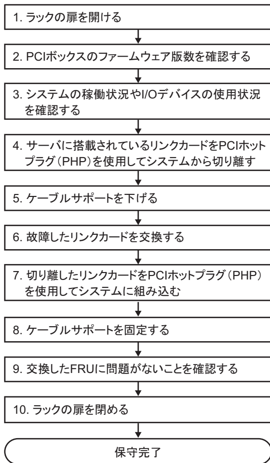
図 7-14 活性交換のながれ（PHPによるリンクカードの交換の場合）
