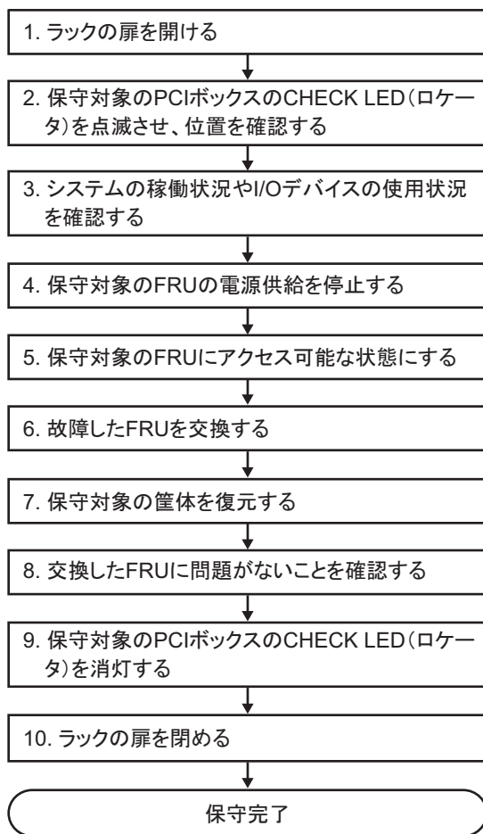
図 7-2 通電交換のながれ（電源ユニット、ファンユニットの場合）
