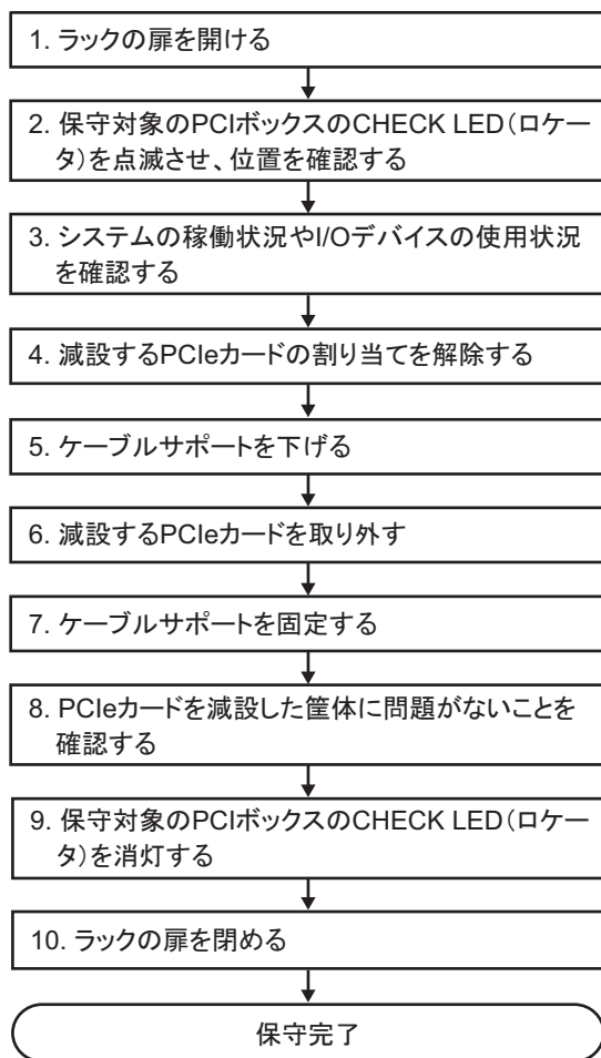
図 7-10 通電減設のながれ（PCI Expressカードの場合）
