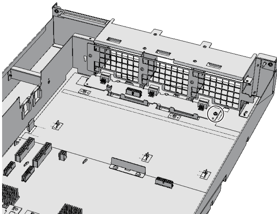
図 17-6 ファンバックプレーンのねじ
