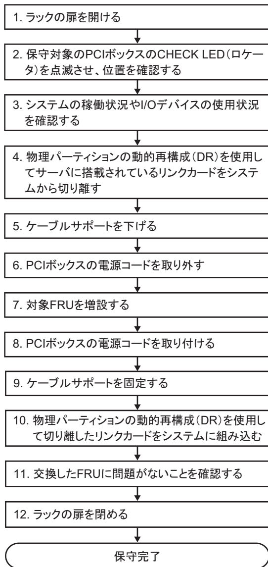
図 7-9 停電増設のながれ（DRによるリンクカードの切り離し）
