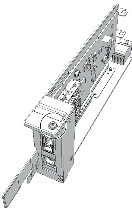
図 9-4 金具の取り外し
