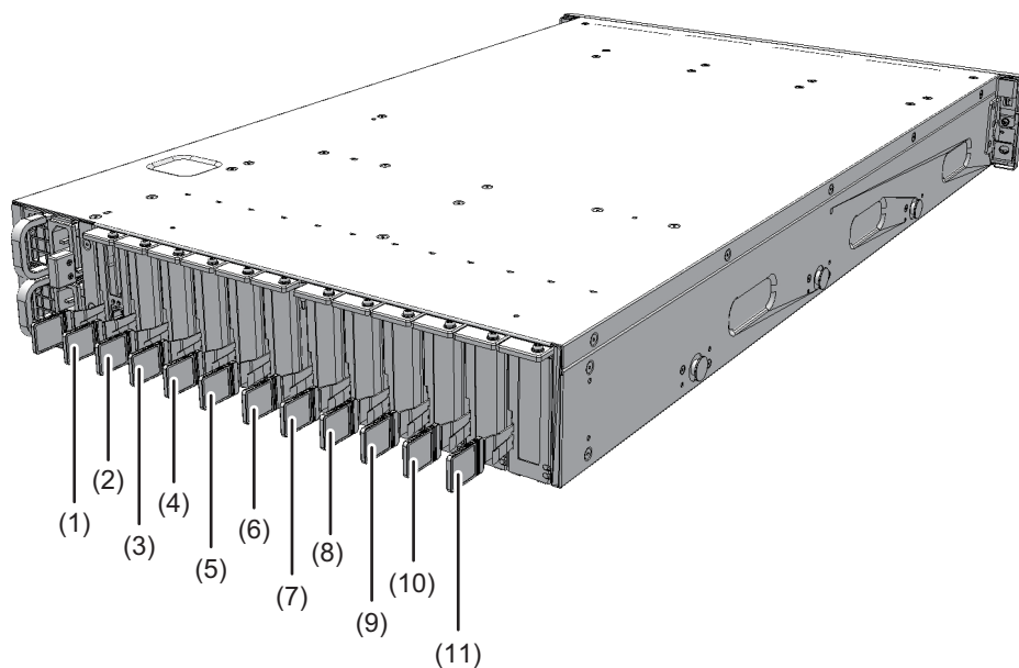
図 8-1 PCIeカードの位置
