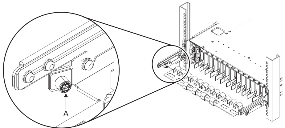
図 6-6 ケーブルサポートのロック
