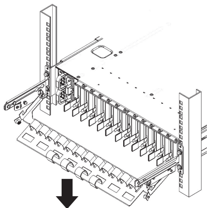
図 5-4 ケーブルサポートの操作
