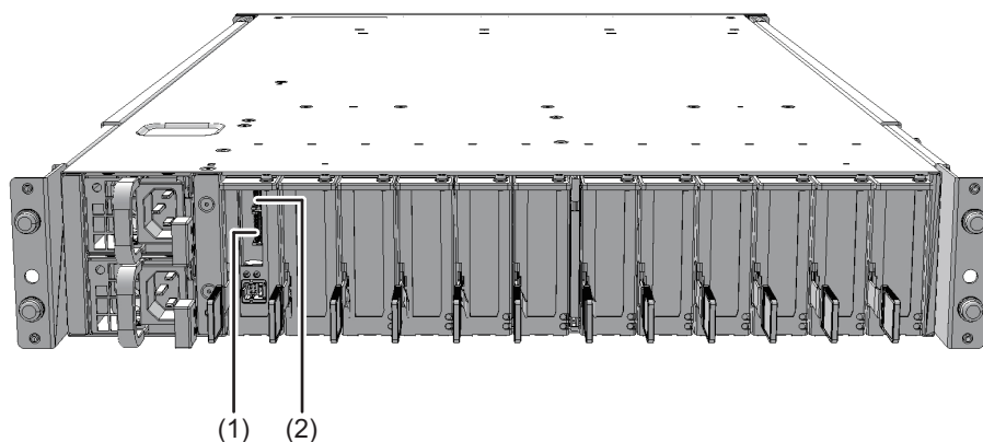
図 11-1 リンクケーブル接続ポートの位置
