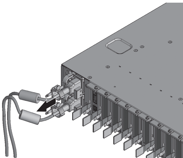
図 5-6 電源コードの取り外し
