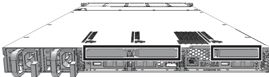
図 10-3 リンクカードの搭載位置 (SPARC M10-1)
