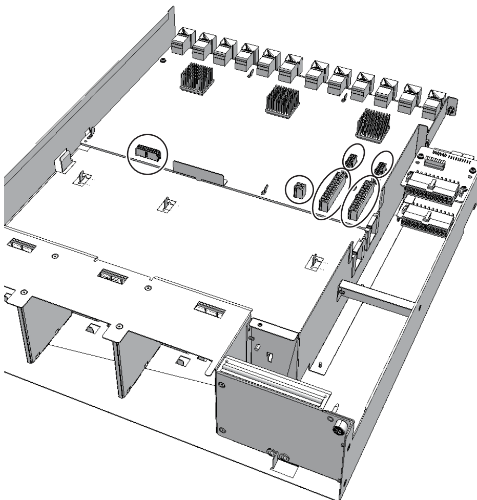
図 16-2 I/Oボードのケーブル
