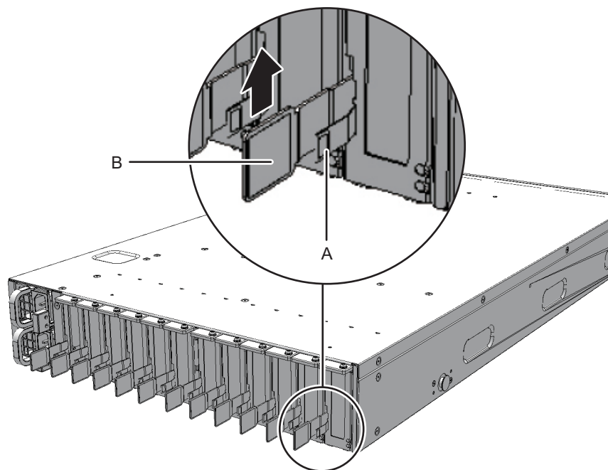
図 8-3 PCIeカードカセットのラッチとレバー
