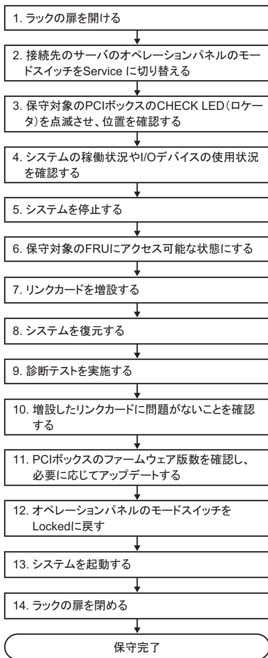
図 7-24 停止増設のながれ（システム停止によるリンクカードの増設）
