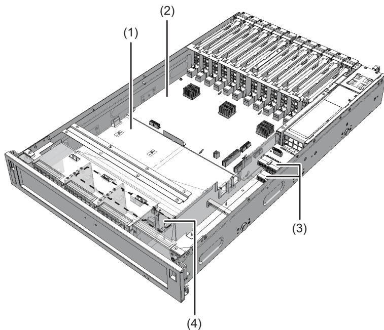
図 2-4 内部コンポーネントの位置
