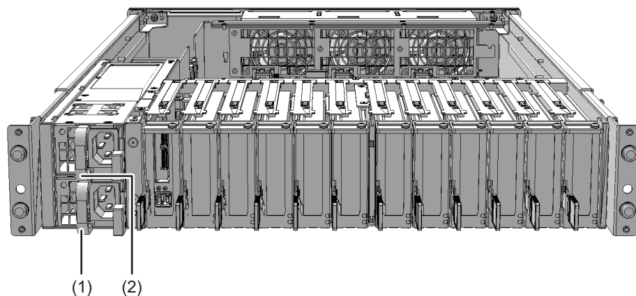
図 13-1 電源ユニットの位置
