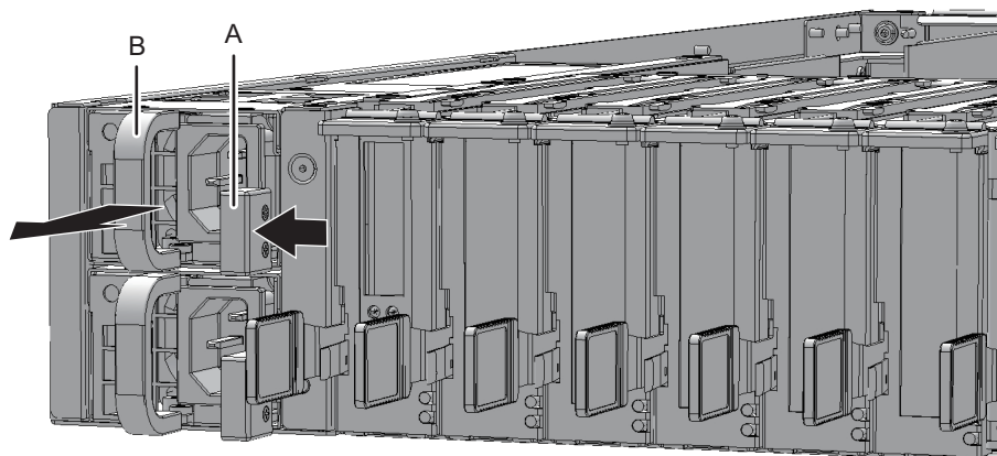
図 13-2 電源ユニットの取り外し
