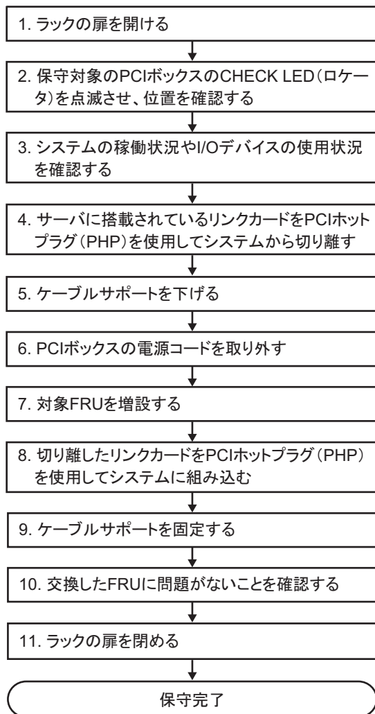
図 7-8 停電増設のながれ（PHPによるリンクカードの切り離し）
