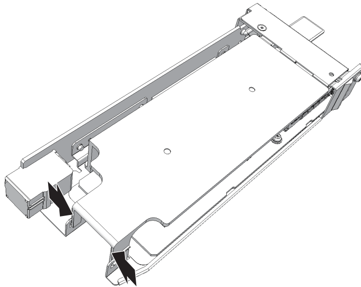
図 8-5 カバーのつめ
