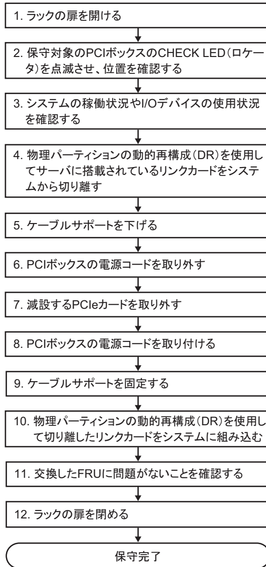
図 7-13 停電減設のながれ（DRによるリンクカードの切り離し）
