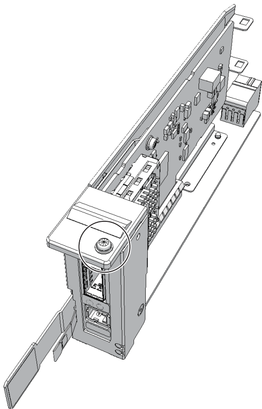
図 8-9 金具の取り付け
