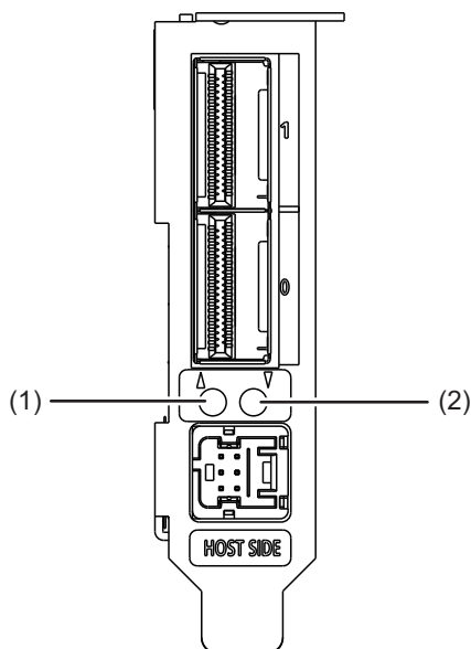
図 2-7 リンクカードのLED
