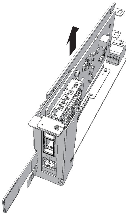
図 8-7 PCIeカードの取り外し
