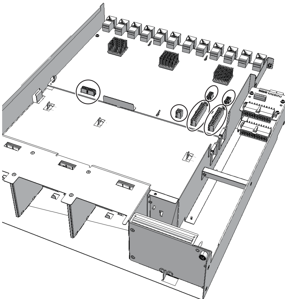
図 16-7 I/Oボードのケーブル
