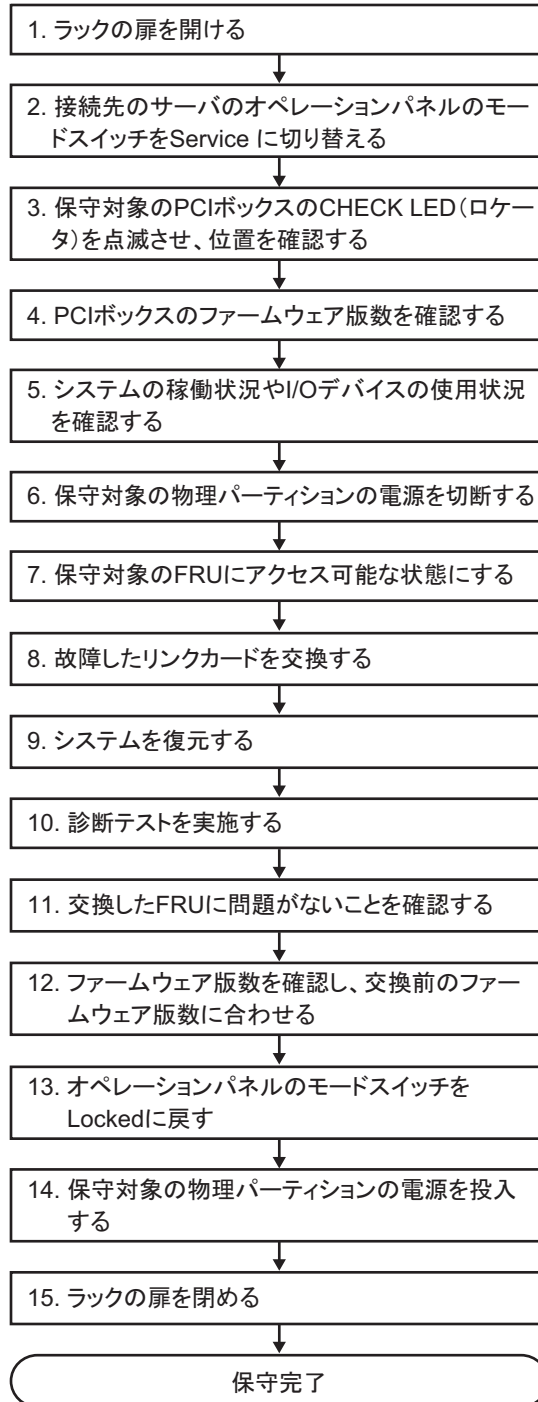
図 7-20 非活性交換のながれ（物理パーティション停止によるリンクカードの交換）
