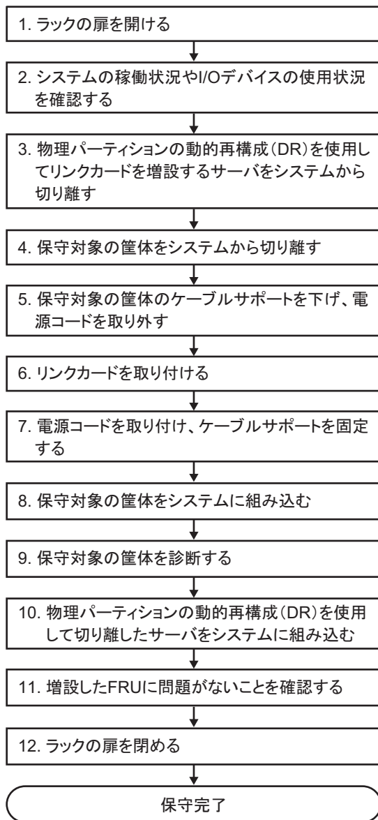
図 7-17 活性増設のながれ（DRによるリンクカードの増設の場合）
