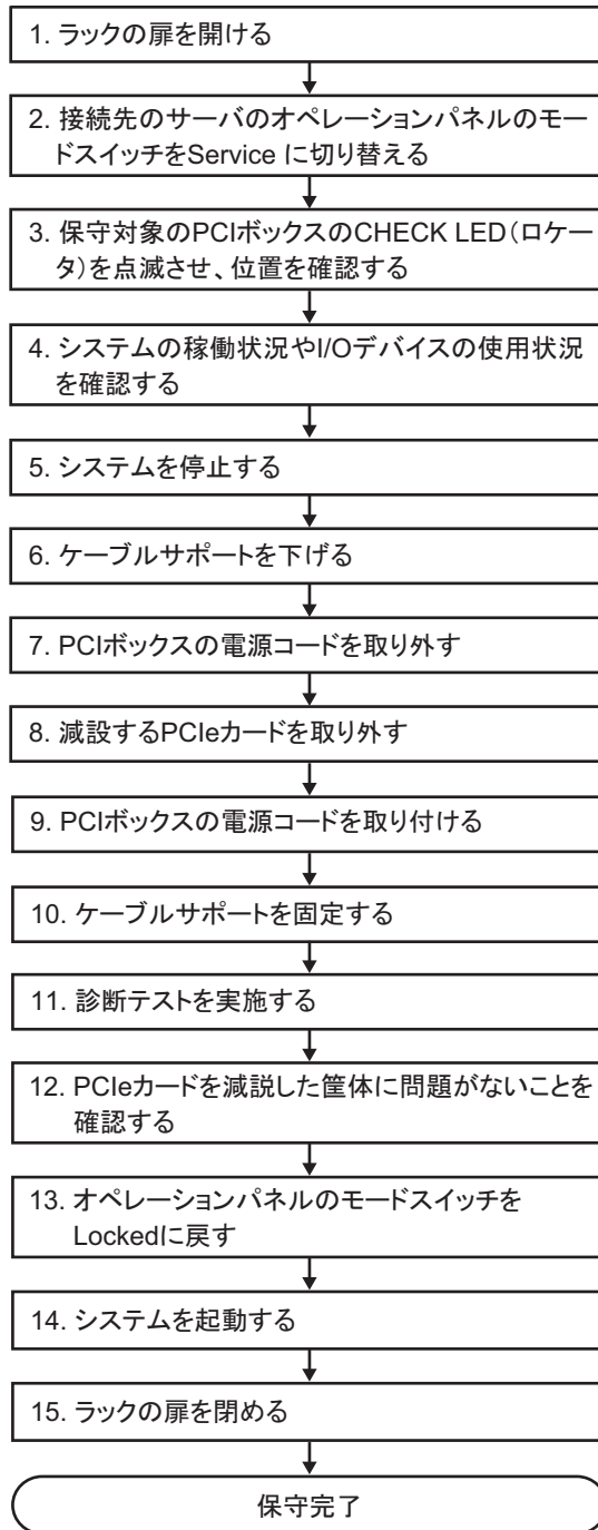
図 7-11 停電減設のながれ（システム停止によるリンクカードの切り離し）
