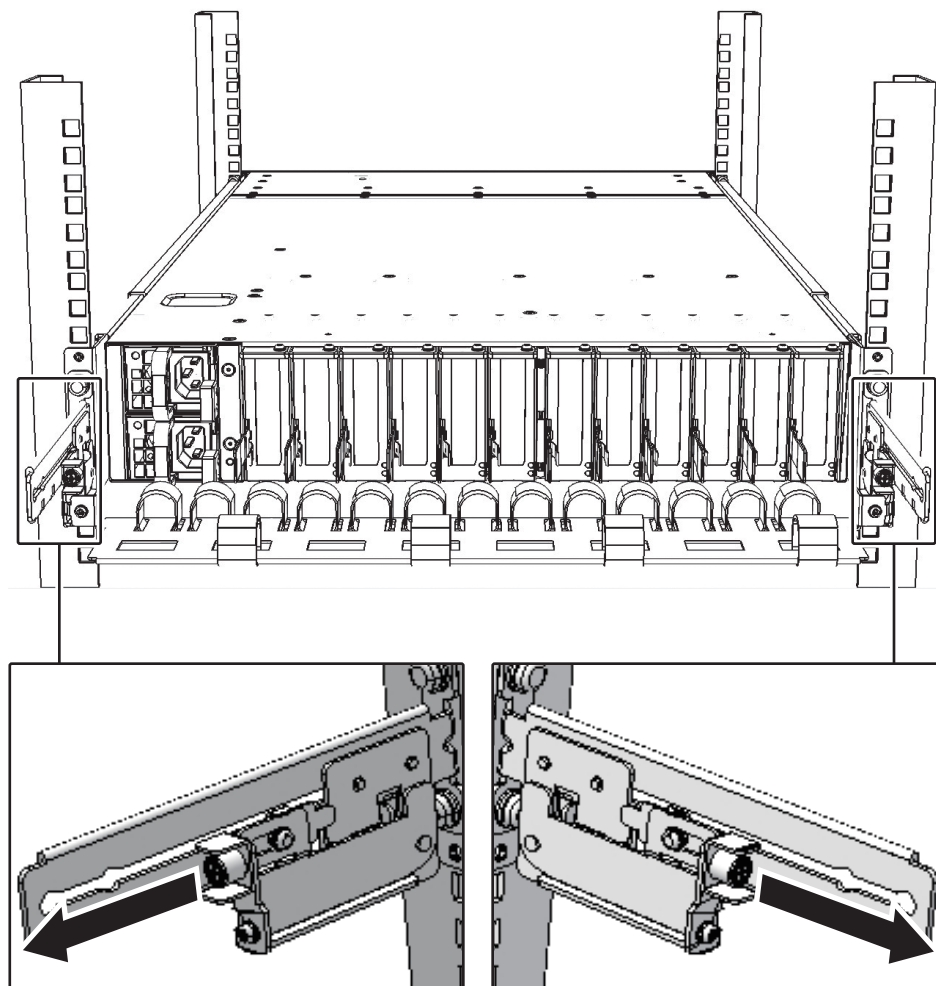
図 5-1 ケーブルサポートのねじの位置
