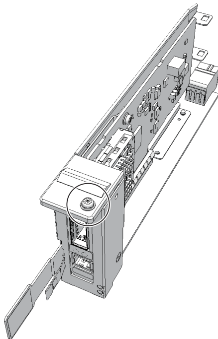
図 9-7 金具の取り付け
