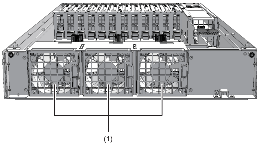
図 2-1 前面からアクセス可能なコンポーネントの位置
