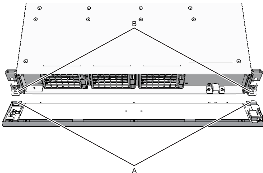
図 6-1 フロントカバーの取り付け
