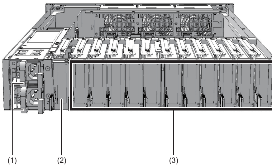
図 2-2 背面からアクセス可能なコンポーネントの位置
