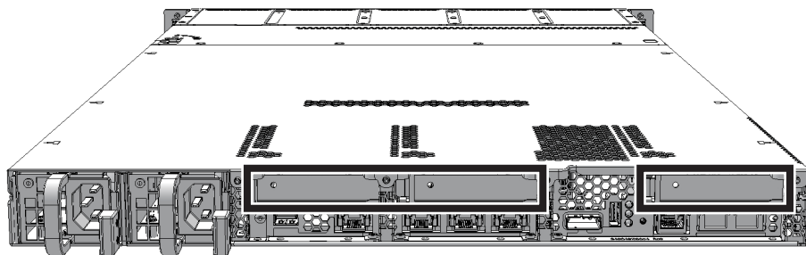
図 10-1 リンクカードの搭載位置 (SPARC M12-1)
