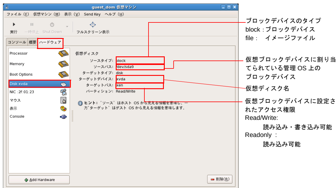
図 8.8 仮想マシンの詳細画面 (VBD 情報)
