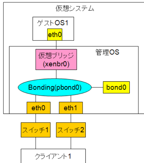
図 D.1 Bonding 使用時の仮想ブリッジ構成例 (1)
