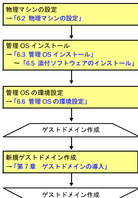
図 6.1 仮想システムの導入のながれ
