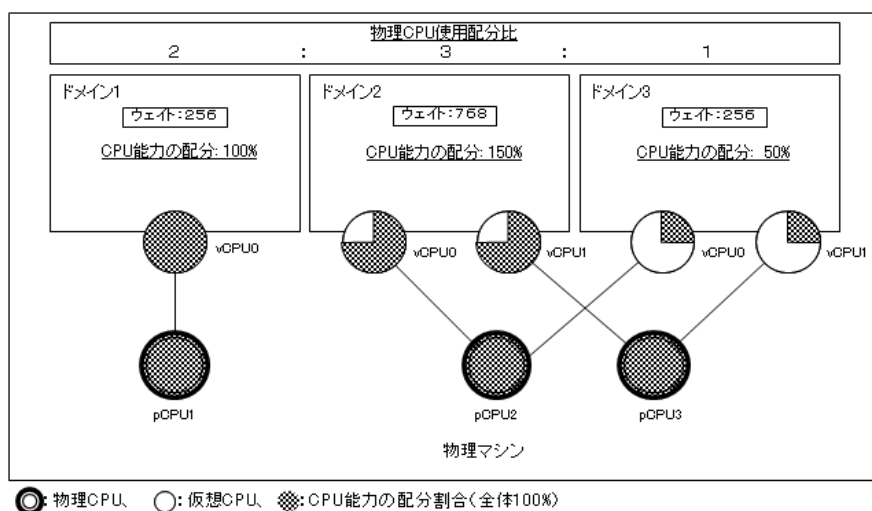
図 4.4 ドメインのウェイトの指定例
