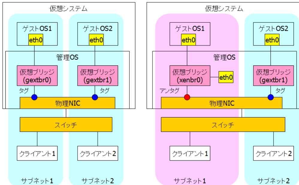
図 3.9 タグ VLAN 機能を使用した場合の仮想ネットワークの構成例
