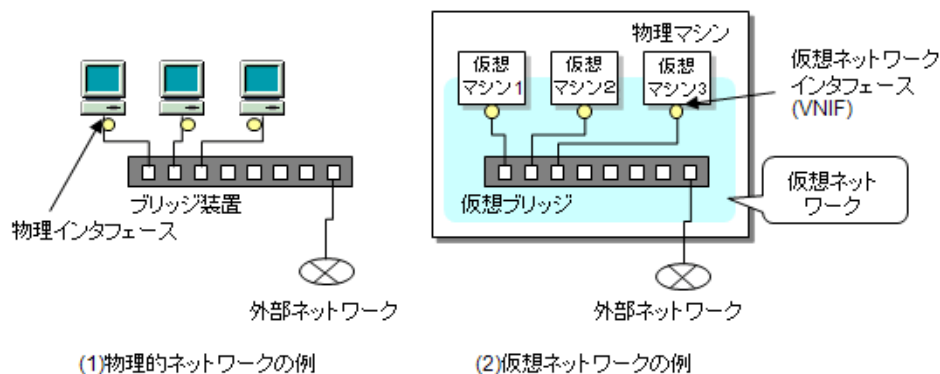
図 1.15 物理ネットワークと仮想ネットワーク
