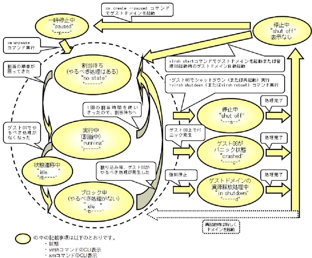
図 8.3 ドメインの状態遷移
