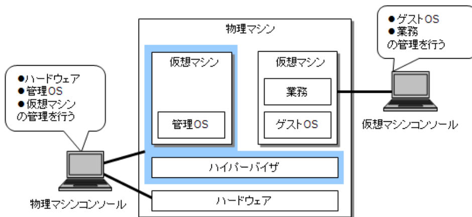
図 1.18 仮想マシン環境のコンソール
