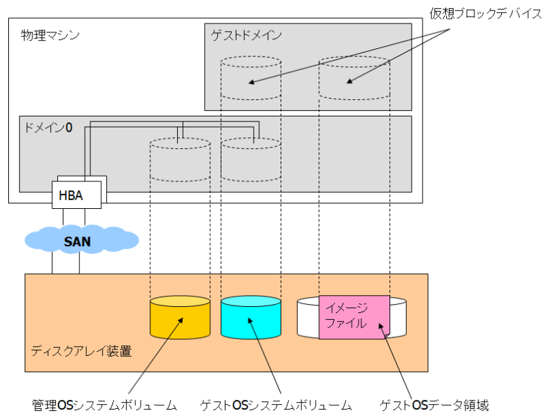
図 3.19 イメージファイルを仮想ブロックデバイスとして使用する場合のディスク構成例 (1)
