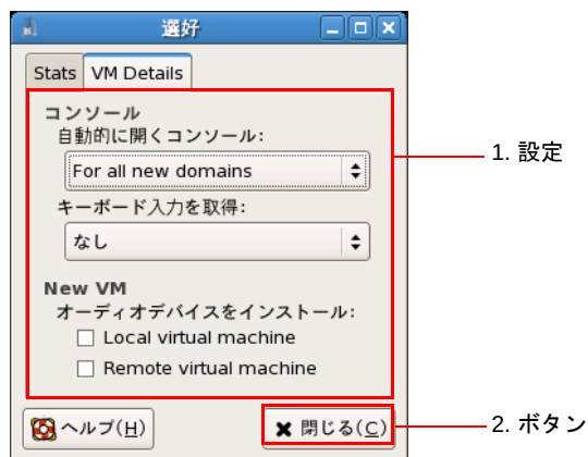
図 C.5 選好画面 -2
