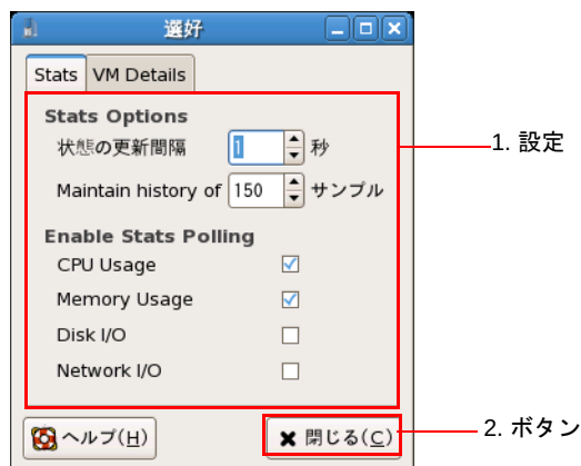
図 C.4 選好画面 -1
