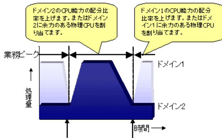
図 4.2 業務の運用時間に合わせた CPU 能力の配分比率と物理 CPU 割当の変更
