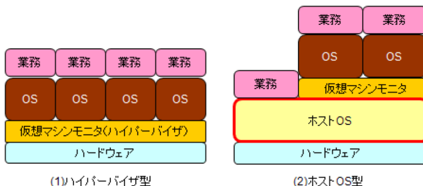
図 1.3 ソフトウェアによる仮想化方式
