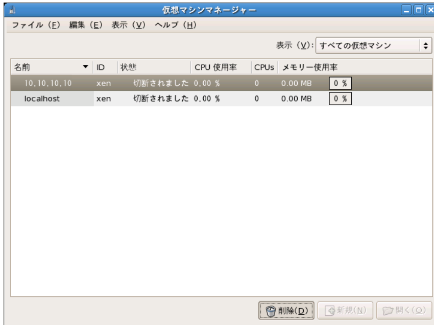
図 9.28 削除画面
