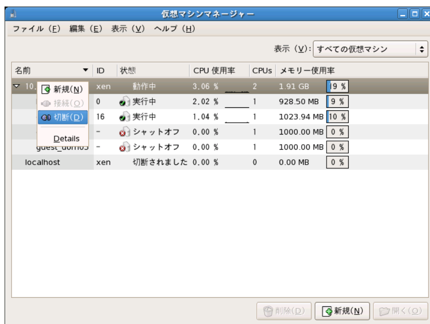
図 9.27 切断画面
