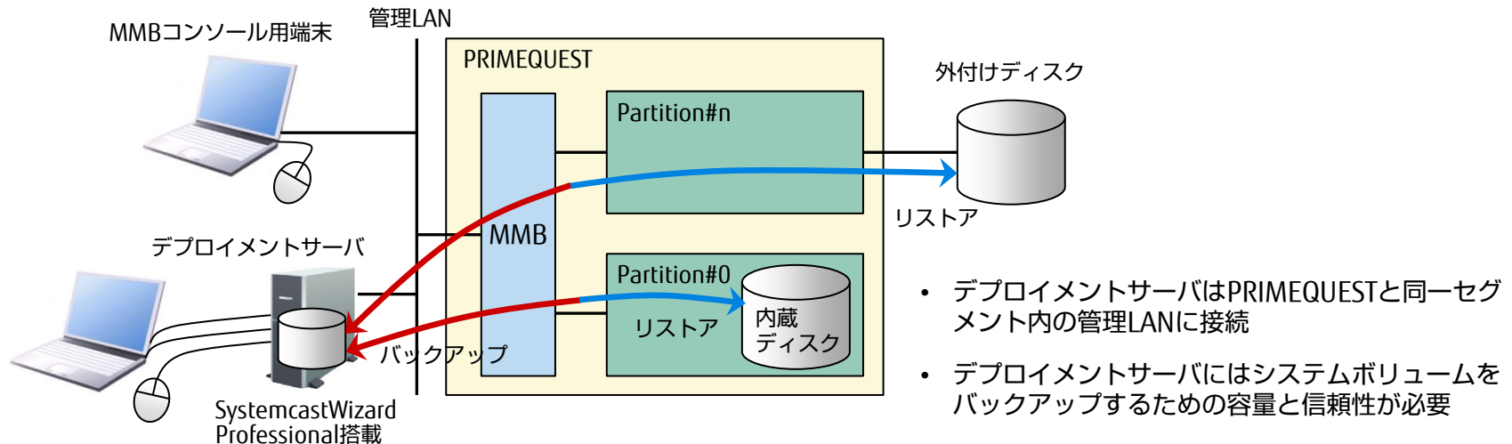
【SystemcastWizard Professionalによるバックアップの構成】
