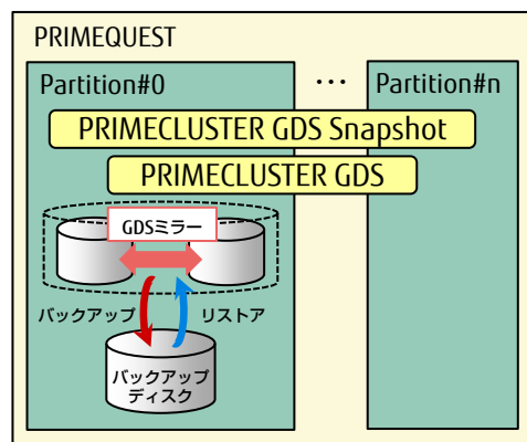
【内蔵ディスクを使用したバックアップの構成例】
