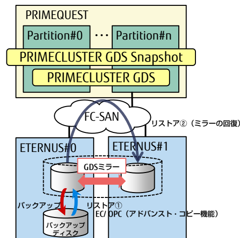
【ETERNUSを使用したバックアップの構成例】
