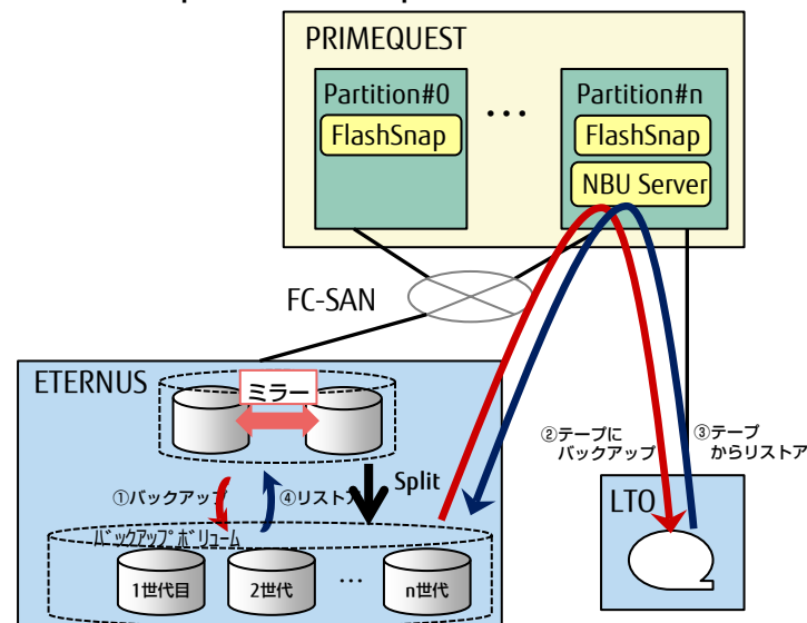
【FlashSnapとNetBackupによるオフホストバックアップ】
