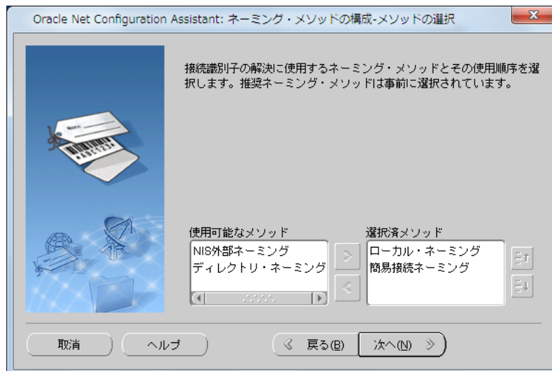
図 4-30 ネーミング・メソッドの構成-メソッドの選択
