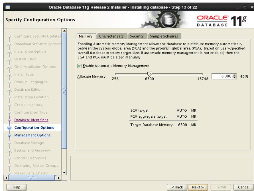
図 4-13 Specify Configuration Options
