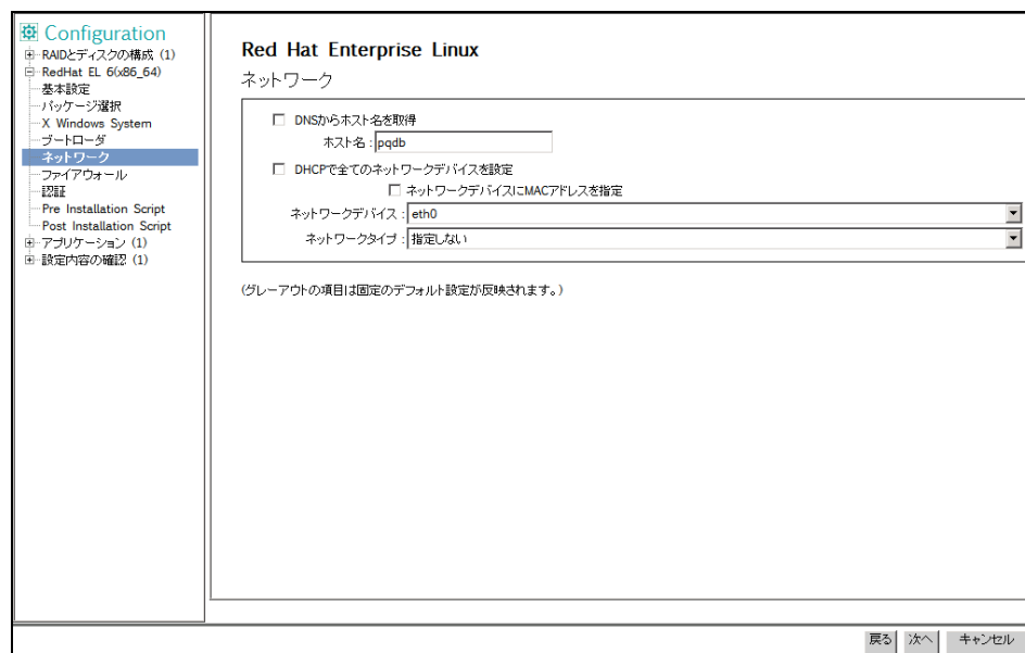
図 2-9 ネットワーク
