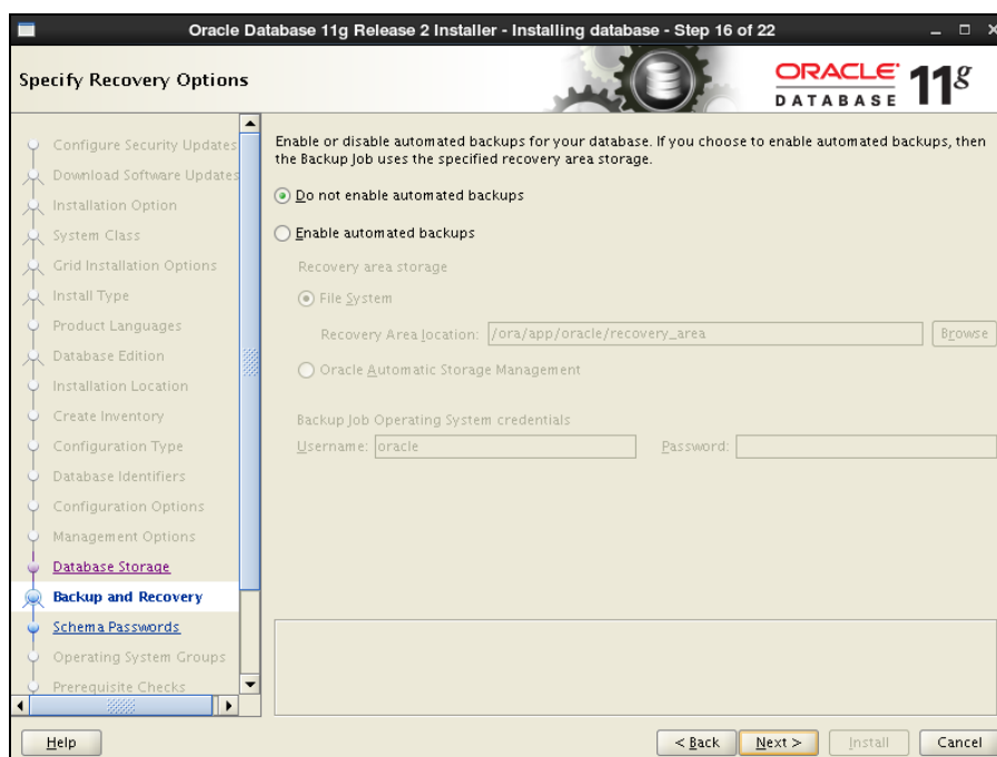
図 4-15 Specify Recovery Options
