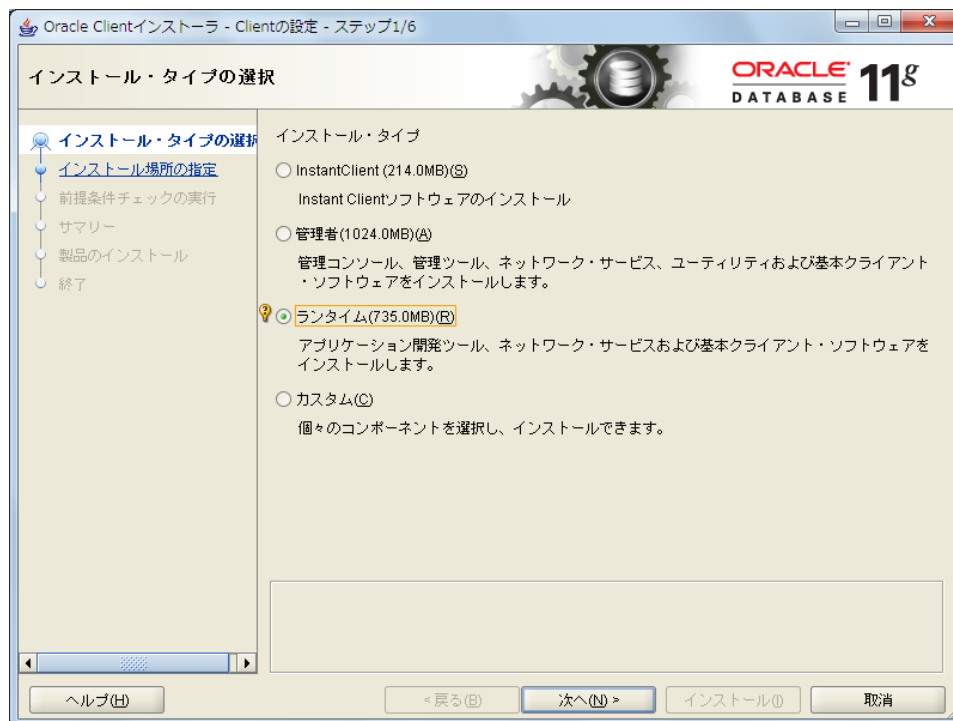
図 4-23 インストール・タイプの選択
