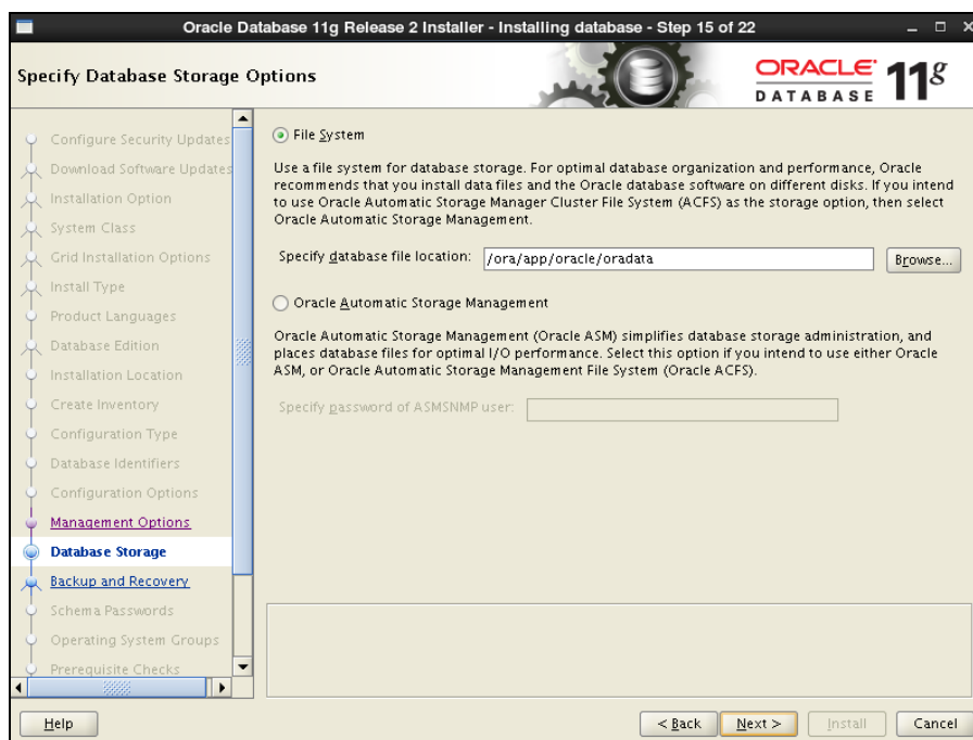
図 4-14 Specify Database Storage Options
