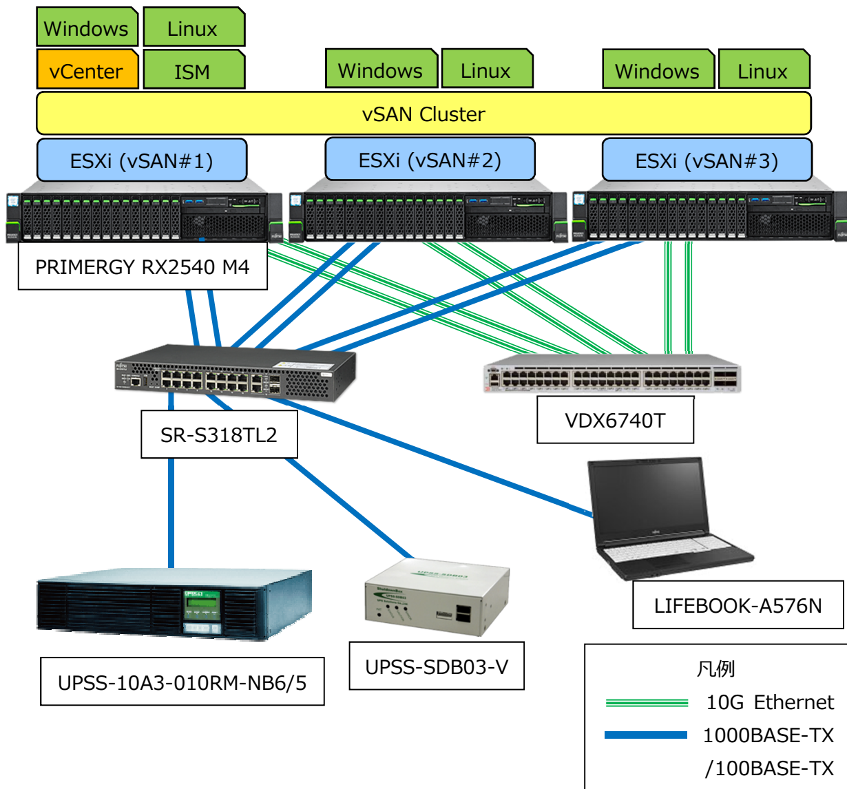
図 1 : PRIMEFLEX for VMware vSAN 検証構成
