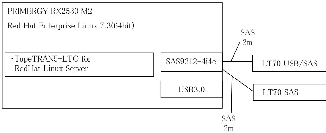
図 2 PRIMERGY RX2530 M2 SAS 接続環境
