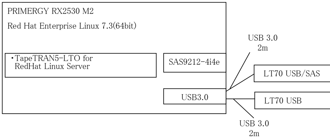
図 1 PRIMERGY RX2530 M2 USB 接続環境
