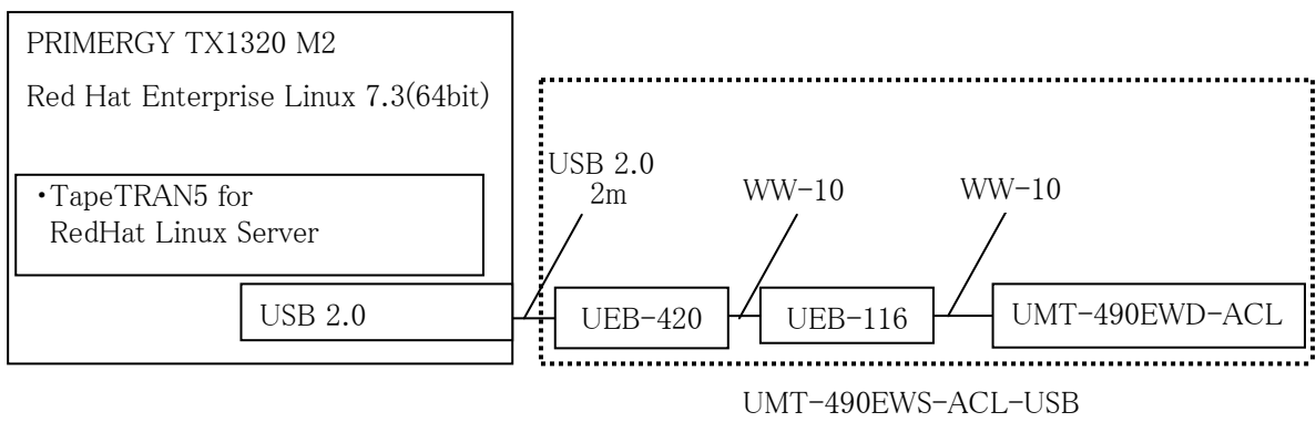
図 4 UMT-490EWS-ACL-USB 検証環境
