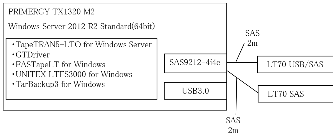
図 2 PRIMERGY TX1320 M2 SAS 接続環境
