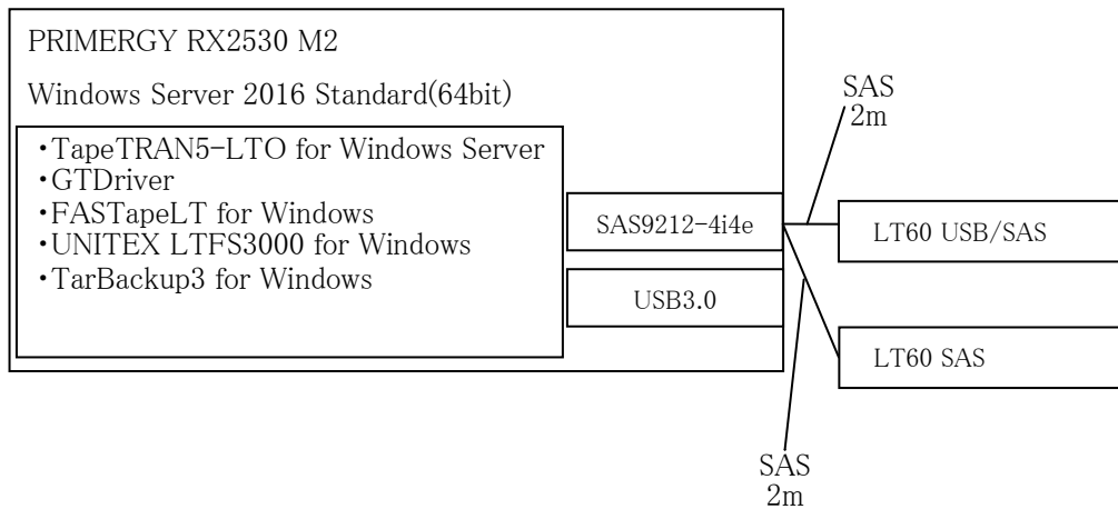
図 2 PRIMERGY RX2530 M2 SAS 接続環境
