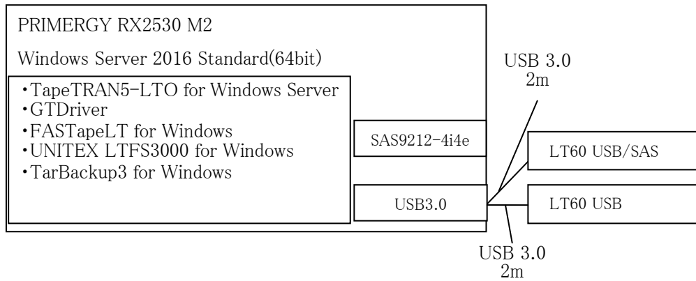
図 1 PRIMERGY RX2530 M2 USB 接続環境
