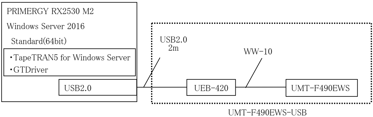
図 3 UMT-F490EWS-USB 検証環境
