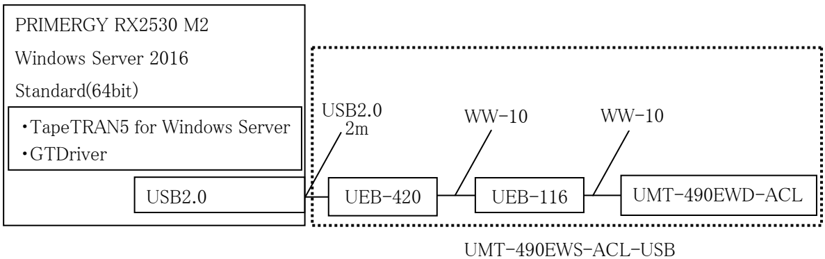
図 4 UMT-490EWS-ACL-USB 検証環境
