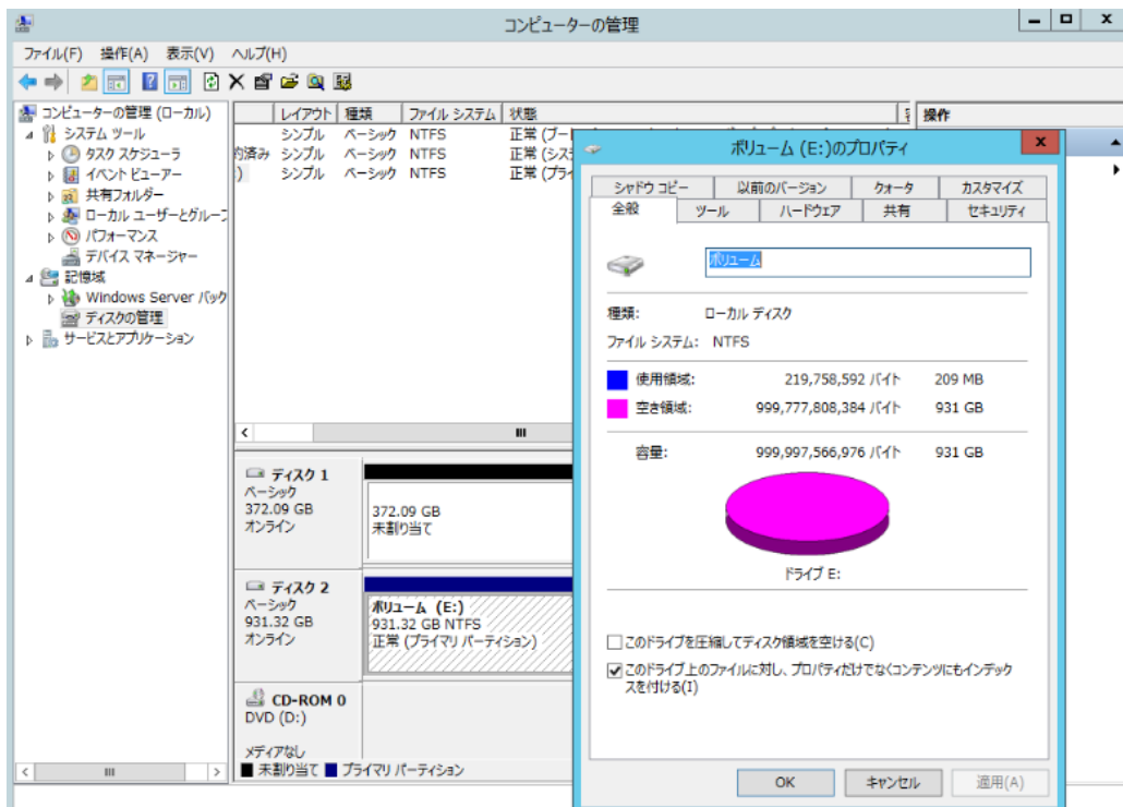
図 8：フォーマットの正常終了を確認
