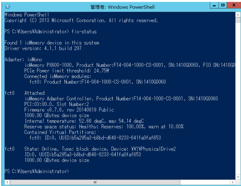
図 5 : fio-status コマンドよりデバイスのステータスが正常であることを確認
