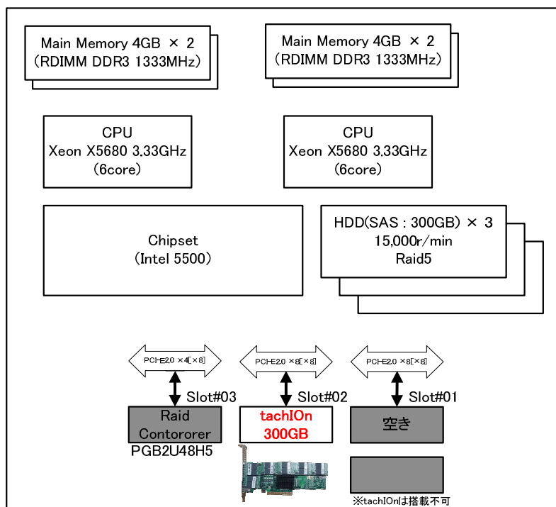
図2-1. RX200S6テスト構成
