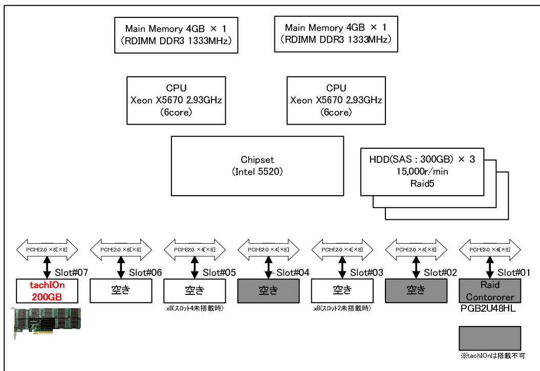
図2-1. TX300S6テスト構成
