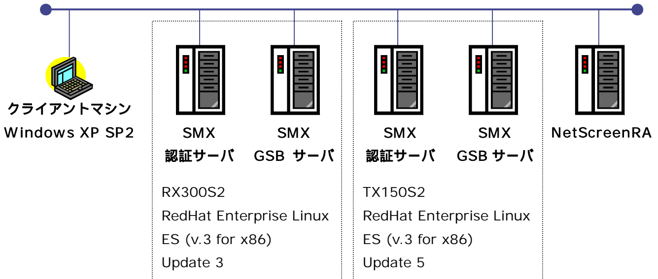
Fig. 1 検証環境構成図
