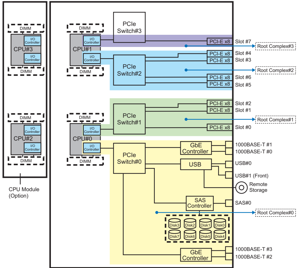
図 3-2 SPARC M10-4Sの4CPU（4ルートコンプレックス）時のハードウェアブ ロック図
