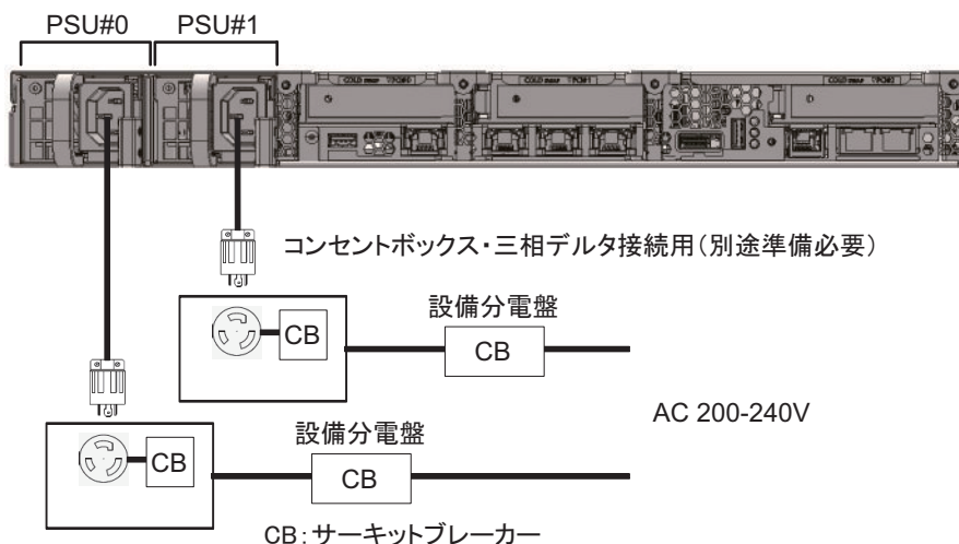
図 2-13 三相受電時の電源系統図（デルタ接続）
