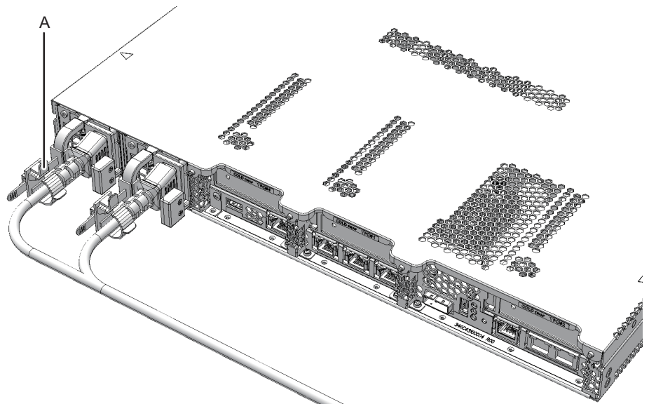
図 4-5 ケーブルクランプのロック
