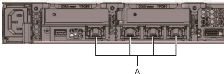
図 4-2 10 GbE LANポートの位置
