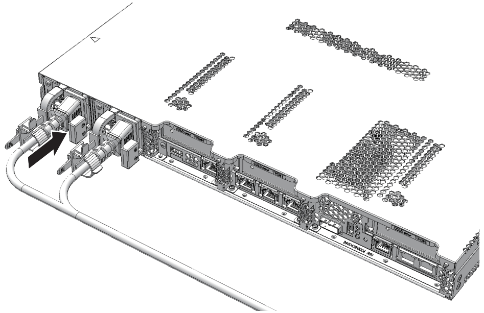
図 4-4 電源コードの取り付け
