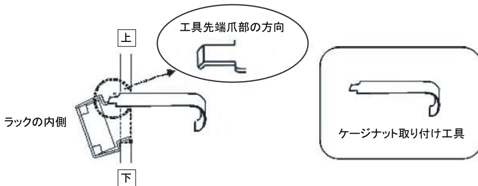
図 3-15 ケージナット取り付け工具の使用
