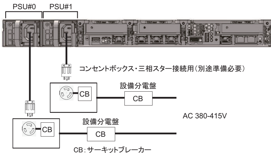
図 2-12 三相受電時の電源系統図 (スター接続)
