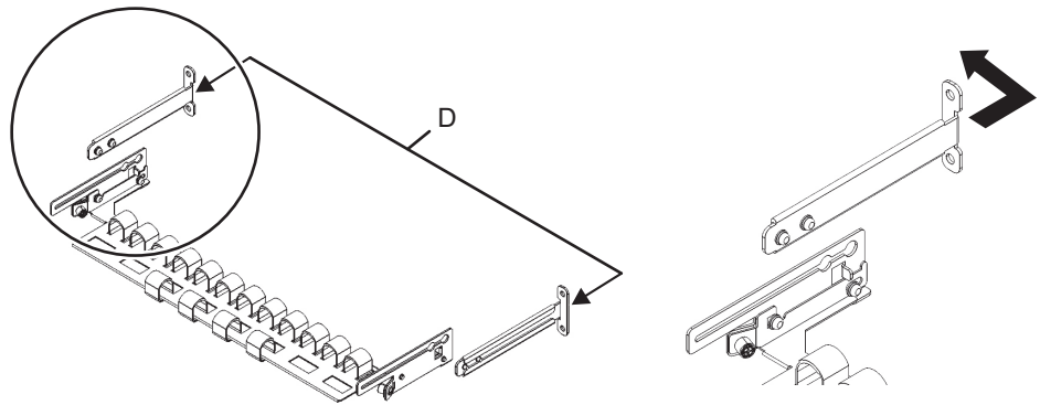
図 3-23 ケーブルサポート固定金具の取り外し（2）
