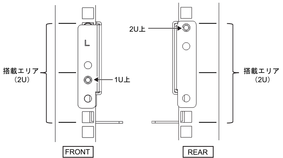
図 3-19 レールの取り付け：突起部の位置（角穴支柱の場合）
