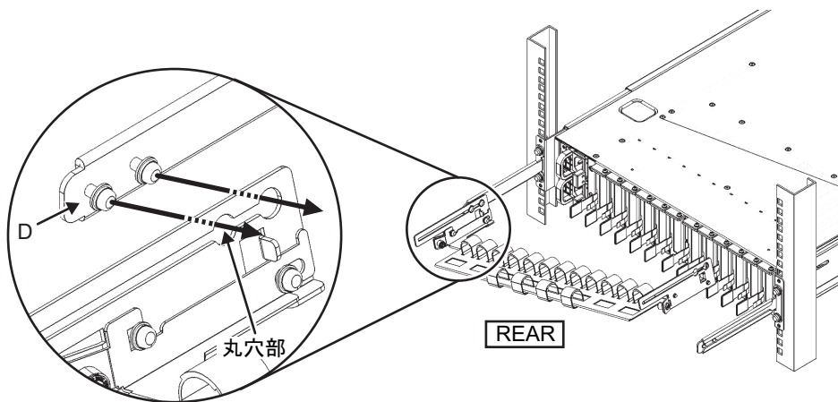
図 3-29 ケーブルサポートの取り付け (1)
