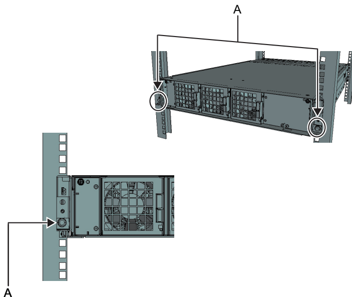
図 3-28 PCIボックスの固定
