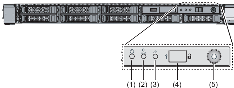
図 2-19 SPARC M12-1のオペレーションパネル
