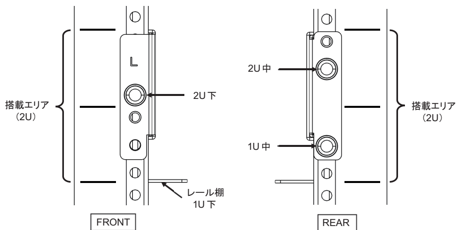
図 3-21 レールの取り付け：M6ねじ穴支柱の場合
