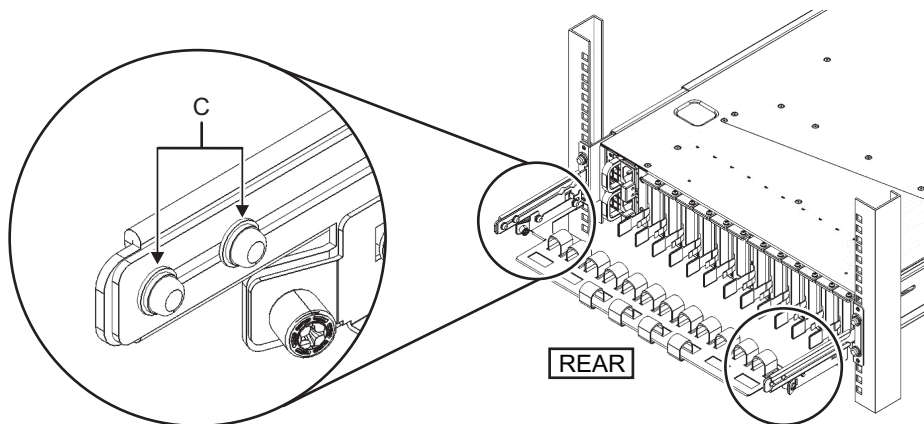
図 3-30 ケーブルサポートの取り付け (2)
