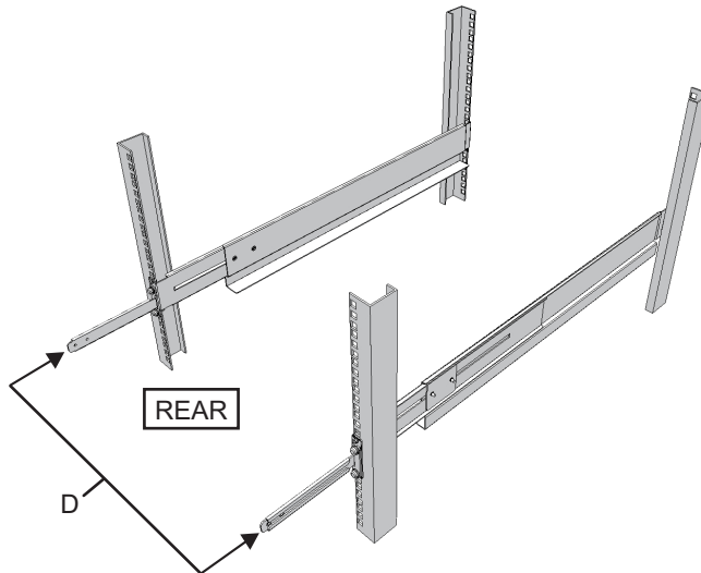
図 3-24 ケーブルサポート金具の取り付け
