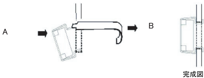
図 3-16 ケージナットの取り付け
