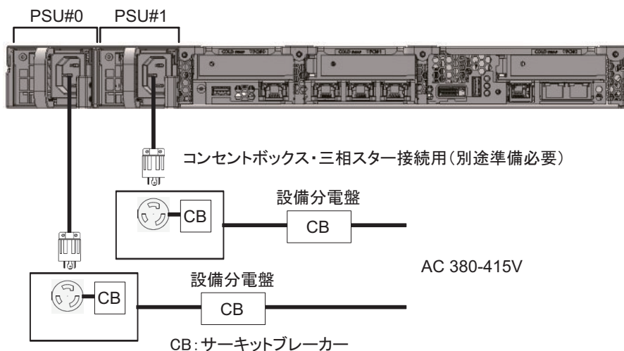
図 2-8 三相受電時の電源系統図（スター接続）
