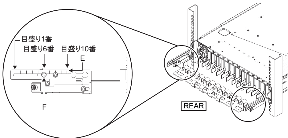
図 3-31 ケーブルサポートの取り付け (3)
