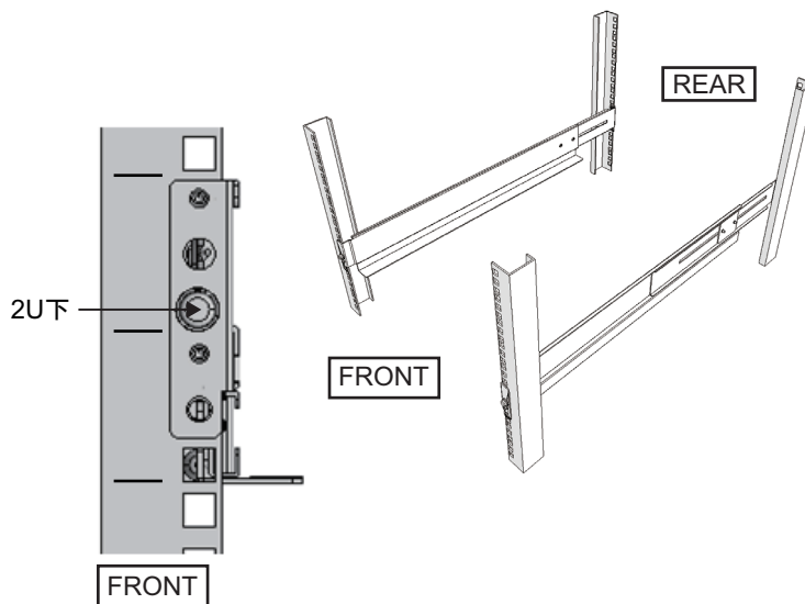
図 3-20 レールの取り付け：ねじの固定位置（角穴支柱の場合）
