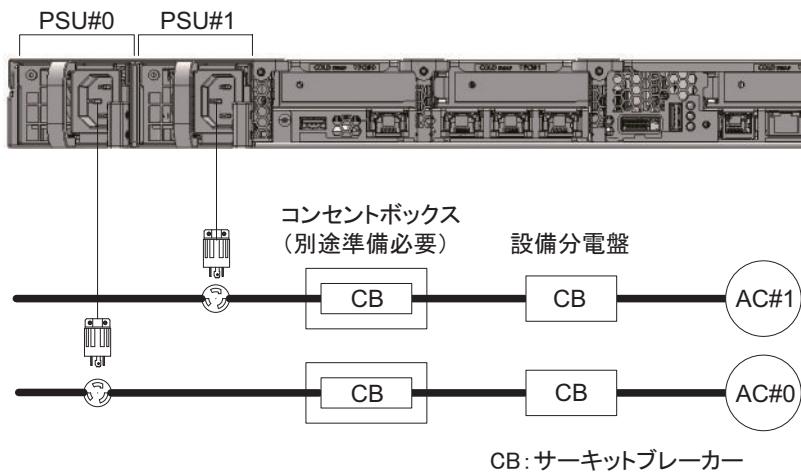
図 2-11 単相受電時の電源系統図
