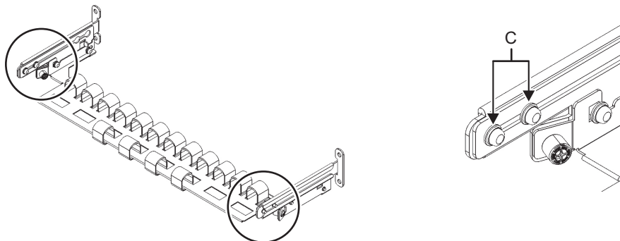
図 3-22 ケーブルサポート固定金具の取り外し (1)
