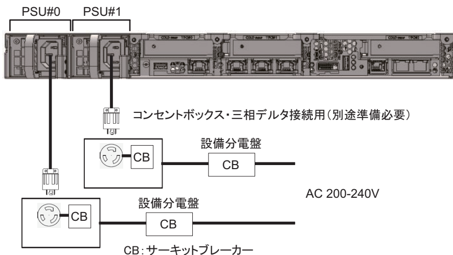
図 2-9 三相受電時の電源系統図（デルタ接続）
