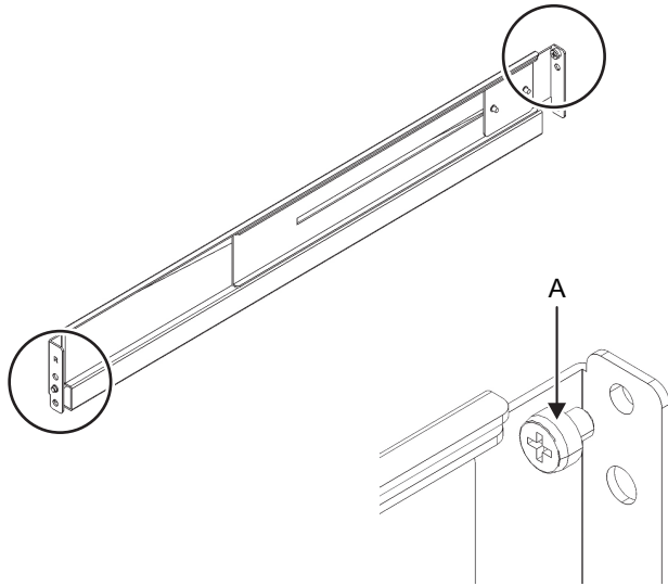
図 3-17 レールのピンの取り外し
