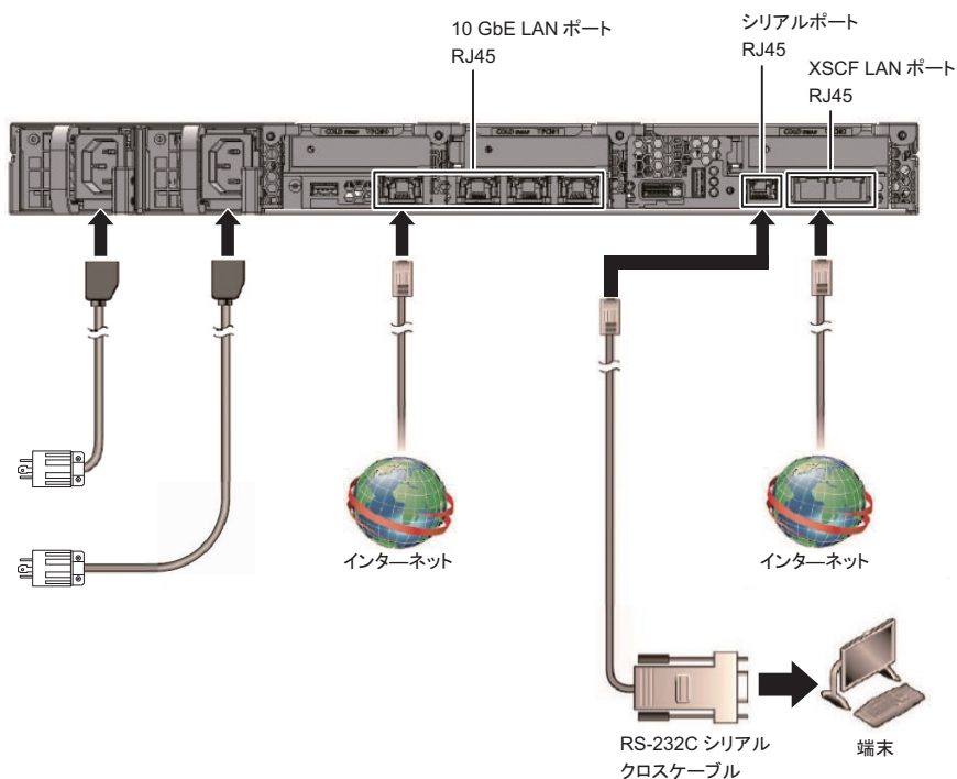
図 2-18 ネットワーク構成例
