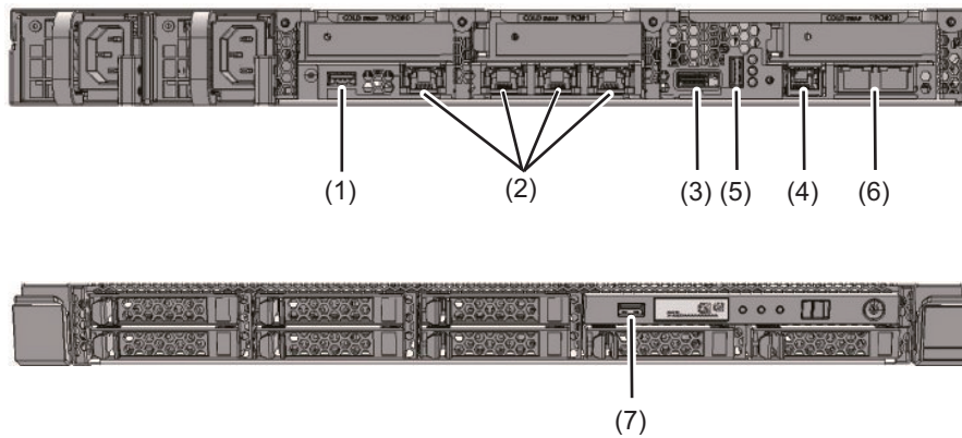
図 2-15 ネットワーク接続用ポートの位置
