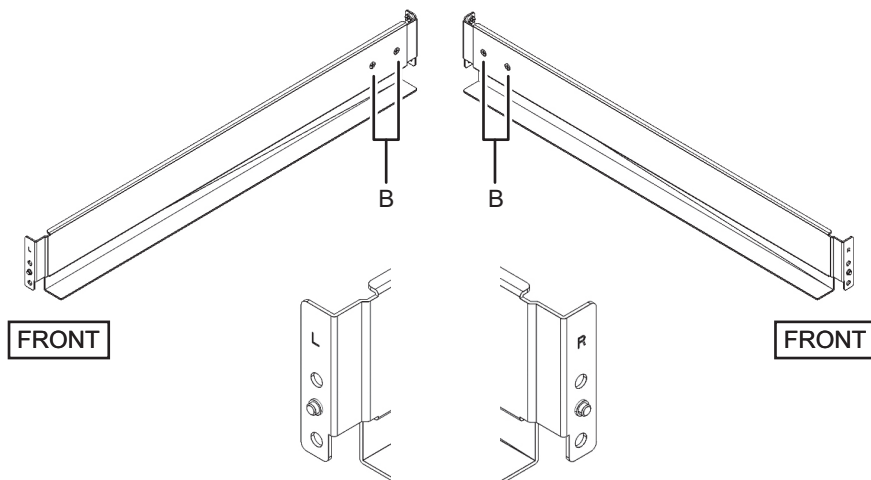
図 3-18 レールの側面のねじ
