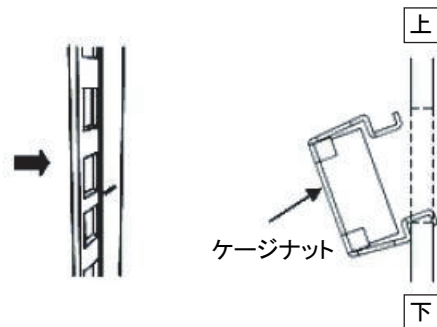
図 3-14 ケージナットのつめの向き
