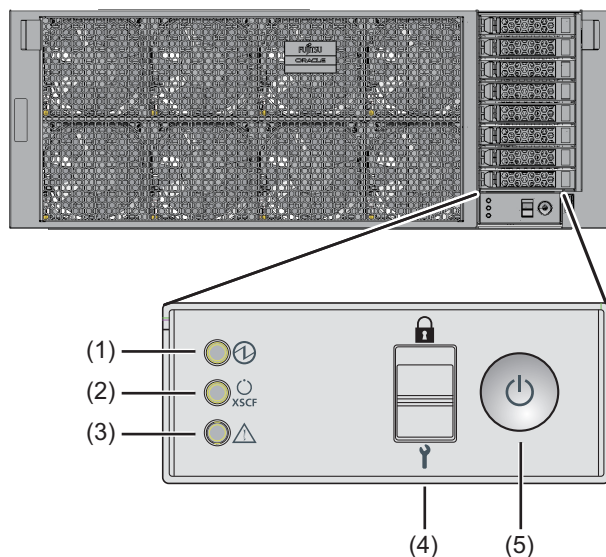
図 2-17 SPARC M12-2のオペレーションパネル
