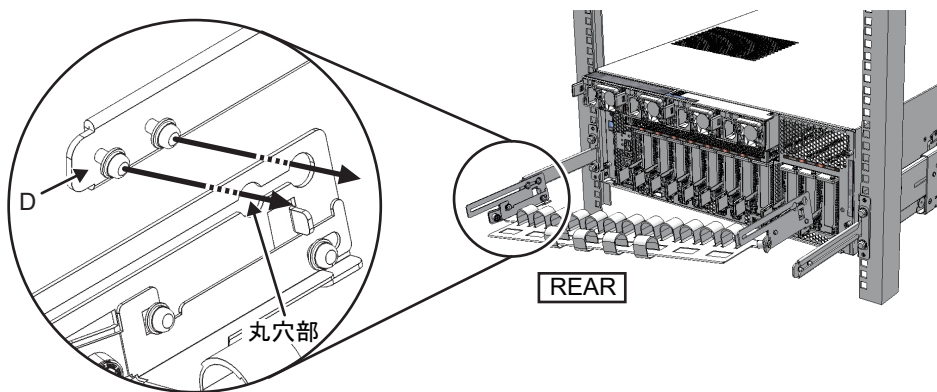
図 3-17 ケーブルサポートの取り付け (1)
