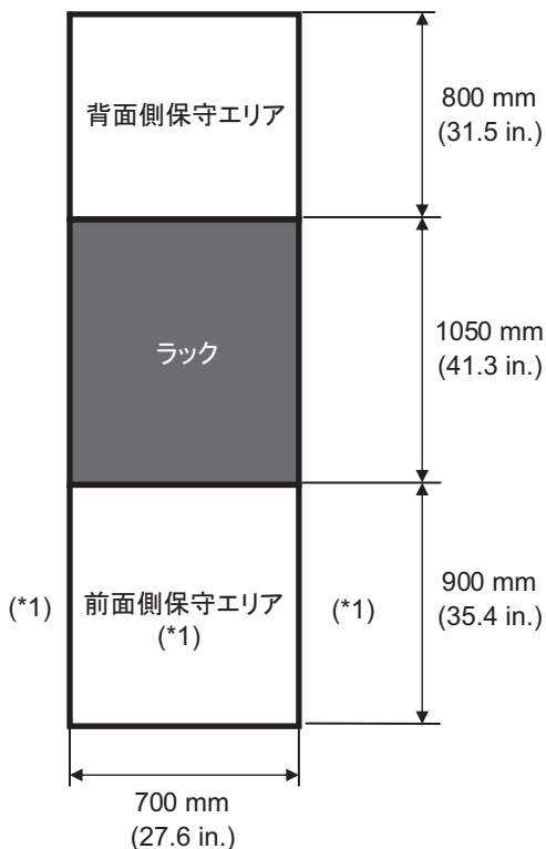
図 2-3 PCIボックスの保守エリアの例（上面図）
