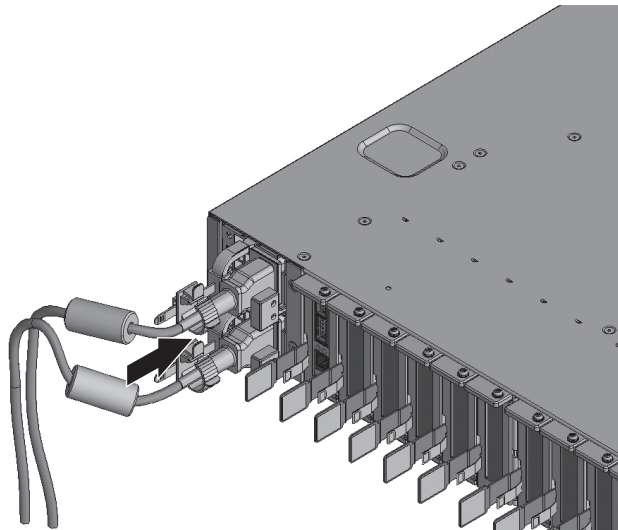
図 4-14 電源コードの取り付け
