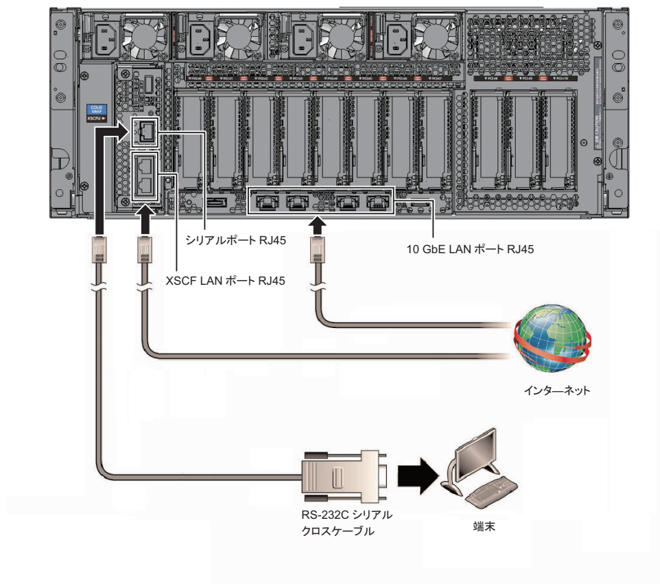
図 2-16 ネットワーク構成例
