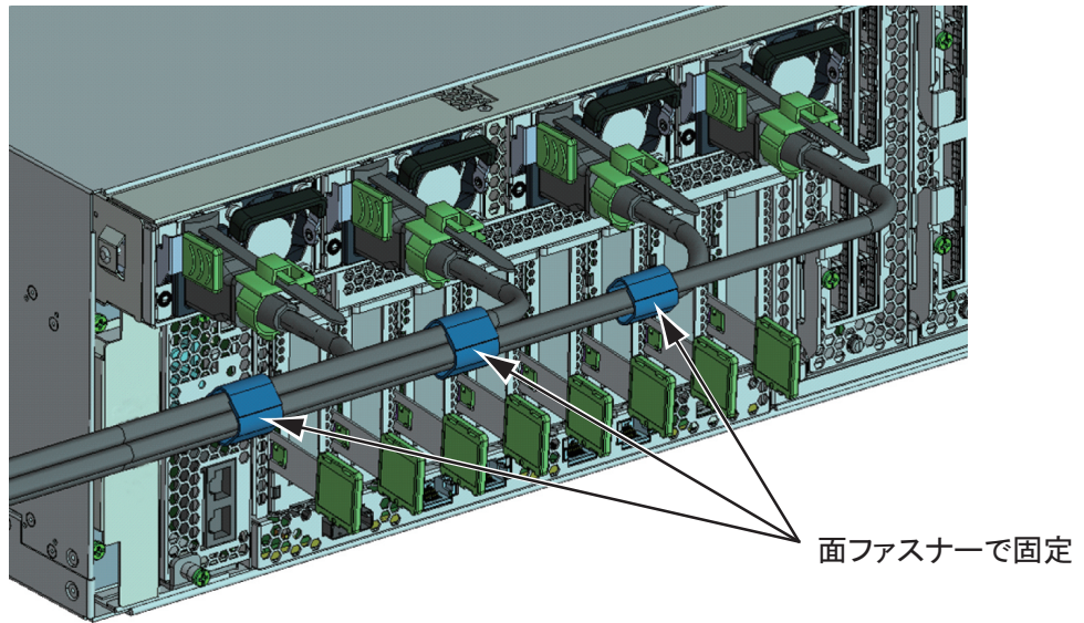
図 4-6 電源コードの結束
