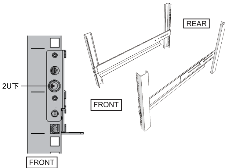
図 3-30 レールの取り付け：ねじの固定位置（角穴支柱の場合）
