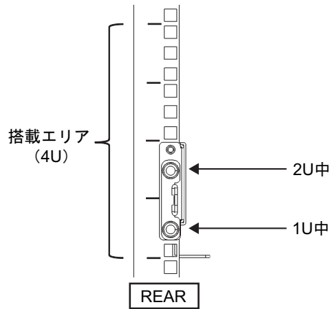
図 3-13 ケーブルサポート固定金具とレールの固定
