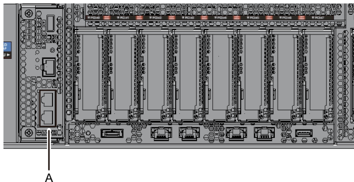
図 6-2 XSCF-LANポートの位置
