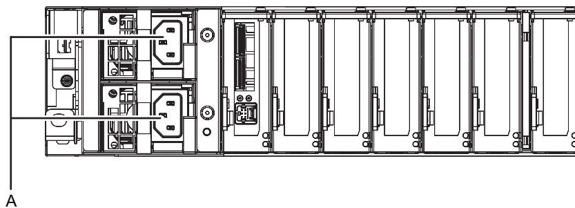
図 4-13 PCIボックスの電源ユニットの位置
