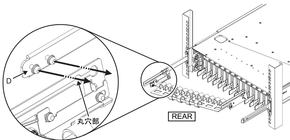
図 3-39 ケーブルサポートの取り付け (1)
