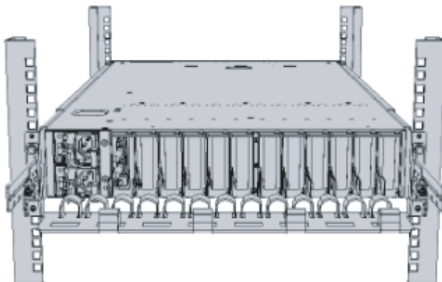
図 3-42 ケーブルサポートの取り付け完成図
