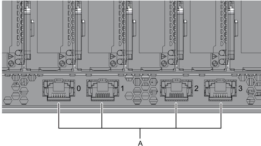
図 4-2 10 GbE LANポートの位置
