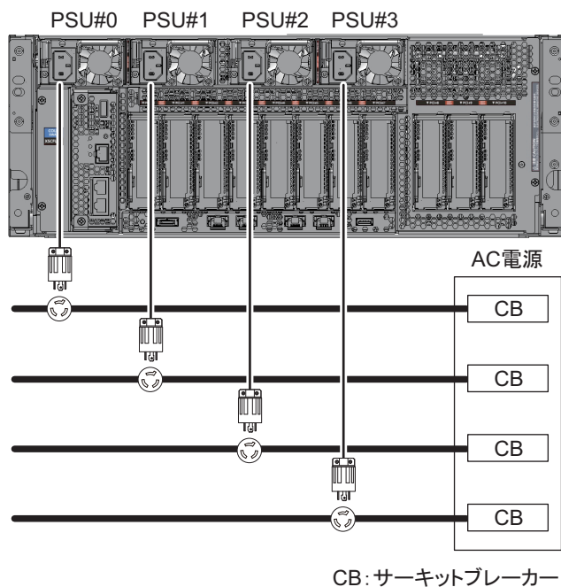
図 2-4 電源冗長接続時の電源系統図
