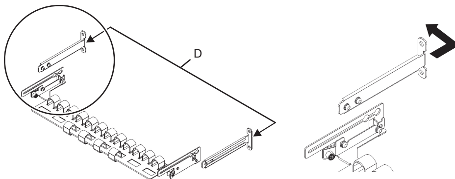
図 3-33 ケーブルサポート固定金具の取り外し (2)
