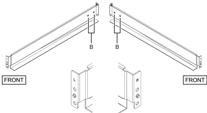
図 3-28 レールの側面のねじ
