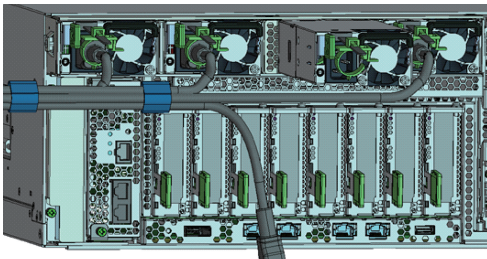
図 4-8 参考：電源ユニットの活性保守時の例
