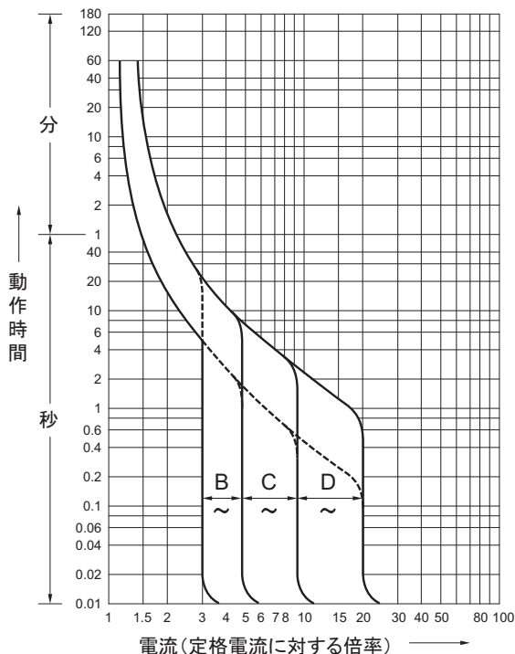
図 2-12 設備側分電盤のブレーカー特性
