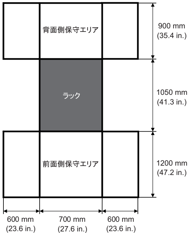
図 2-2 SPARC M12-2の保守エリアの例（上面図）
