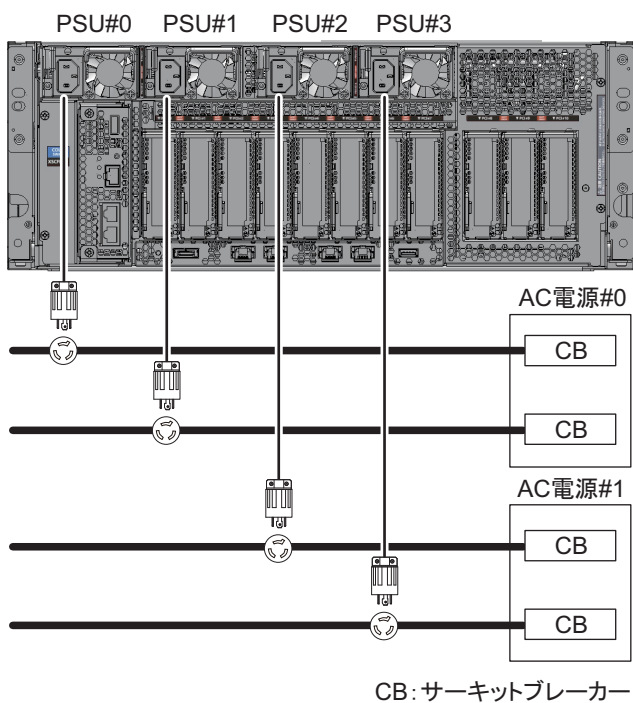
図 2-5 二系統受電時の電源系統図
