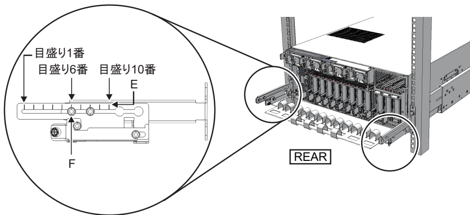
図 3-19 ケーブルサポートの取り付け (3)
