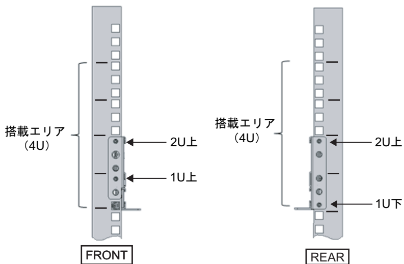
図 3-8 レールの取り付け：突起部の位置
