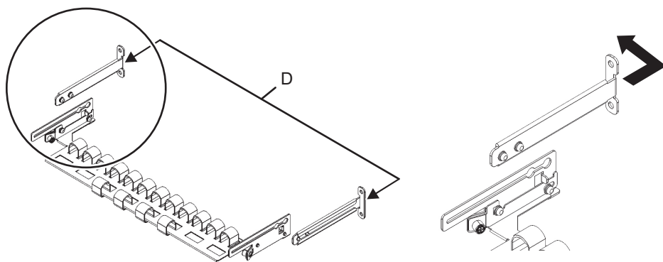
図 3-11 ケーブルサポート固定金具の取り外し (2)
