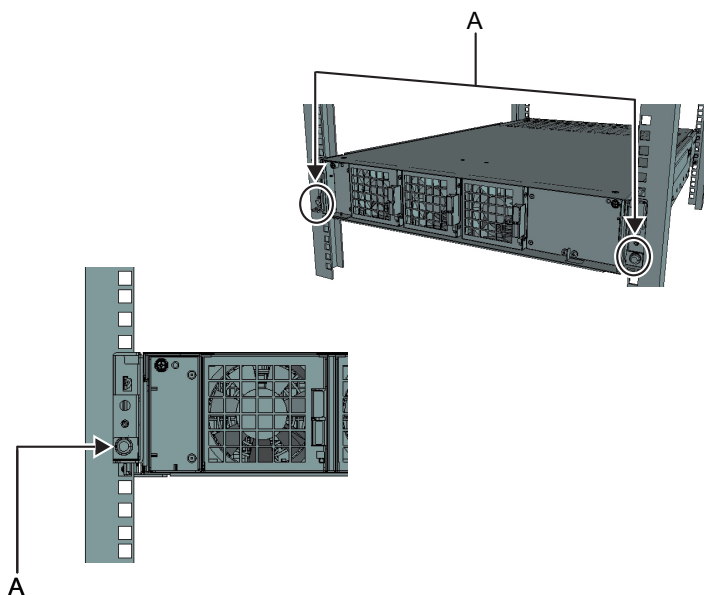
図 3-38 PCIボックスの固定
