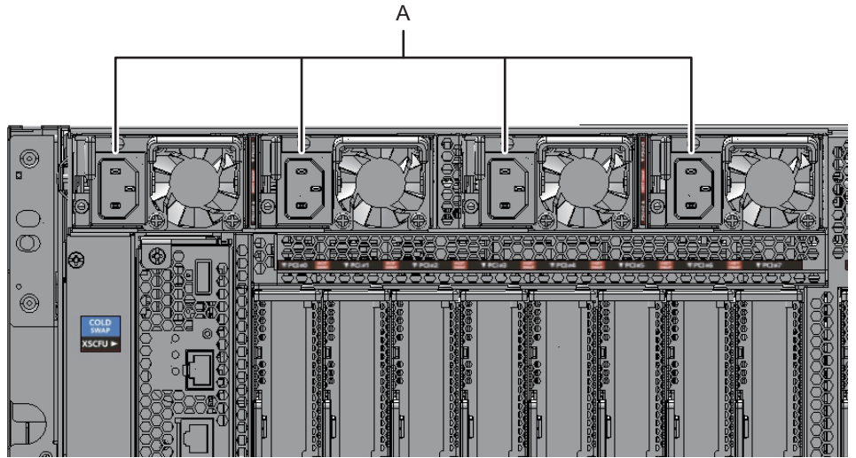
図 4-4 電源ユニットの位置
