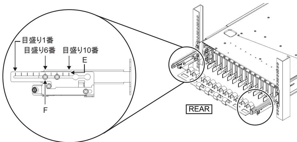
図 3-41 ケーブルサポートの取り付け (3)
