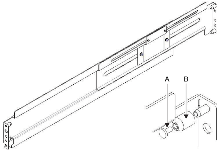
図 3-6 レールピンの取り外し
