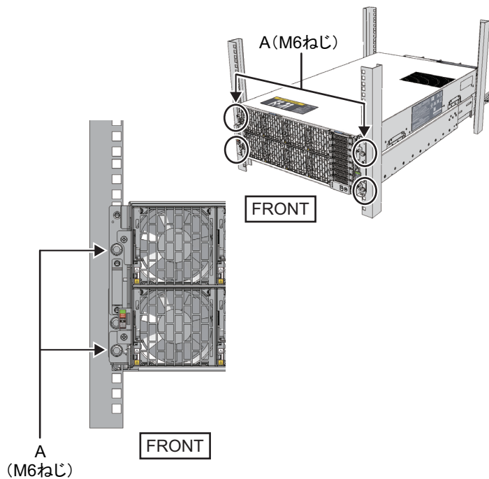
図 3-16 SPARC M12-2の固定
