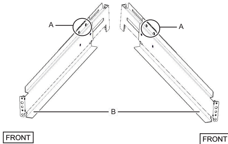
図 3-7 レールの取り付け向き
