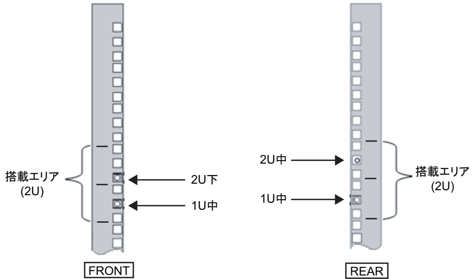
図 3-23 ラック支柱のケージナット取り付け位置
