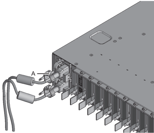
図 4-15 ケーブルクランプのロック
