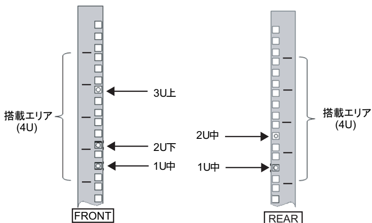
図 3-2 ラック支柱のケージナット取り付け位置
