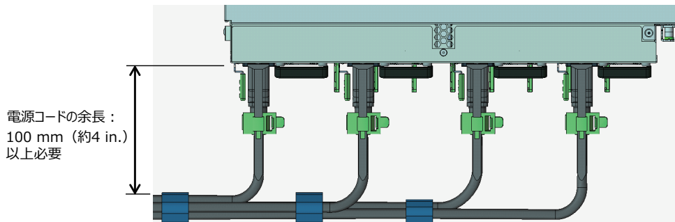
図 4-7 電源コードの余長の確保
