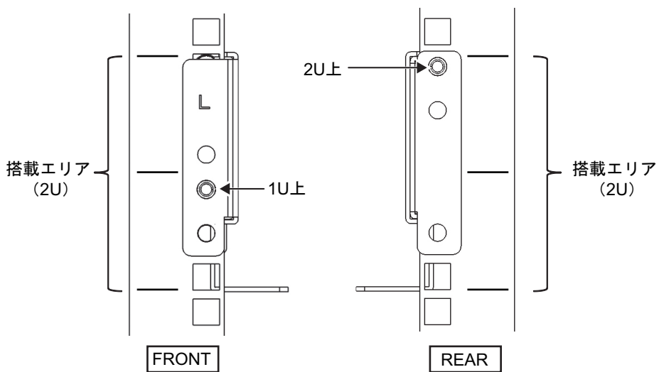
図 3-29 レールの取り付け：突起部の位置（角穴支柱の場合）
