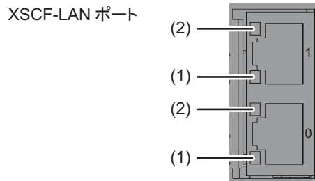
図 2-14 XSCF-LANポートのLED
