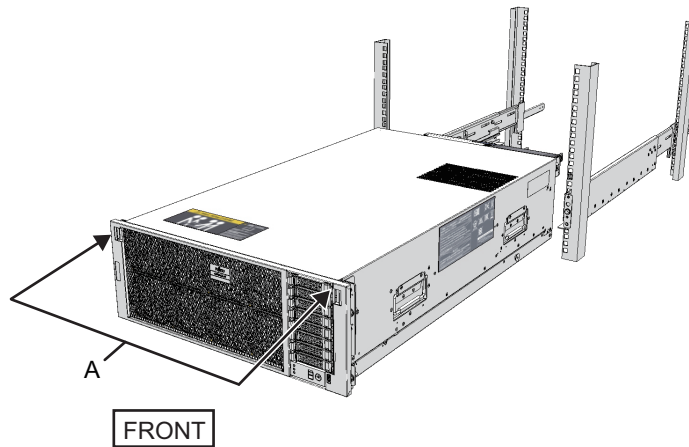
図 3-15 ラックへの搭載
