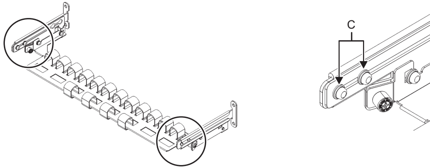
図 3-10 ケーブルサポート固定金具の取り外し（1）
