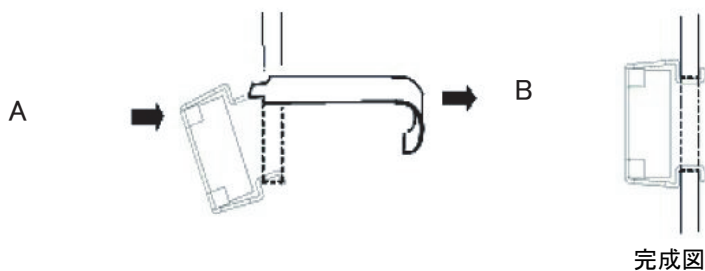
図 3-5 ケージナットの取り付け
