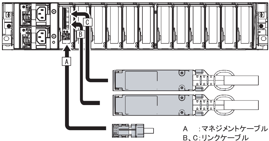
図 4-10 リンクケーブルとマネジメントケーブルの接続（PCIボックス側）
