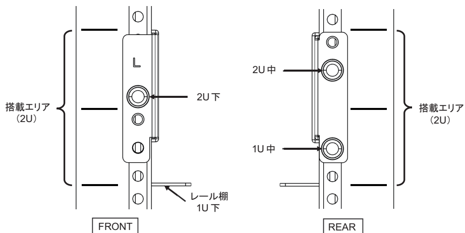
図 3-31 レールの取り付け：ねじの固定位置（M6ねじ穴支柱の場合）
