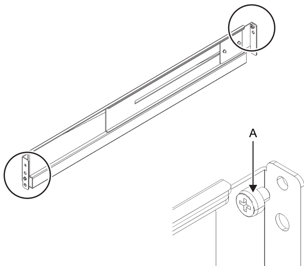
図 3-27 レールのピンの取り外し
