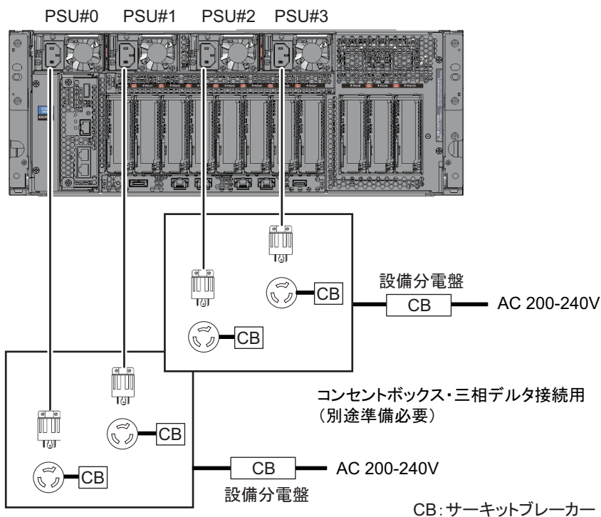
図 2-11 三相受電時の電源系統図 (デルタ接続)
