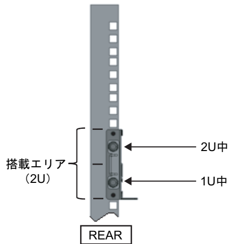
図 3-35 ケーブルサポート固定金具とレールの固定
