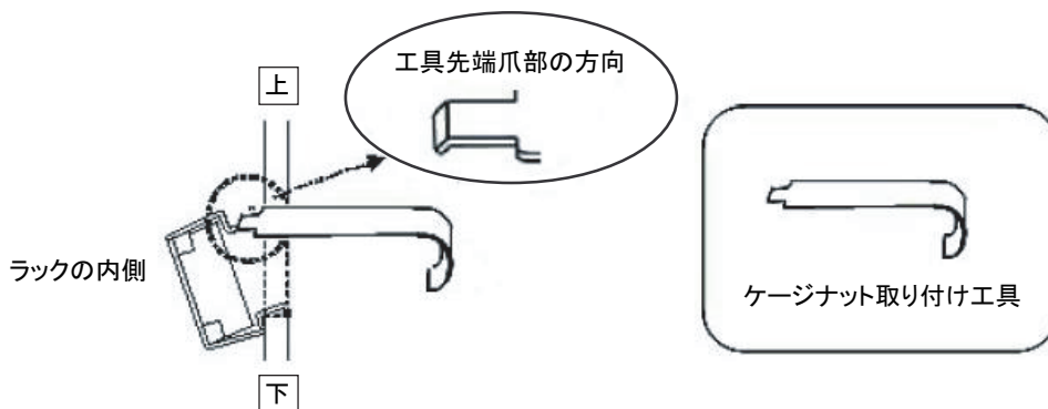
図 3-4 ケージナット取り付け工具の使用
