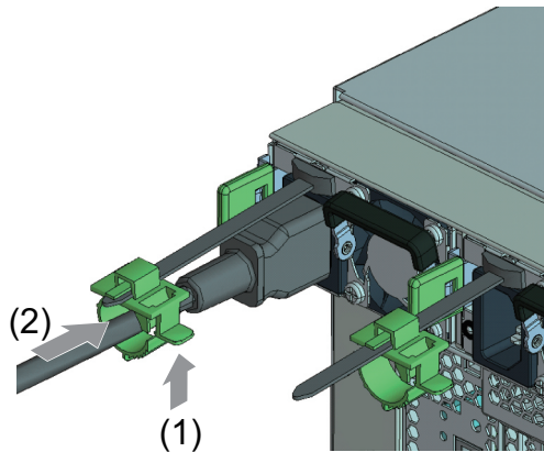
図 4-5 電源コードの固定
