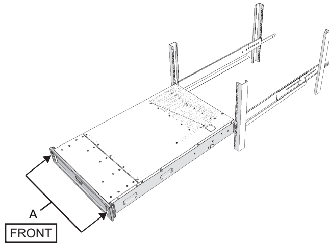
図 3-37 ラックへの搭載
