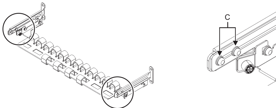
図 3-32 ケーブルサポート固定金具の取り外し (1)
