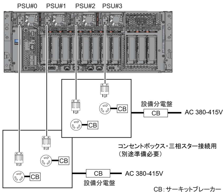
図 2-6 三相受電時の電源系統図（スター接続）
