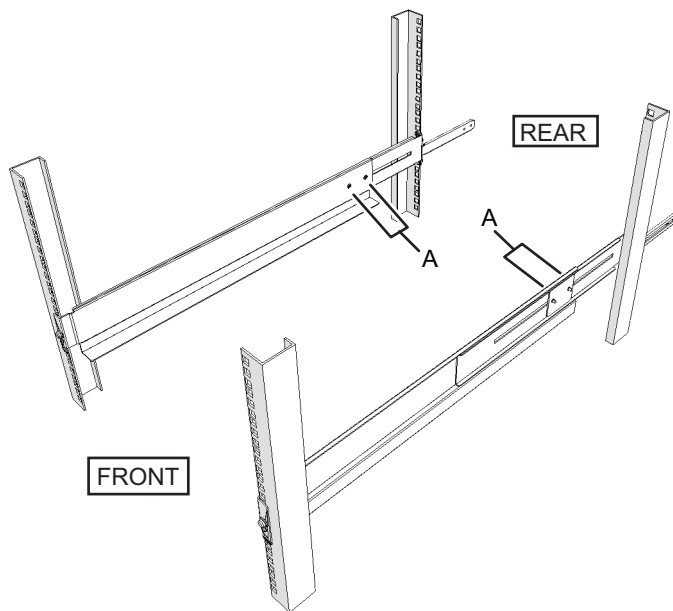
図 3-36 レール側面のねじ固定
