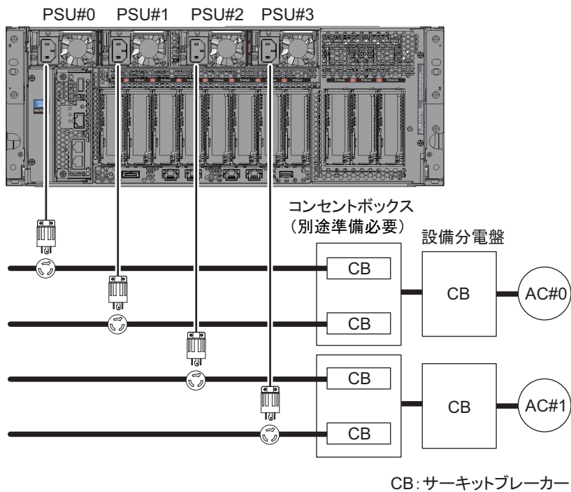
図 2-9 単相受電時の電源系統図
