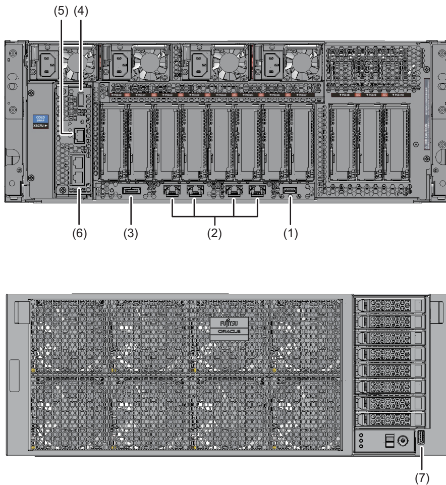
図 2-13 ネットワーク接続用ポートの位置
