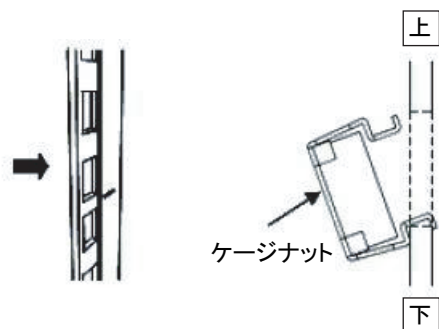
図 3-3 ケージナットのつめの向き
