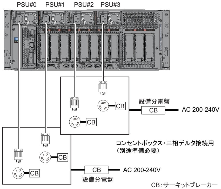
図 2-7 三相受電時の電源系統図（デルタ接続）
