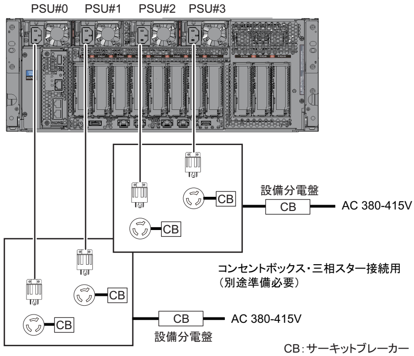
図 2-10 三相受電時の電源系統図（スター接続）
