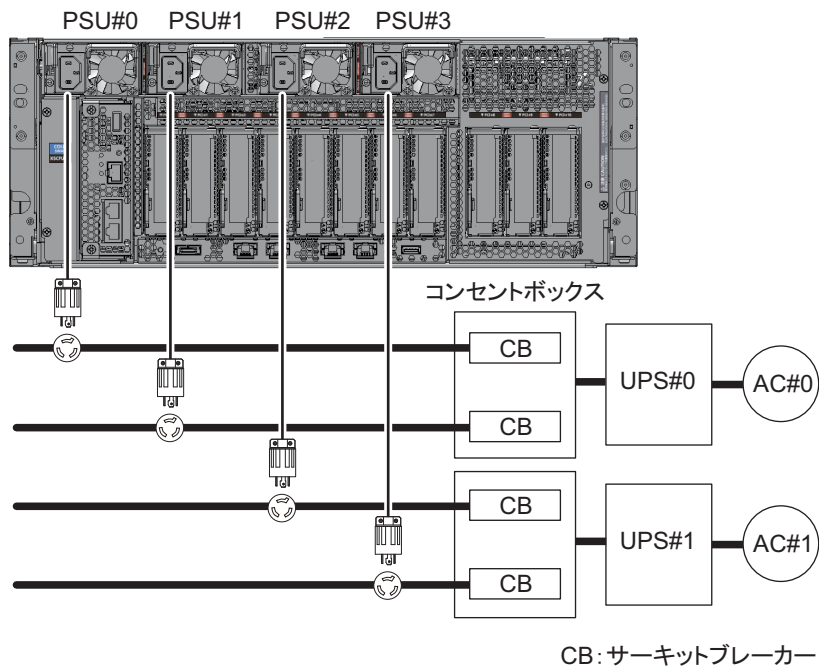
図 2-8 UPS接続時の電源系統図
