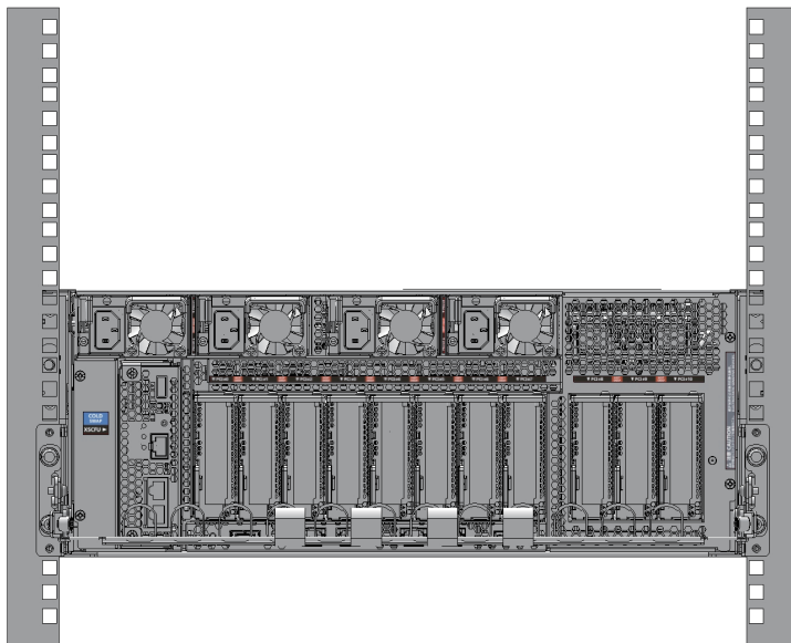
図 3-21 SPARC M12-2搭載完成図（背面）
