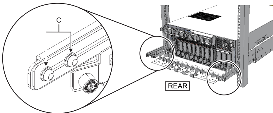
図 3-18 ケーブルサポートの取り付け (2)
