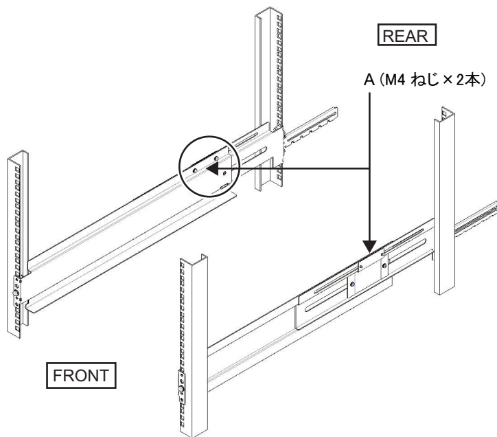
図 3-14 レール側面のねじ固定
