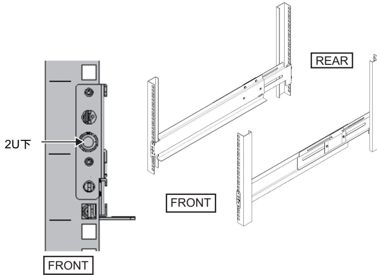
図 3-9 レールの取り付け：ねじの固定位置
