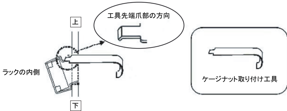
図 3-25 ケージナット取り付け工具の使用
