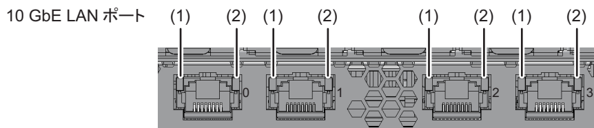
図 2-15 10 GbE LANポートのLED
