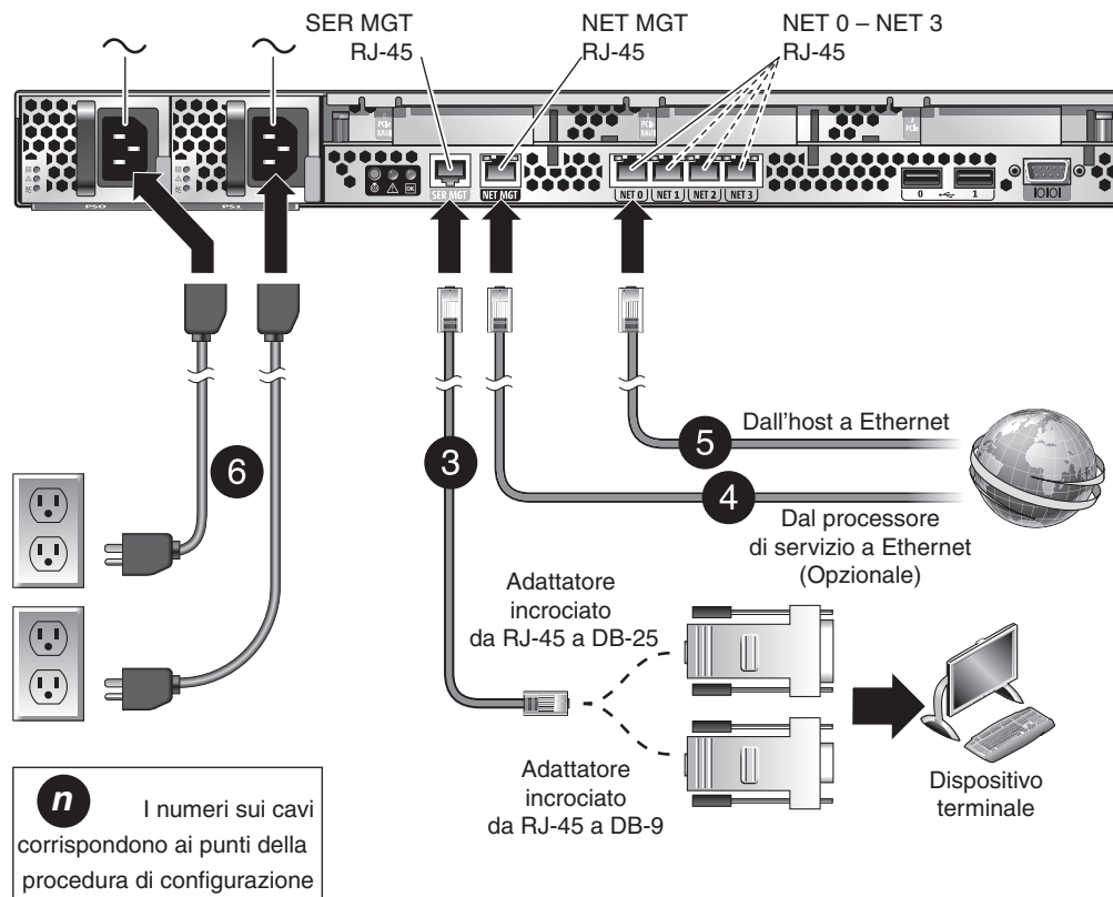
FIGURA 2 Connessioni del server
