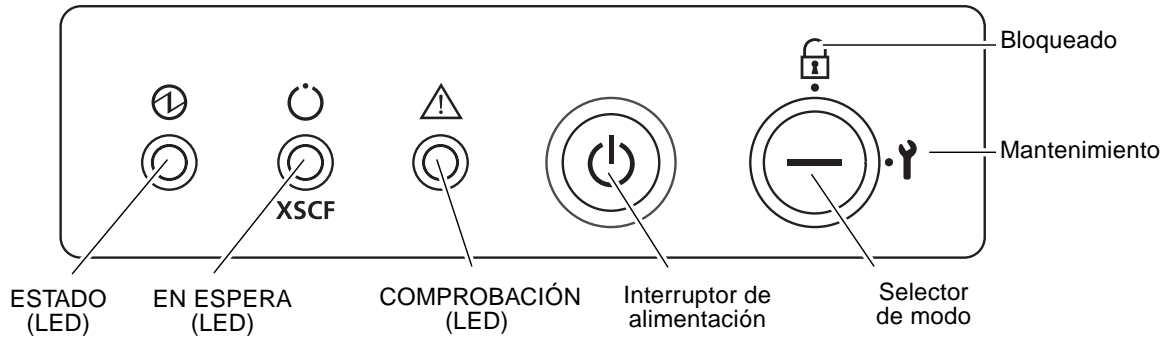
FIGURA 1-10 Panel del operador
