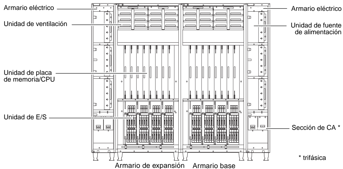
FIGURA 1-9 Vista posterior del servidor M9000 (con un armario de expansión) y el armario eléctrico
