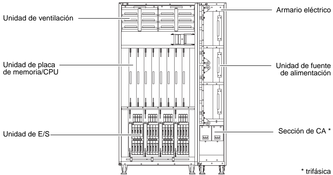
FIGURA 1-7 Vista posterior del servidor M9000 (armario base sólo) y armario eléctrico
