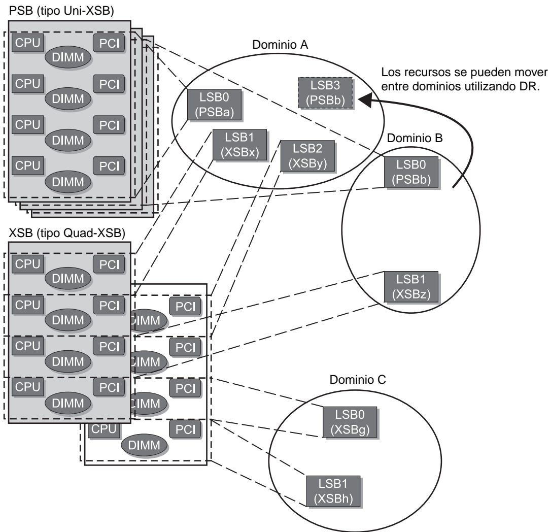
FIGURA 2-4 Configuración de dominio
