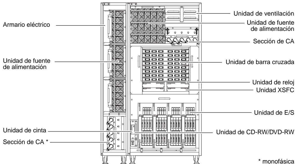
FIGURA 1-6 Vista frontal del servidor M9000 (armario base sólo) y el armario eléctrico
