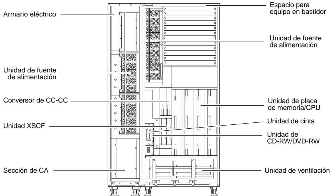
FIGURA 1-4 Vista frontal del servidor M8000 y el armario eléctrico
