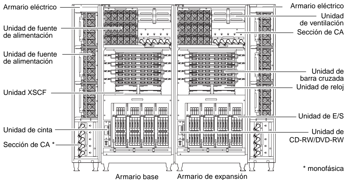
FIGURA 1-8 Vista frontal del servidor M9000 (con un armario de expansión) y el armario eléctrico
