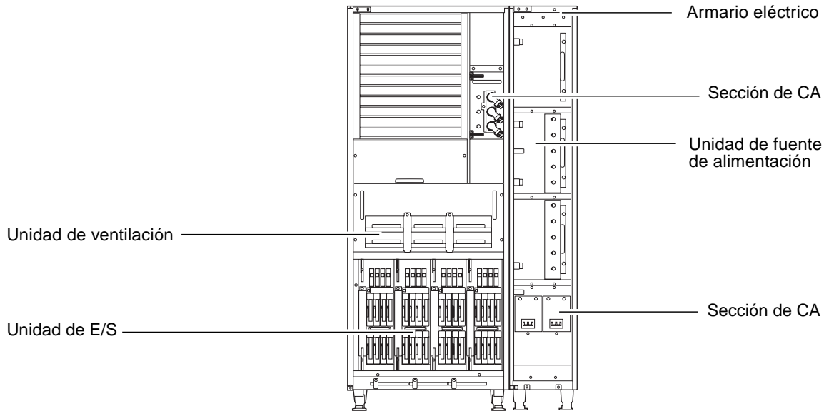
FIGURA 1-5 Vista posterior del servidor M8000 y el armario eléctrico
