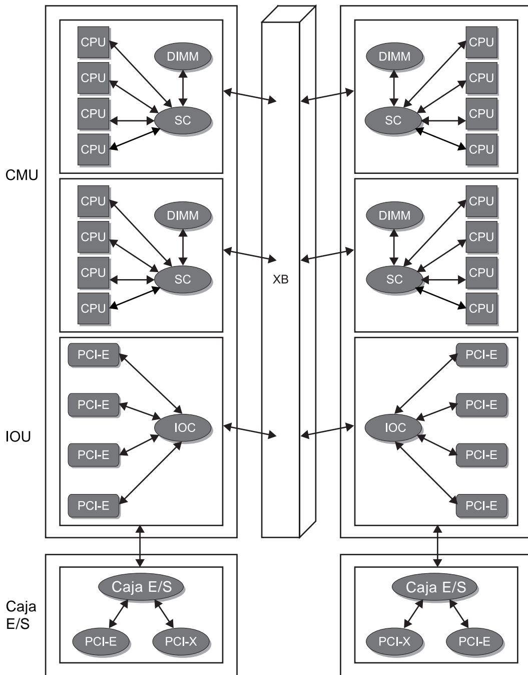
FIGURA 2-2 Conexiones de los componentes principales
