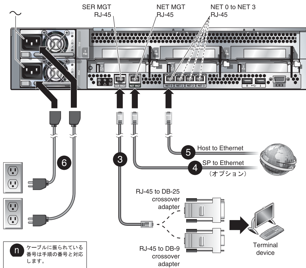
図 2 サーバの接続
