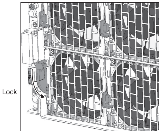
図 14-9 FANUの固定
