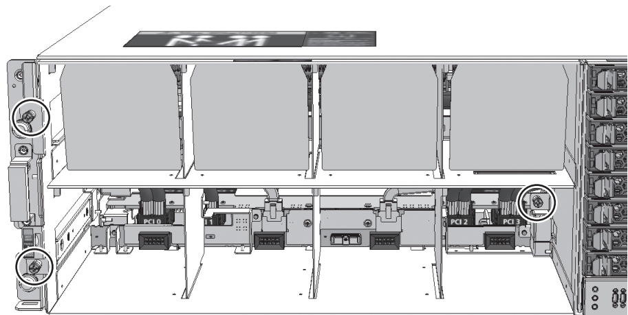
図 18-29 FANBPUの固定
