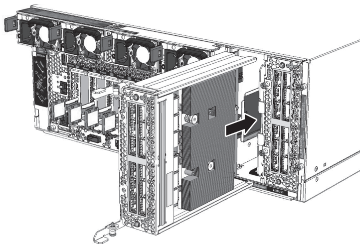
図 20-7 XBUの挿入
