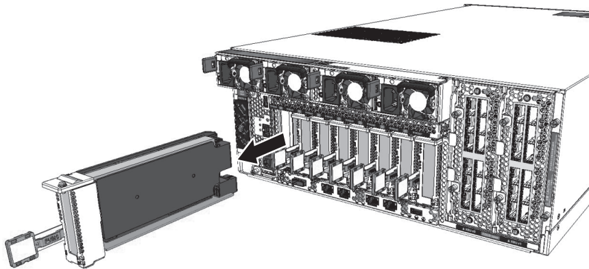
図 18-3 PCICSの取り外し
