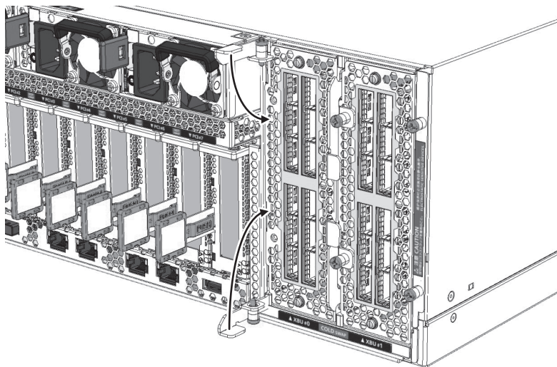
図 20-8 XBUの接続
