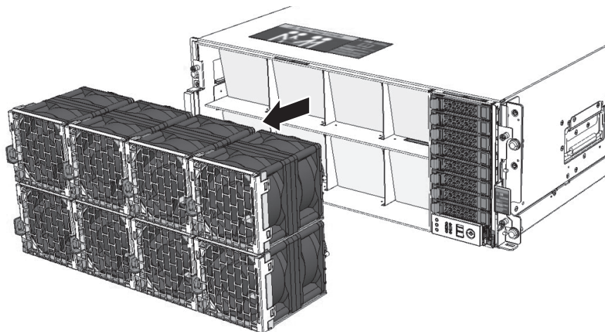
図 16-2 FANUの取り外し
