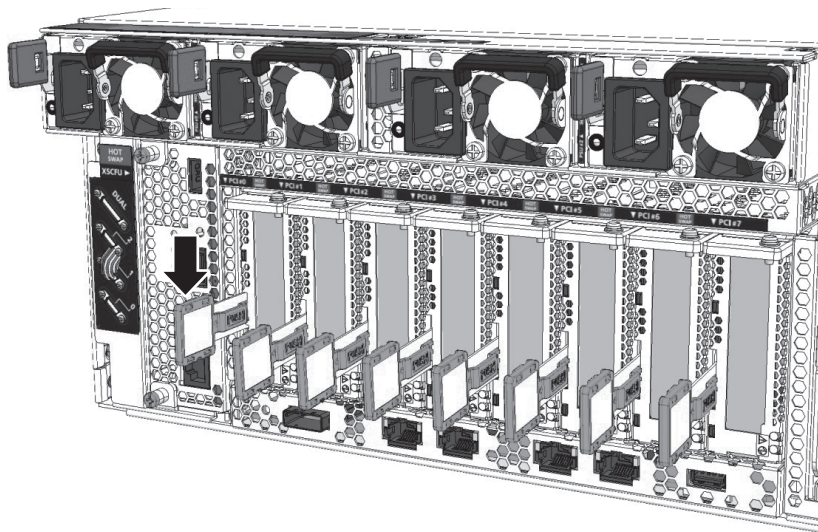
図 12-13 PCICSの固定
