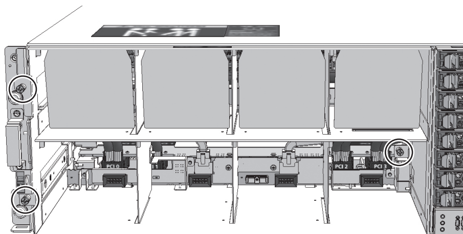
図 16-15 FANBPUの固定
