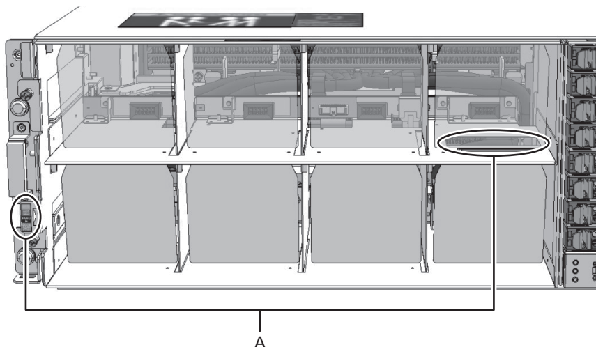
図 14-5 FANBPUの取り外し
