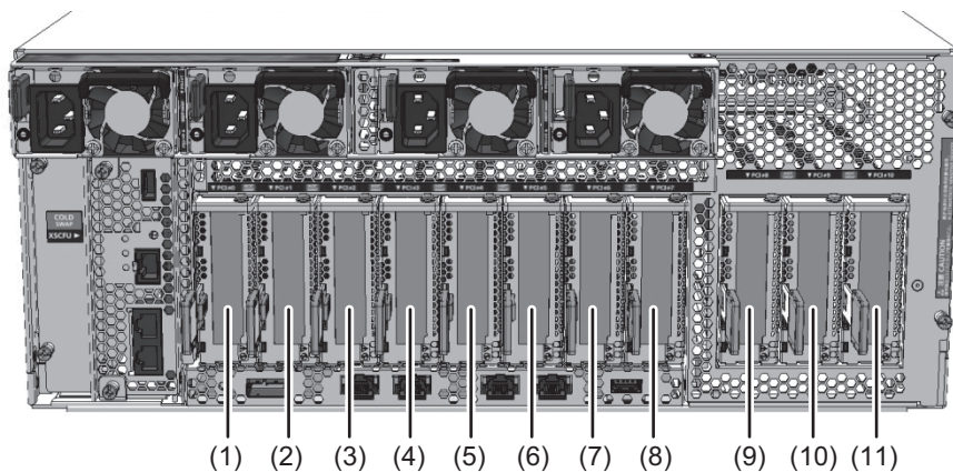
図 12-1 SPARC M12のPCIeカード搭載位置
