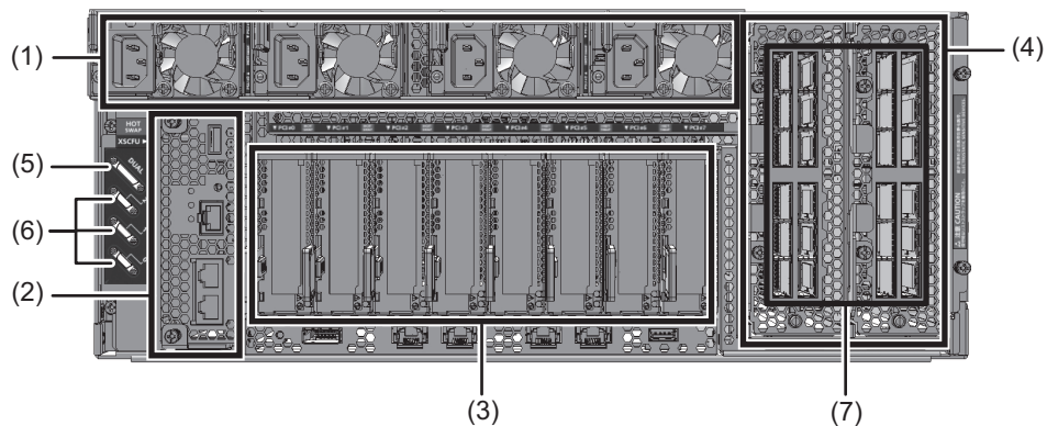
図 2-2 背面からアクセス可能なユニット
