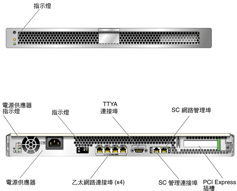
圖 3 SPARC Enterprise T1000 伺服器前方與後方面板
