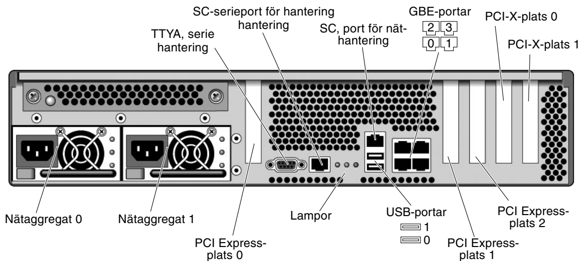
FIGUR 4 Bakpanelen på SPARC Enterprise T2000
