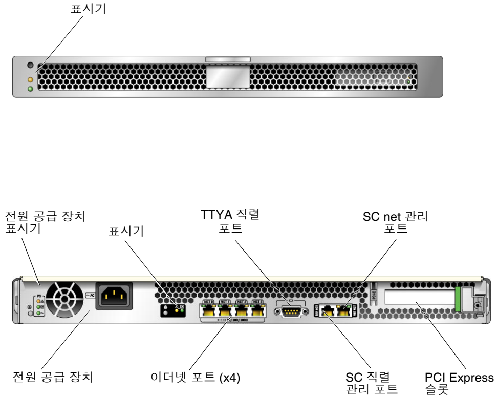
그림 3 SPARC Enterprise T1000 서버 전면 및 후면 패널
