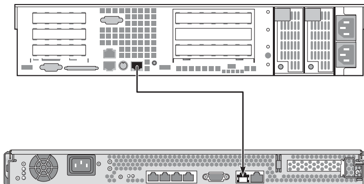
그림 1-4 서버와 다른 시스템 간 TIP 연결
