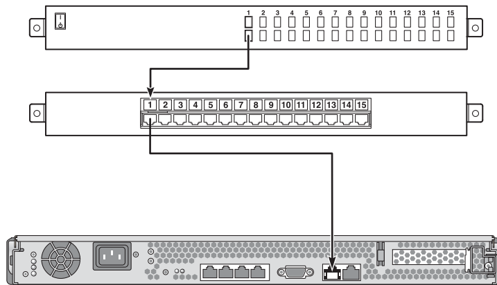
그림 1-3 터미널 서버와 사용 중인 서버 간의 패치 패널 연결
