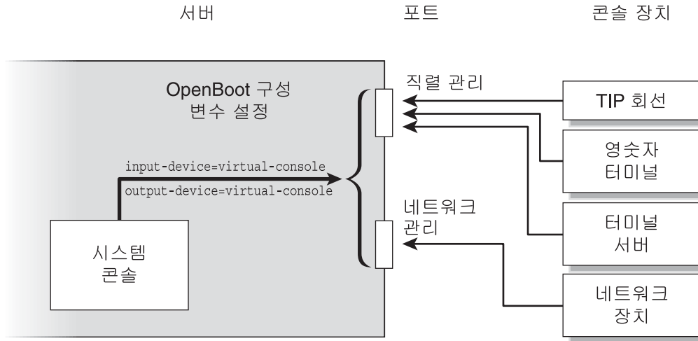
그림 1-1 시스템 콘솔 지정
