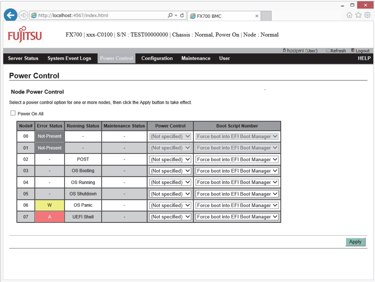
図 3.6 [Power Control] 画面
