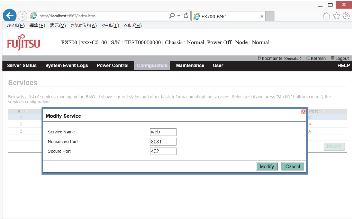
図 3.9 webサービス変更ダイアログボックス
