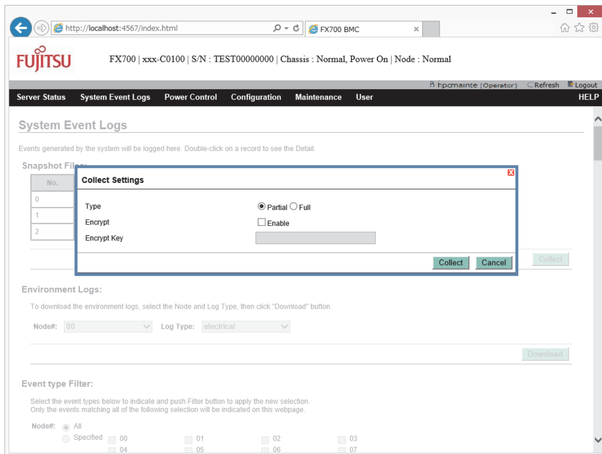
図 3.4 snapshot採取ダイアログ
