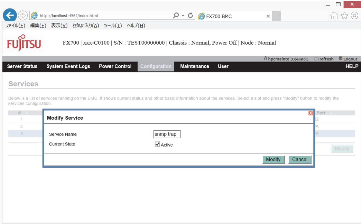
図 3.11 snmpサービス変更ダイアログボックス
